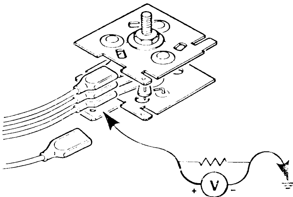
FIG. 7. RECTIFIER DC OUTPUT TEST
