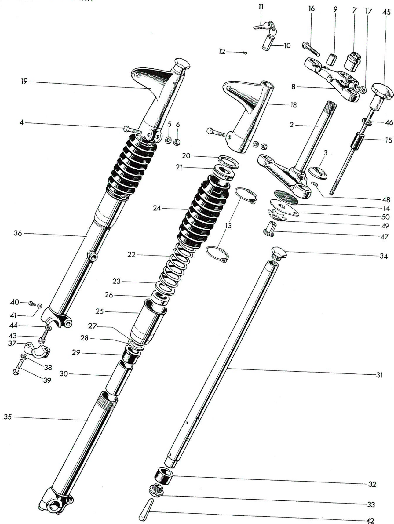
Fig. 17. TELESCOPIC FRONT FORK
