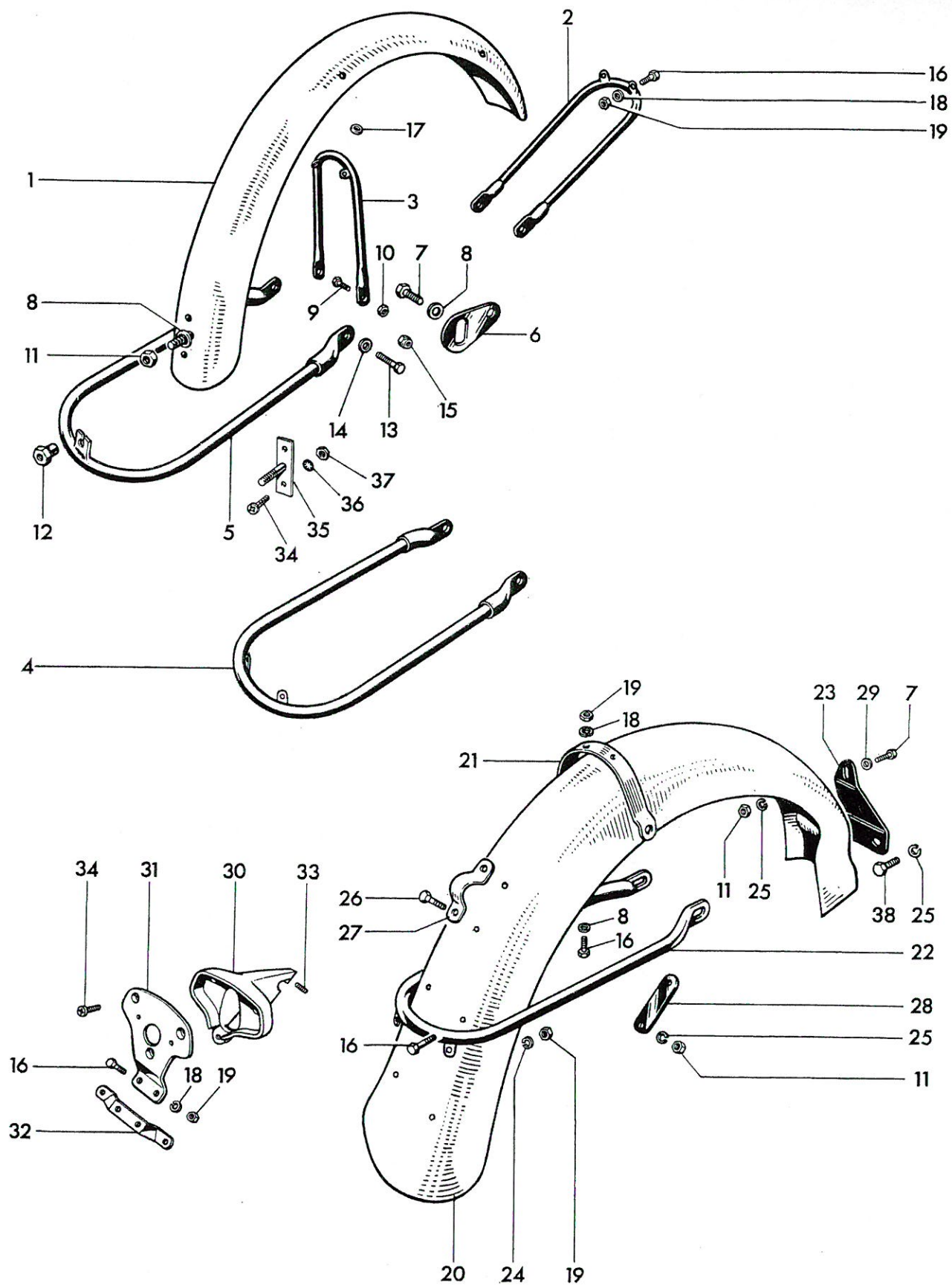
Fig. 26. MUDGUARDS (FENDERS U.S.A.)
