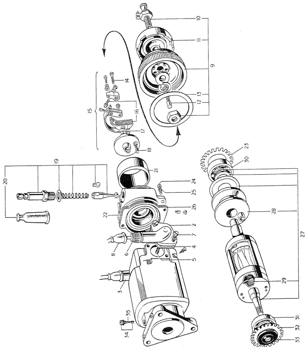
FIG. 32. LUCAS MAGNETO
