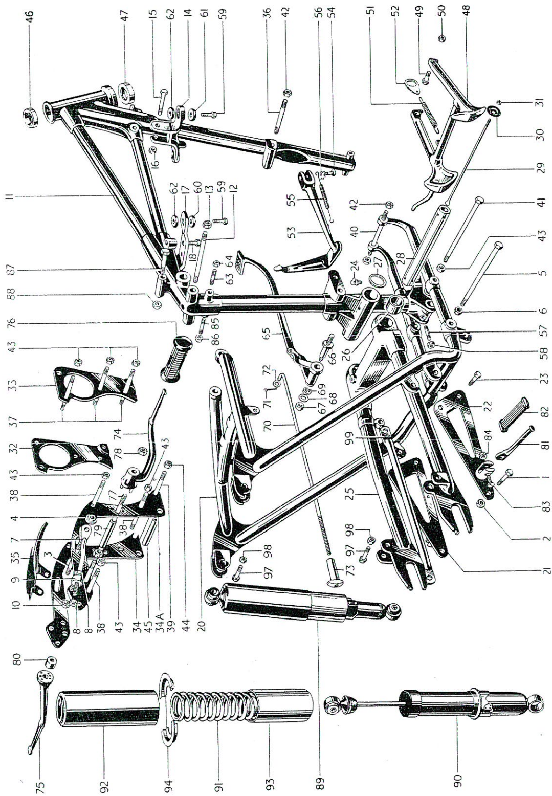
FIG. 13. FRAME
