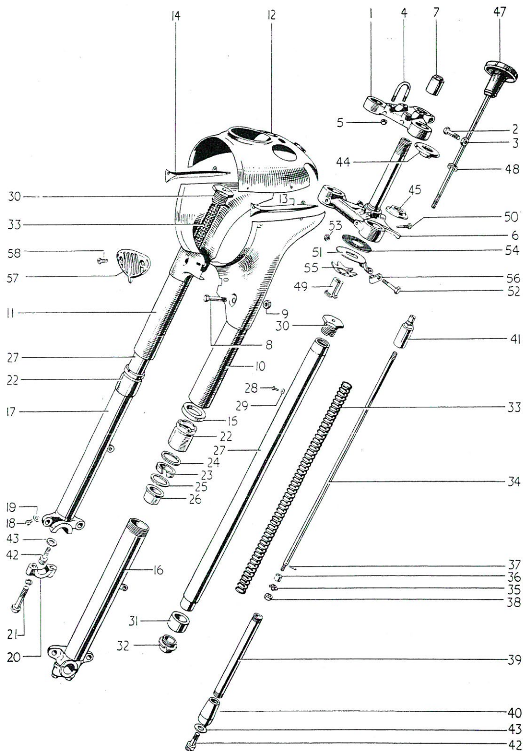
FIG. 15. TELESCOPIC FORK
