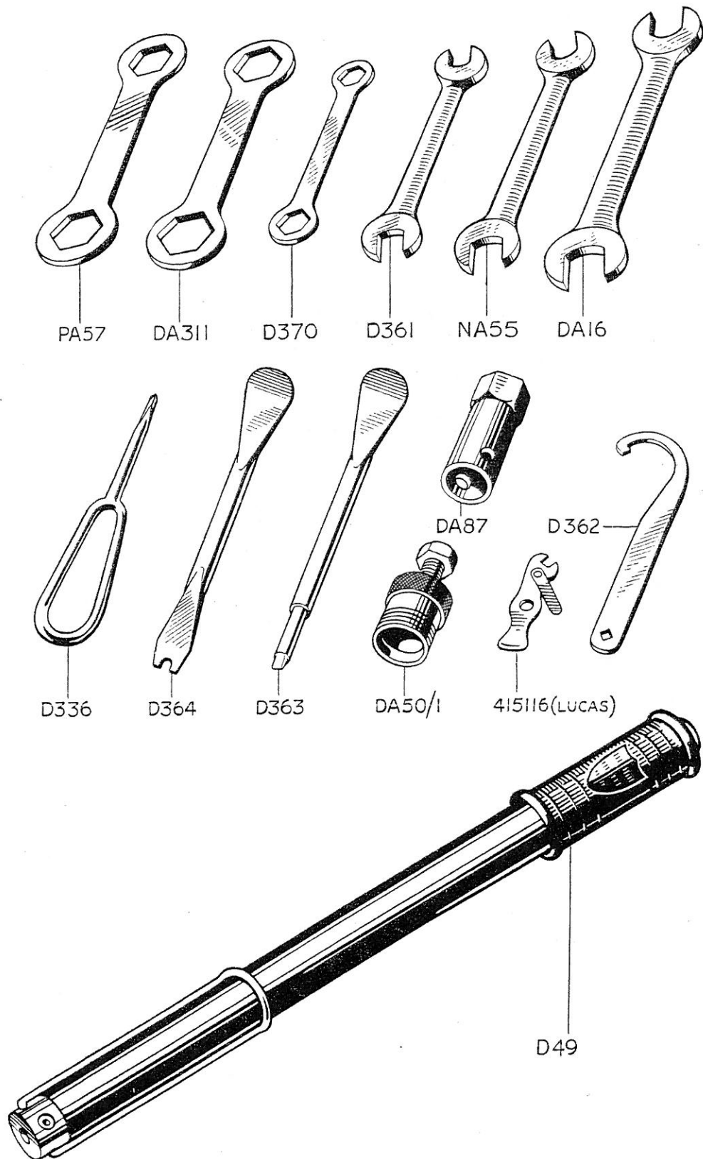
FIG. 27. TOOL KIT
