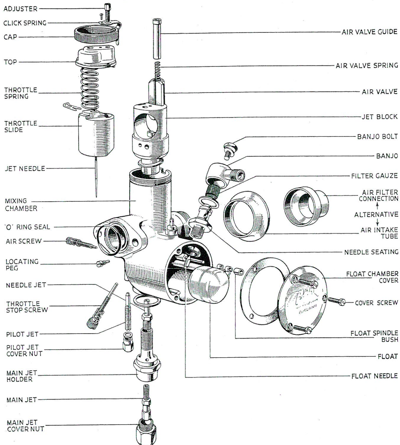
FIG. 29. AMAL CARBURETTER
