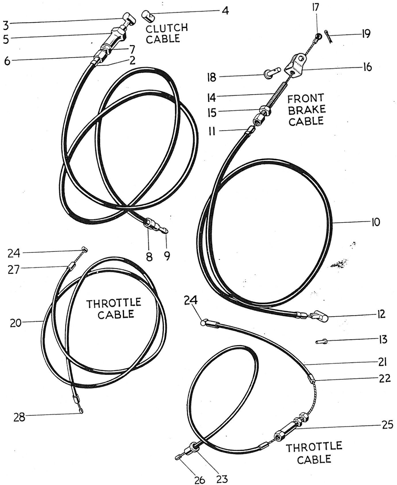
Fig. 20. CONTROL CABLES
