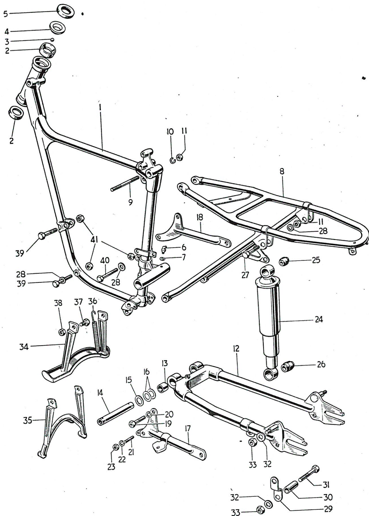
Fig. 7. FRAME COMPLETE
