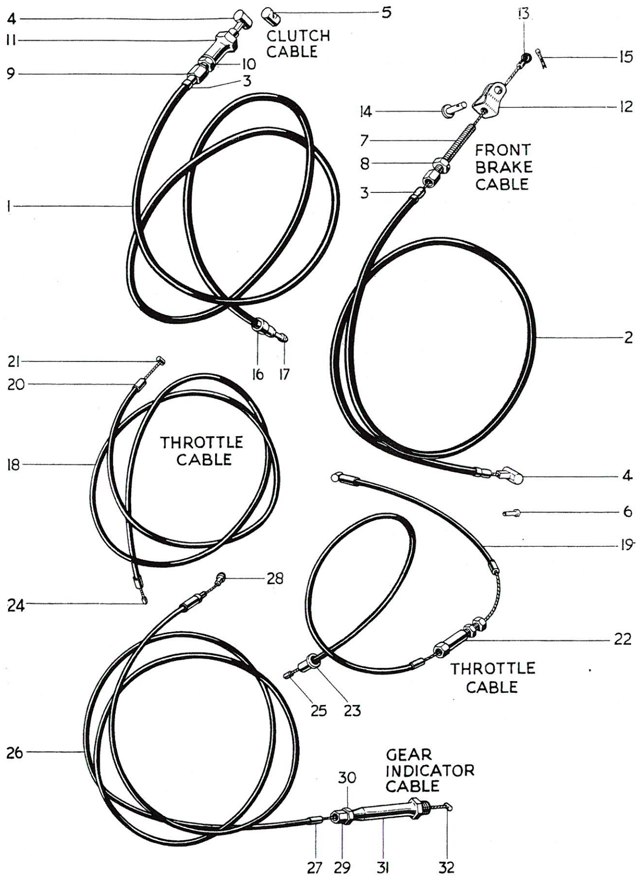
Fig. 23. CONTROL CABLES.
