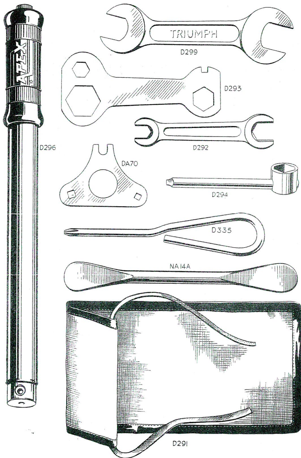
FIG. 12. TOOLS.
