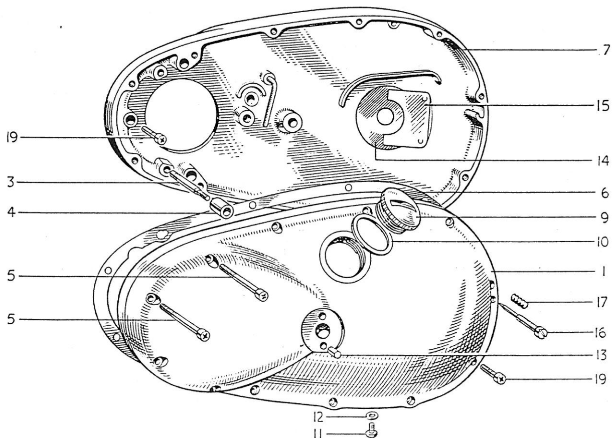
FIG. 24. PRIMARY CHAINCASE
