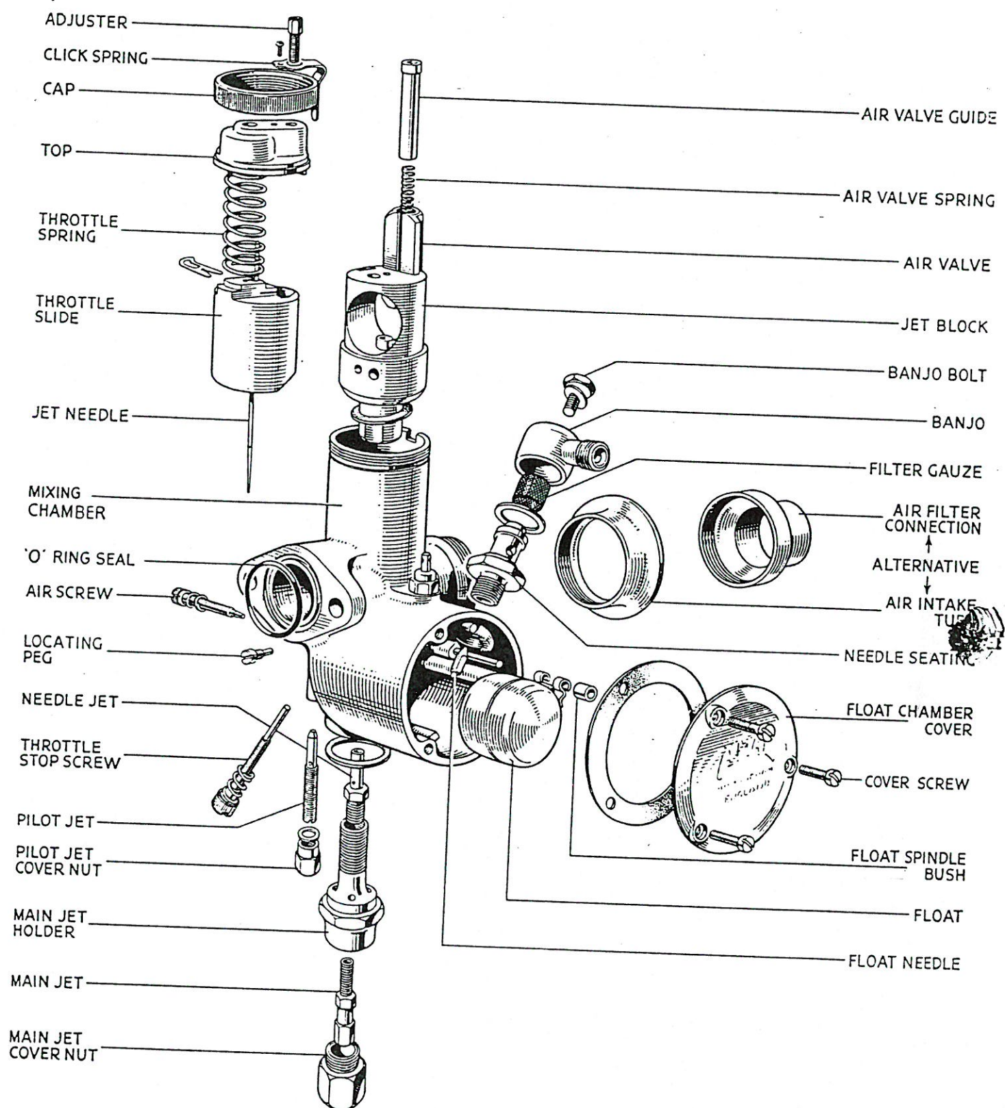
FIG. 29. AMAL CARBURETTER
