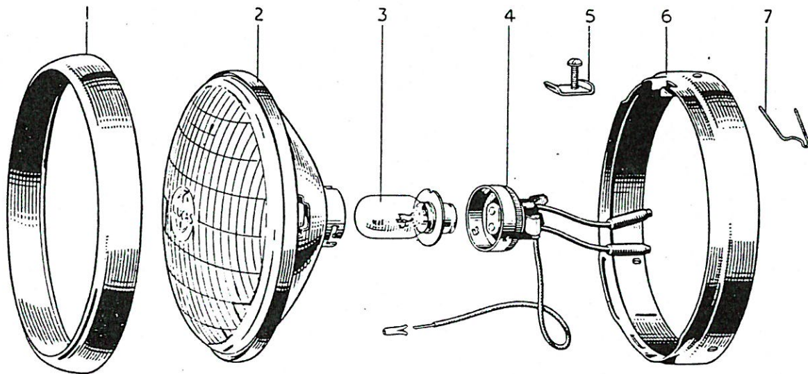
FIG. 31. HEAD LAMP
