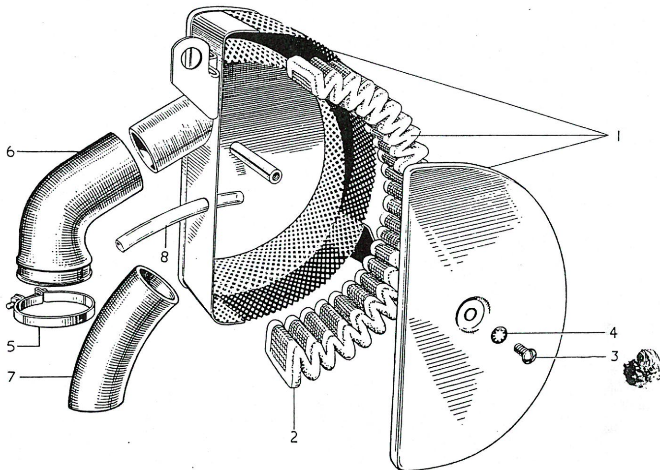
FIG. 28. AIR FILTER
