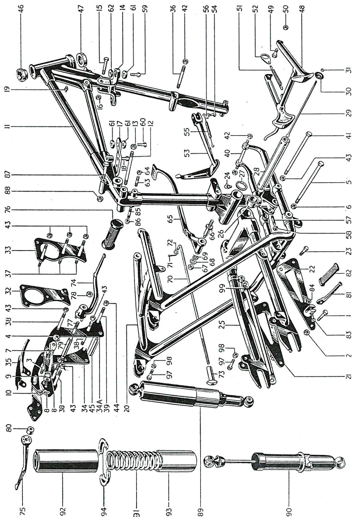
FIG. 13. FRAME
