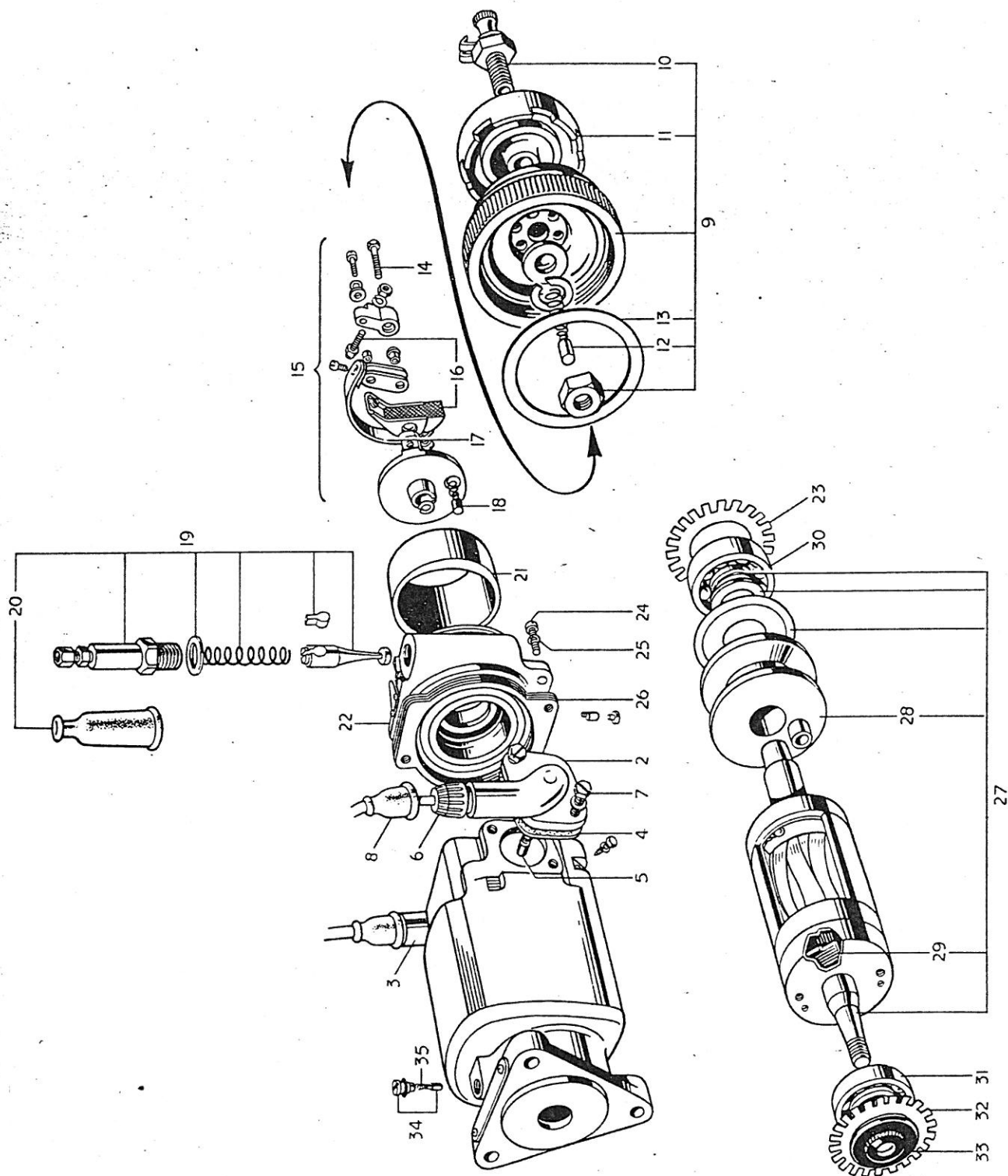
FIG. 34. LUCAS MAGNETO
