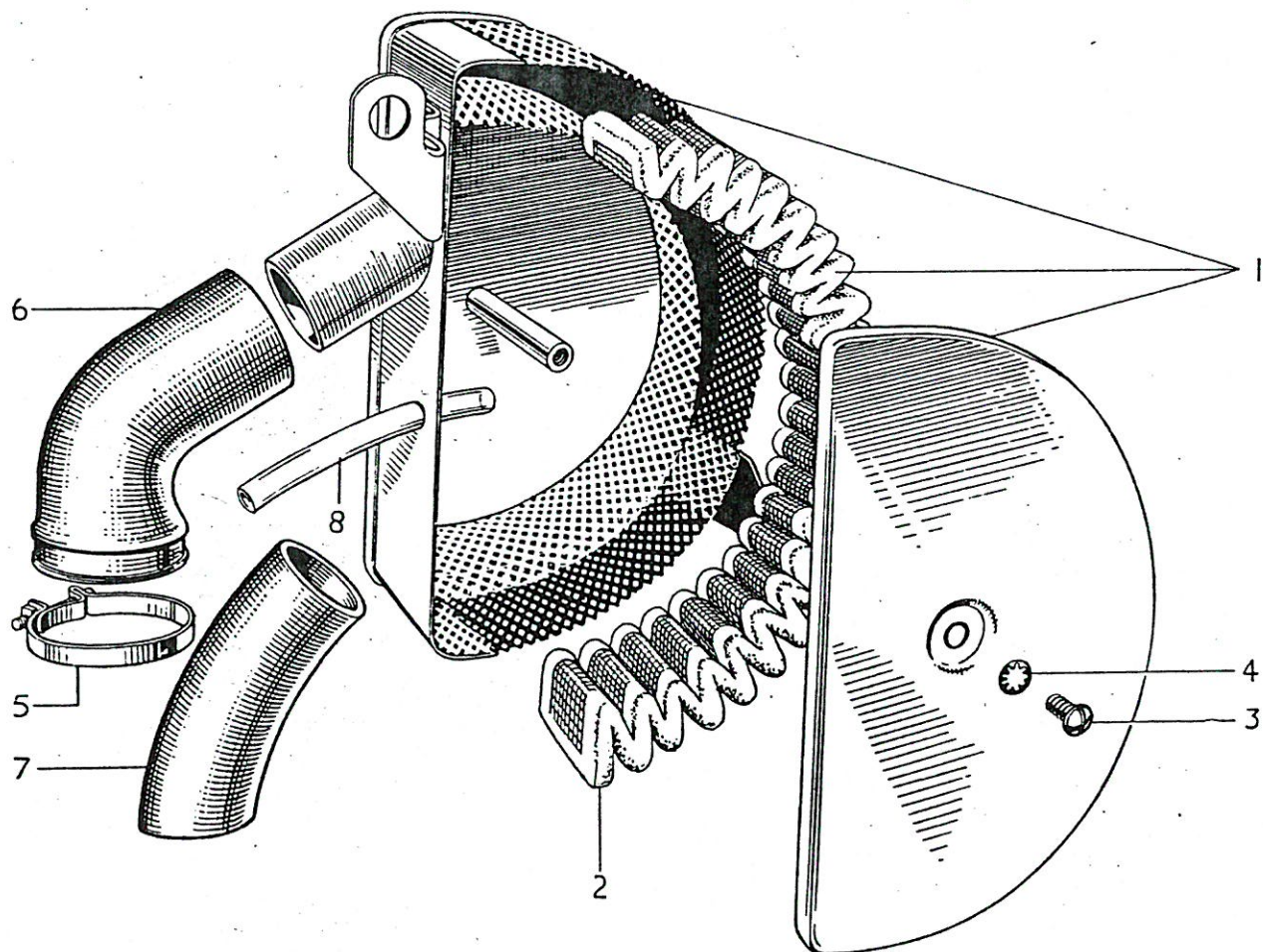
FIG. 29. AIR FILTER
