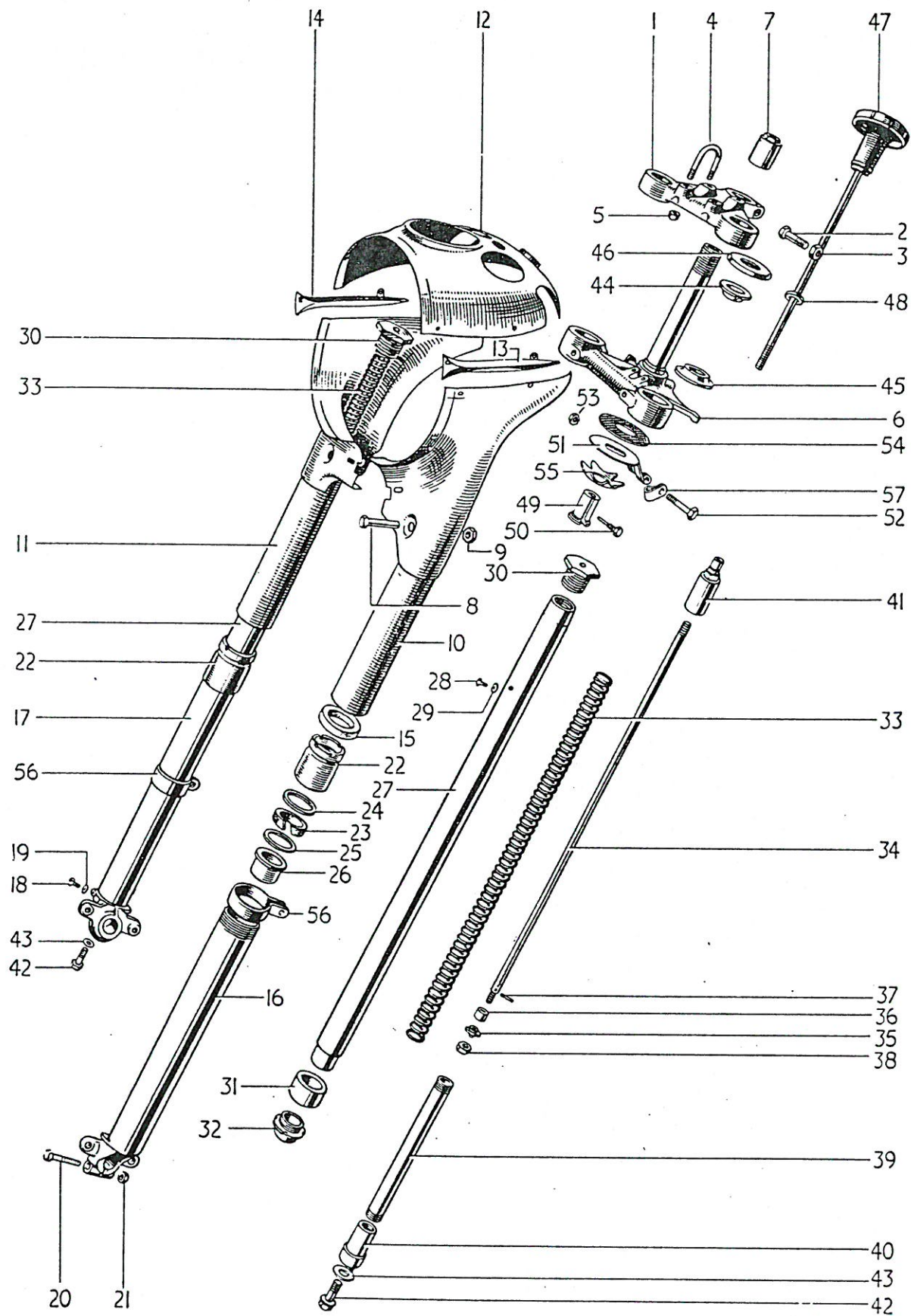
FIG. 16. TELESCOPIC FORK
