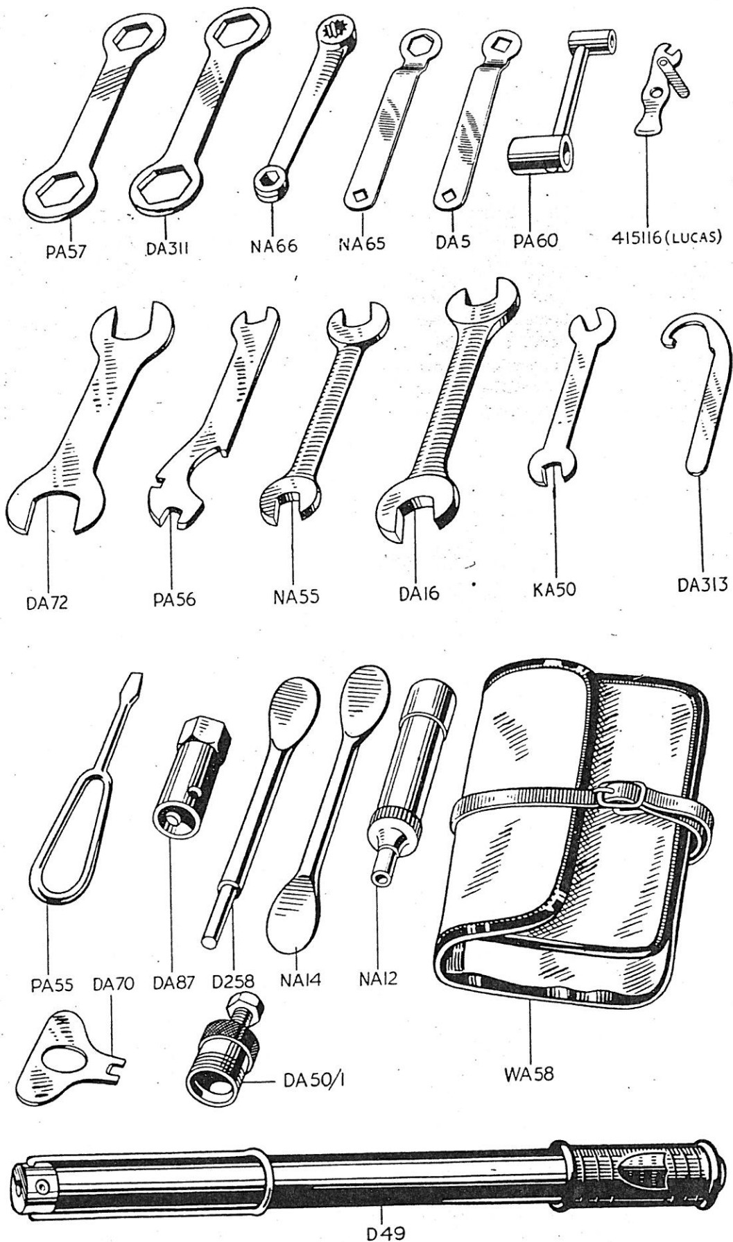
FIG. 28. TOOL KIT
