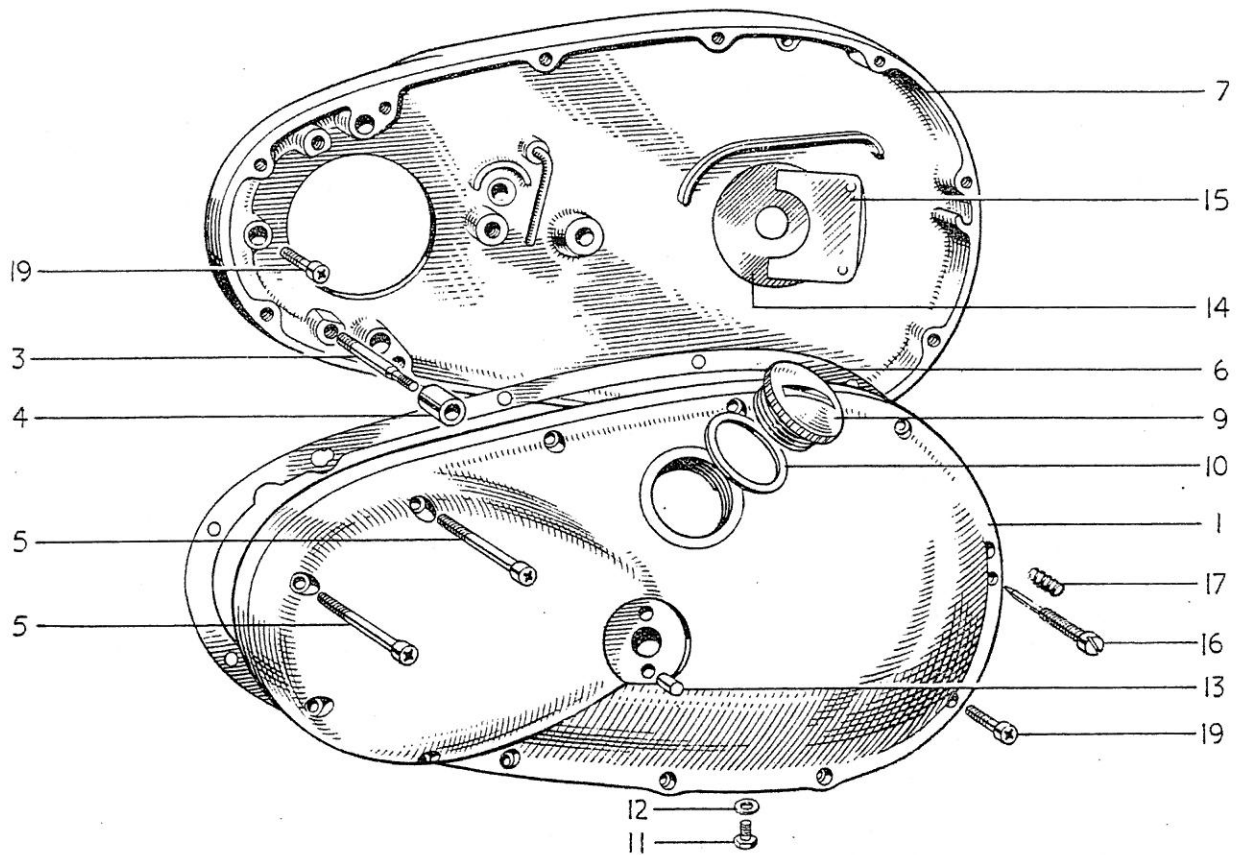
FIG. 24. PRIMARY CHAINCASE
