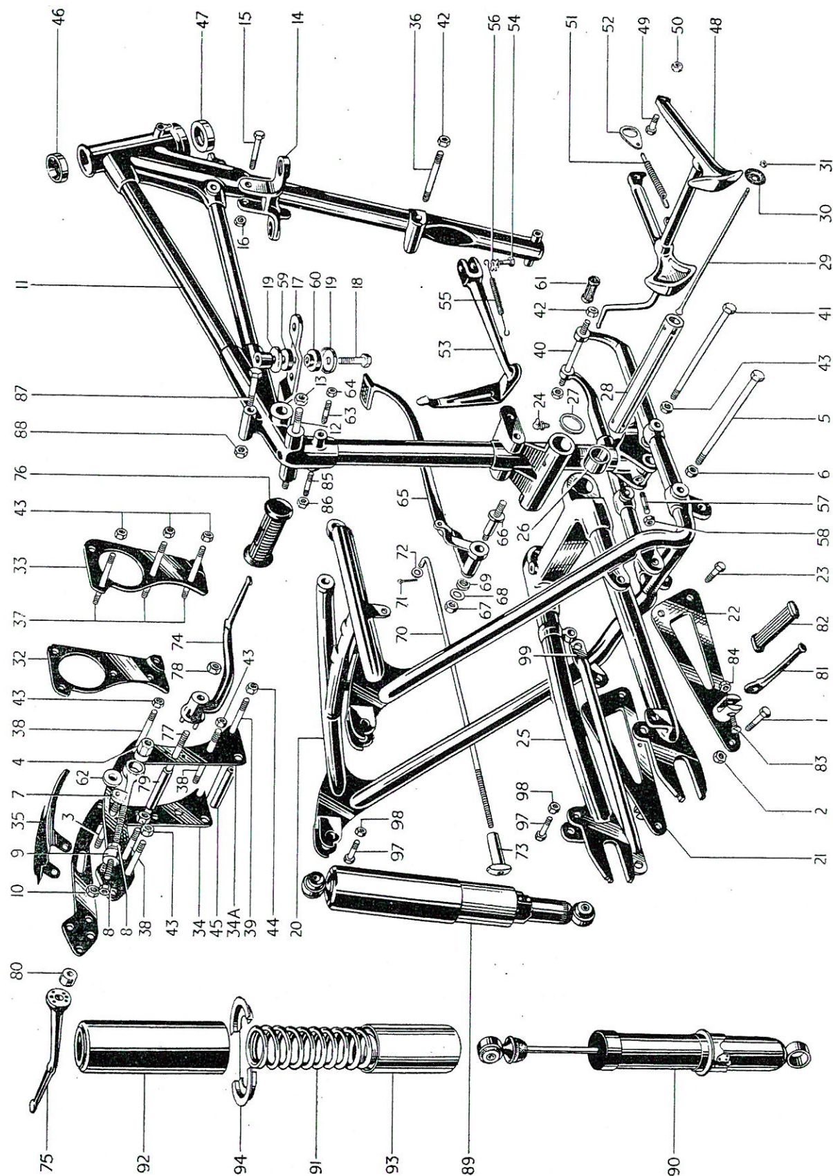
FIG. 13. FRAME
