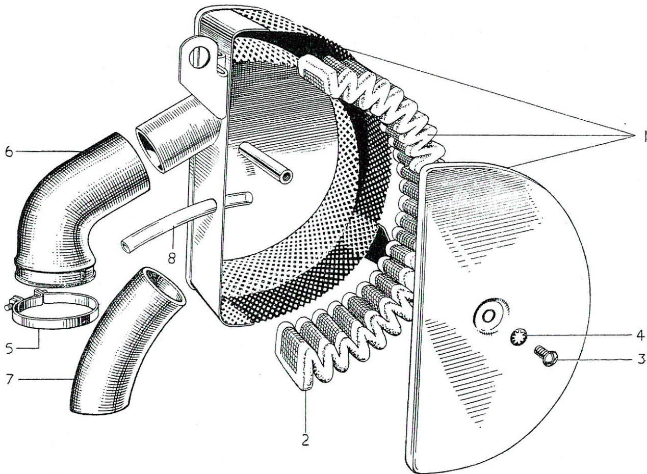
FIG. 28. AIR FILTER
