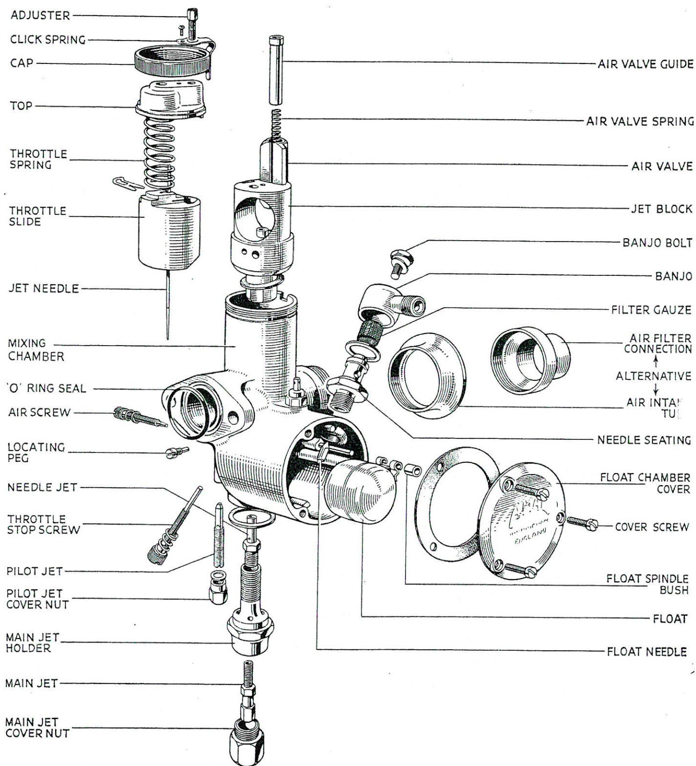
FIG. 29. AMAL CARBURETTER
