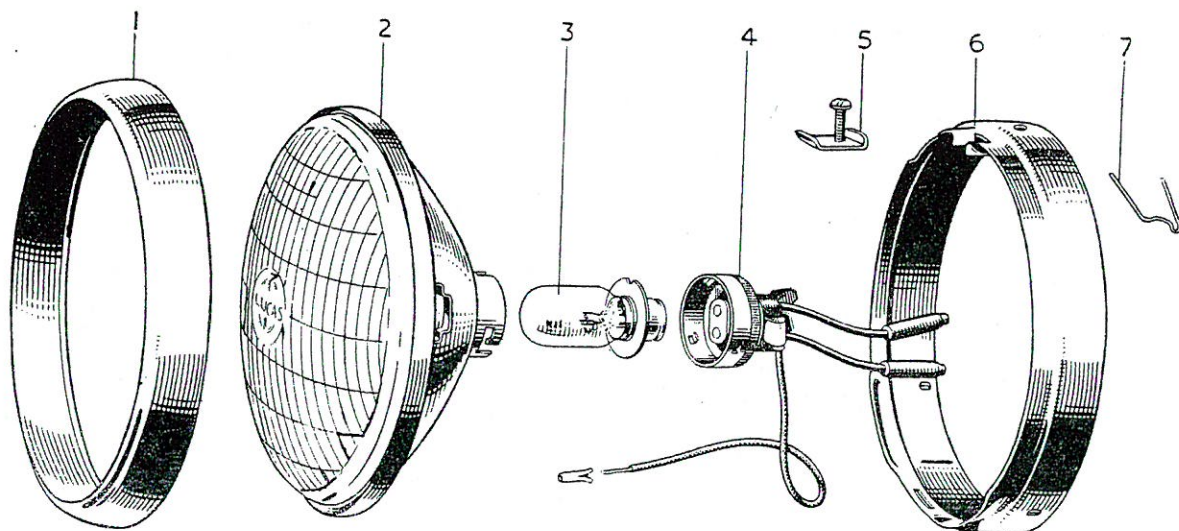
FIG. 31. HEAD LAMP
