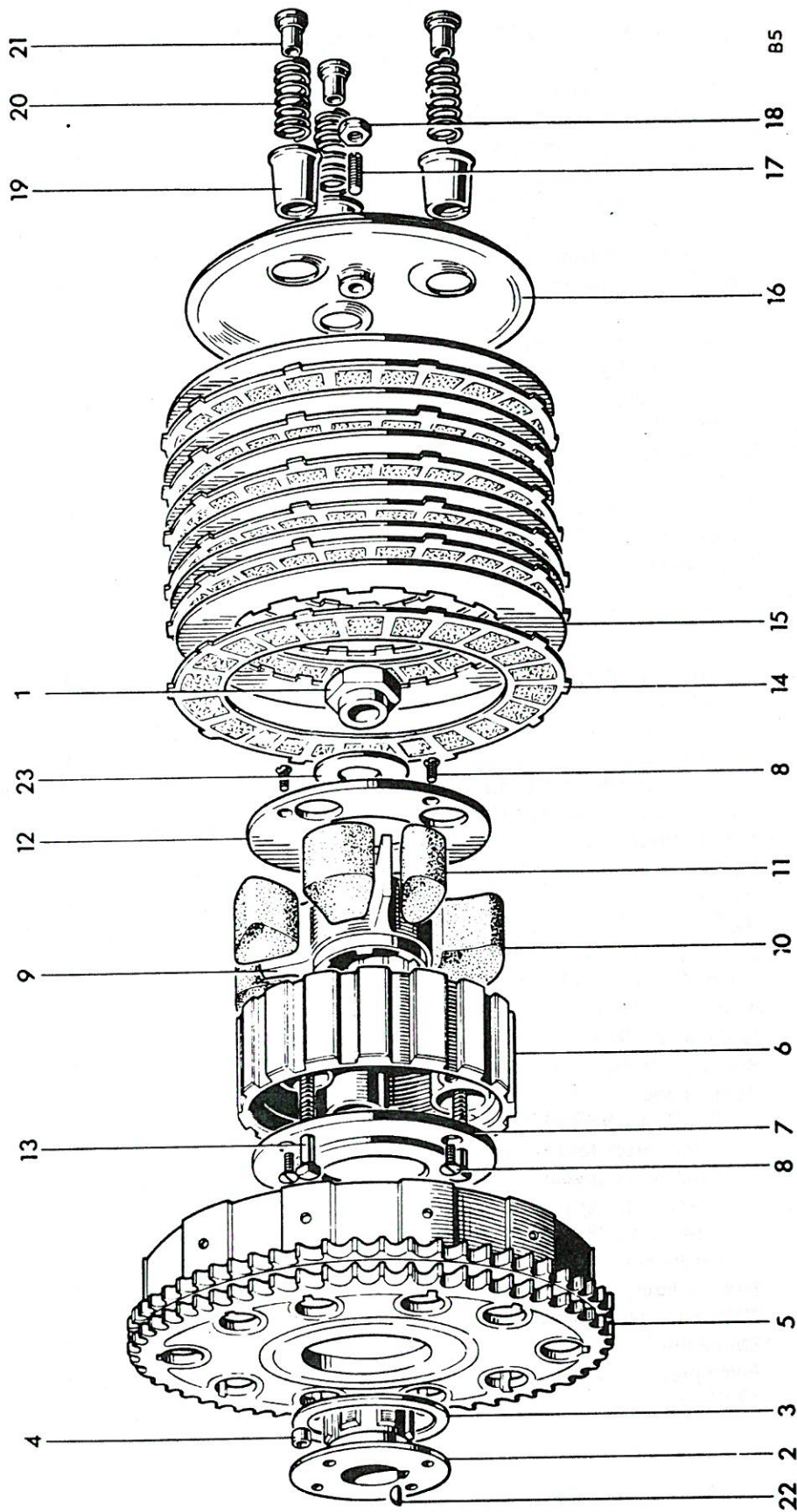
Fig. 10. CLUTCH
