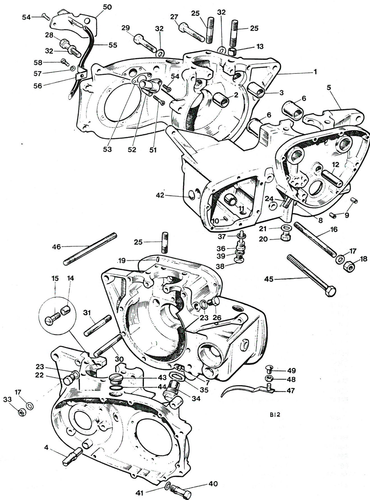
Fig. 2. CRANKCASE
