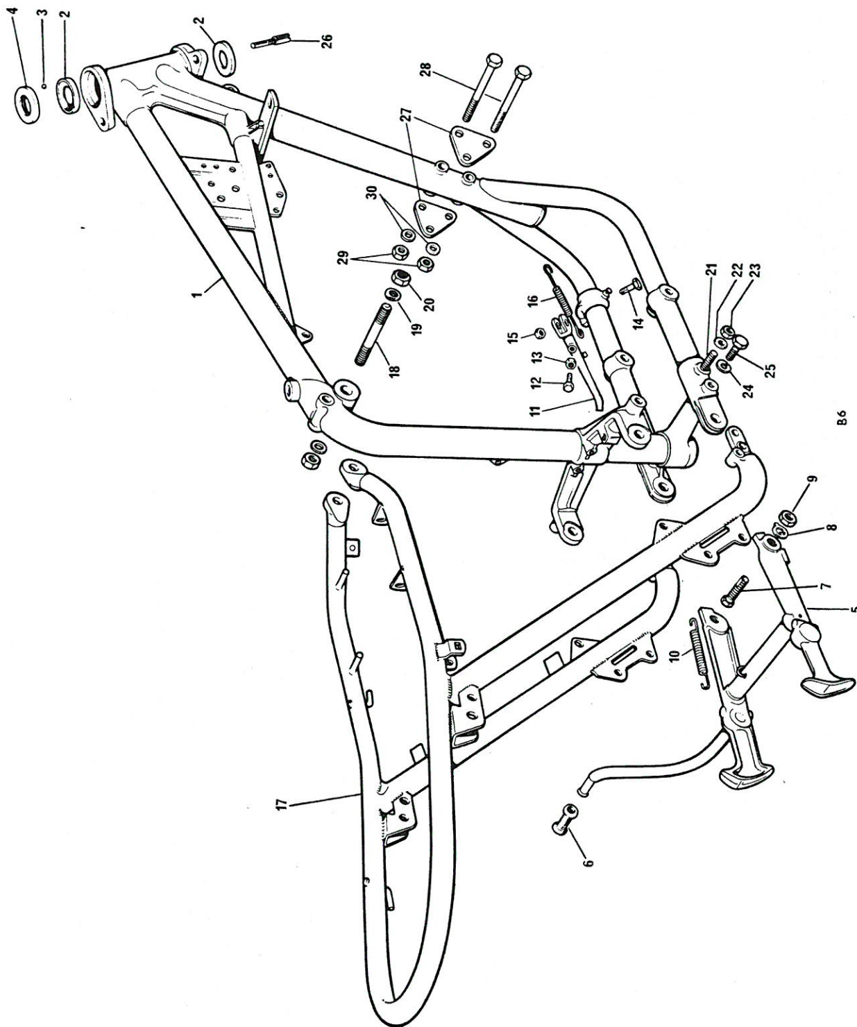
Fig. 12. FRAME
