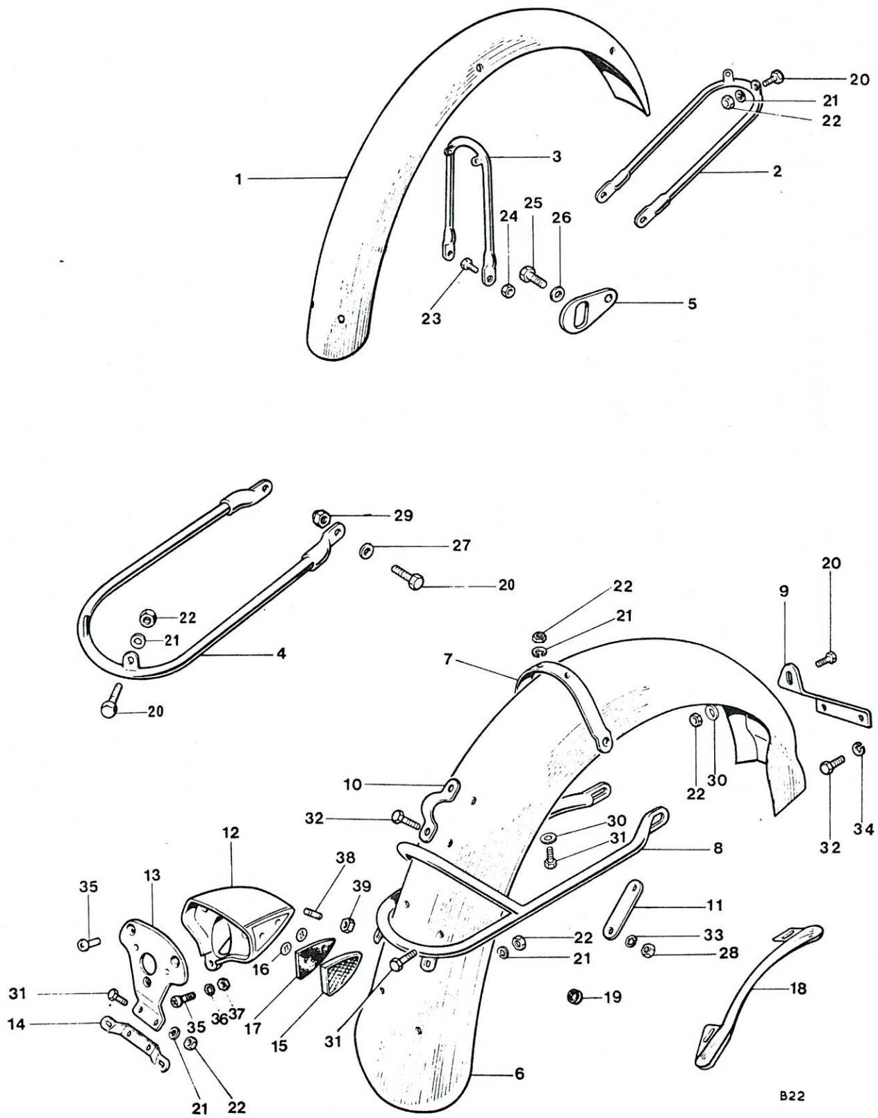
Fig. 25. FENDERS
