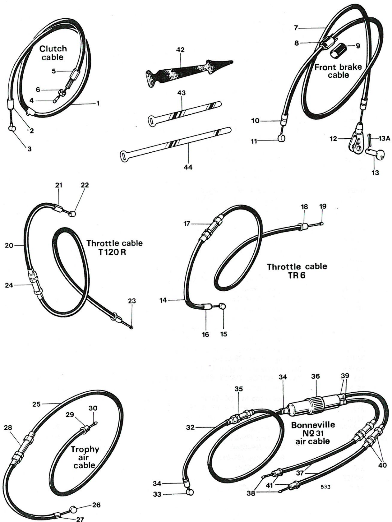
Fig. 27. CONTROL CABLES
