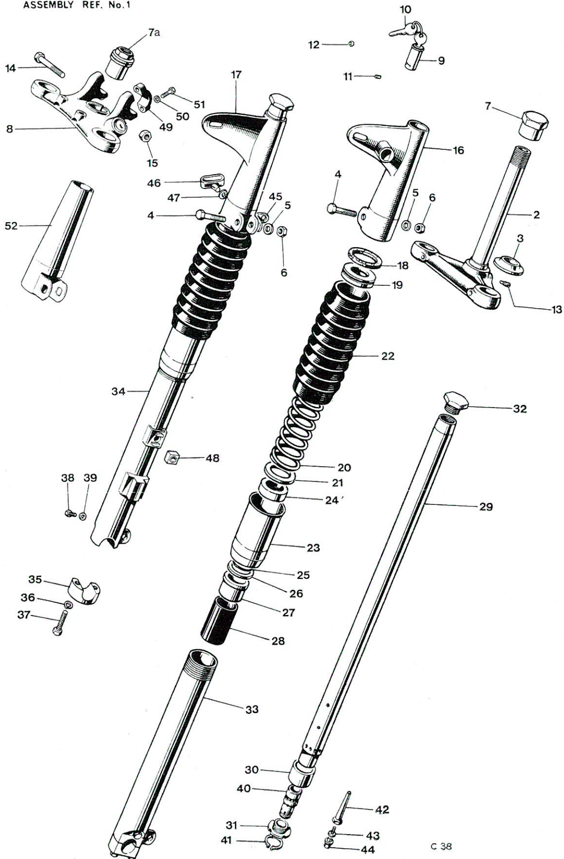
Fig. 17. TELESCOPIC FRONT FORK
