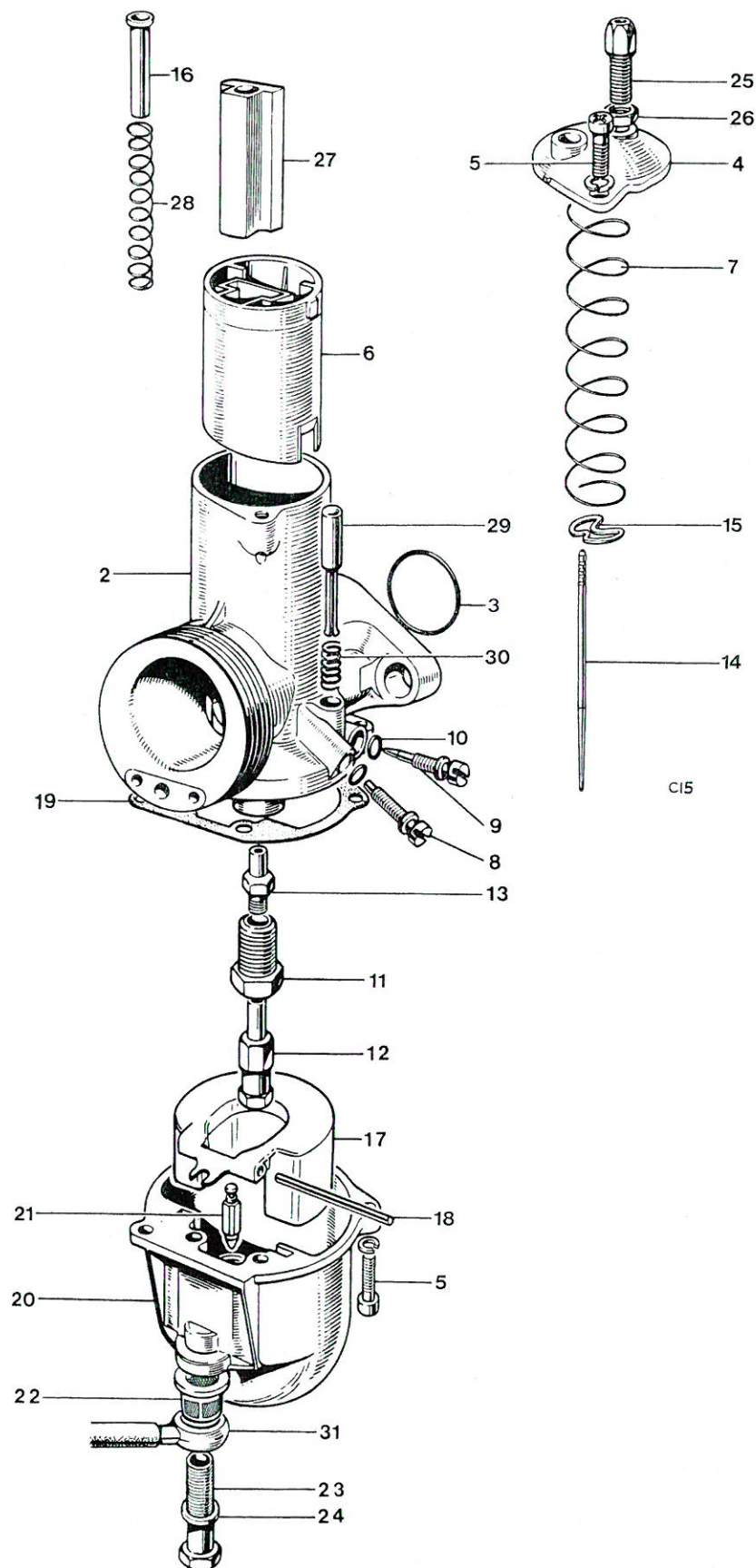
Fig. 31. CARBURETOR T100R
