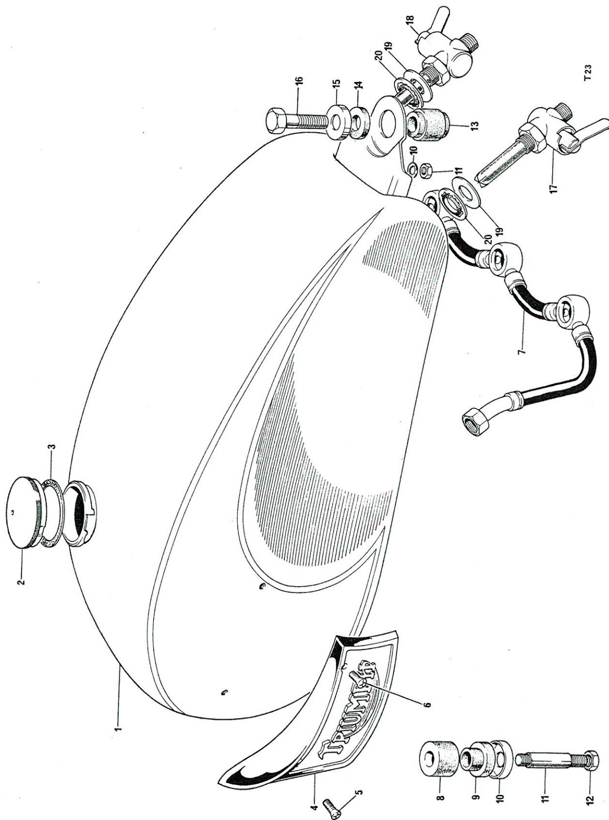
Fig. 24. GAS TANK
