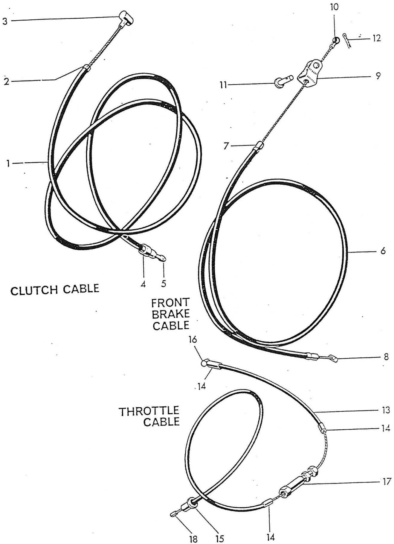
Fig. 17. CONTROL CABLES
