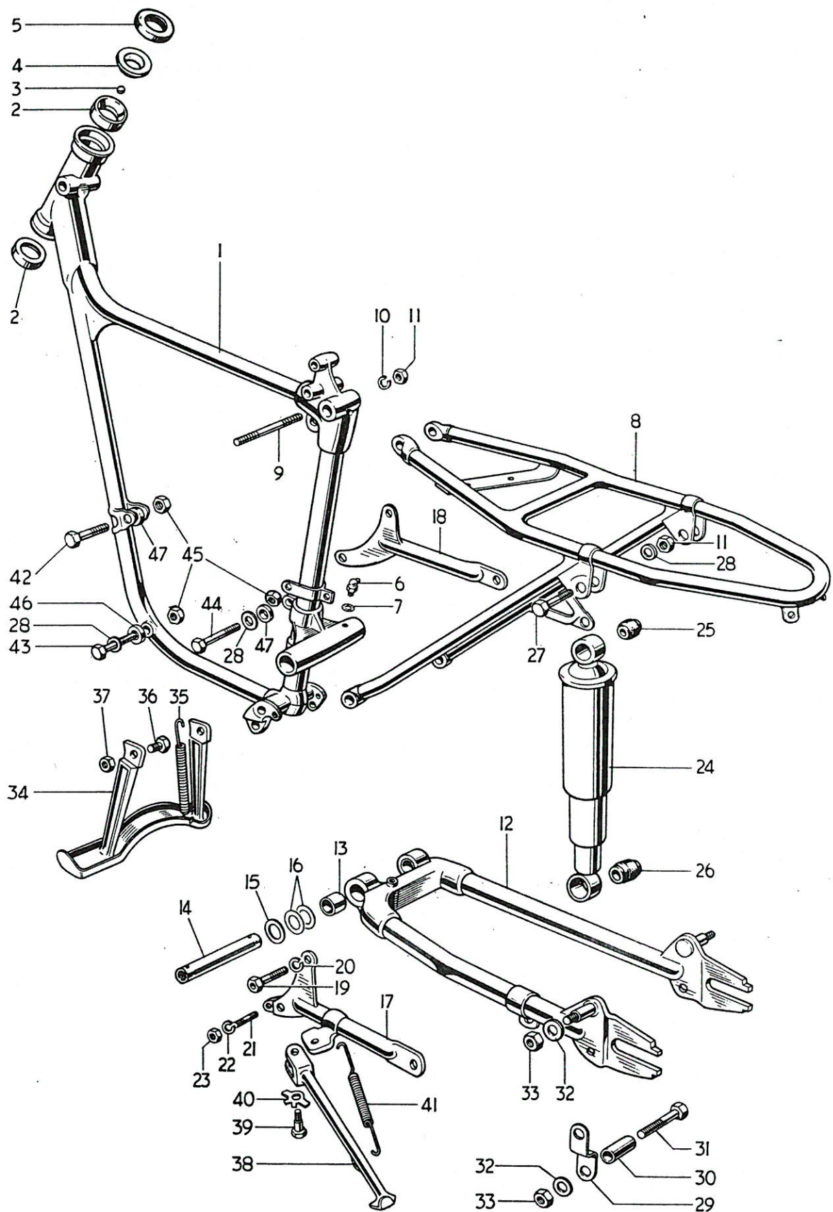
Fig. 8. FRAME COMPLETE
