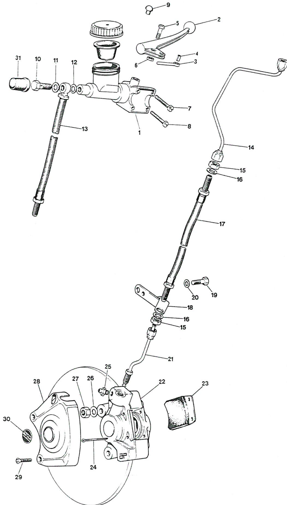
Fig. 23. FRONT BRAKE
