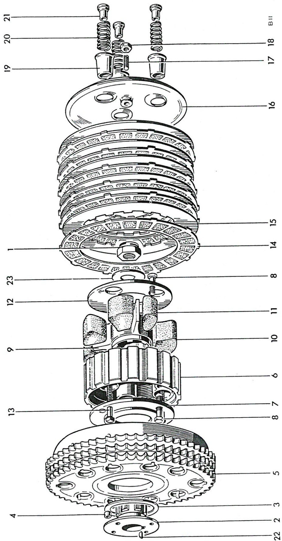
Fig. 14. CLUTCH
