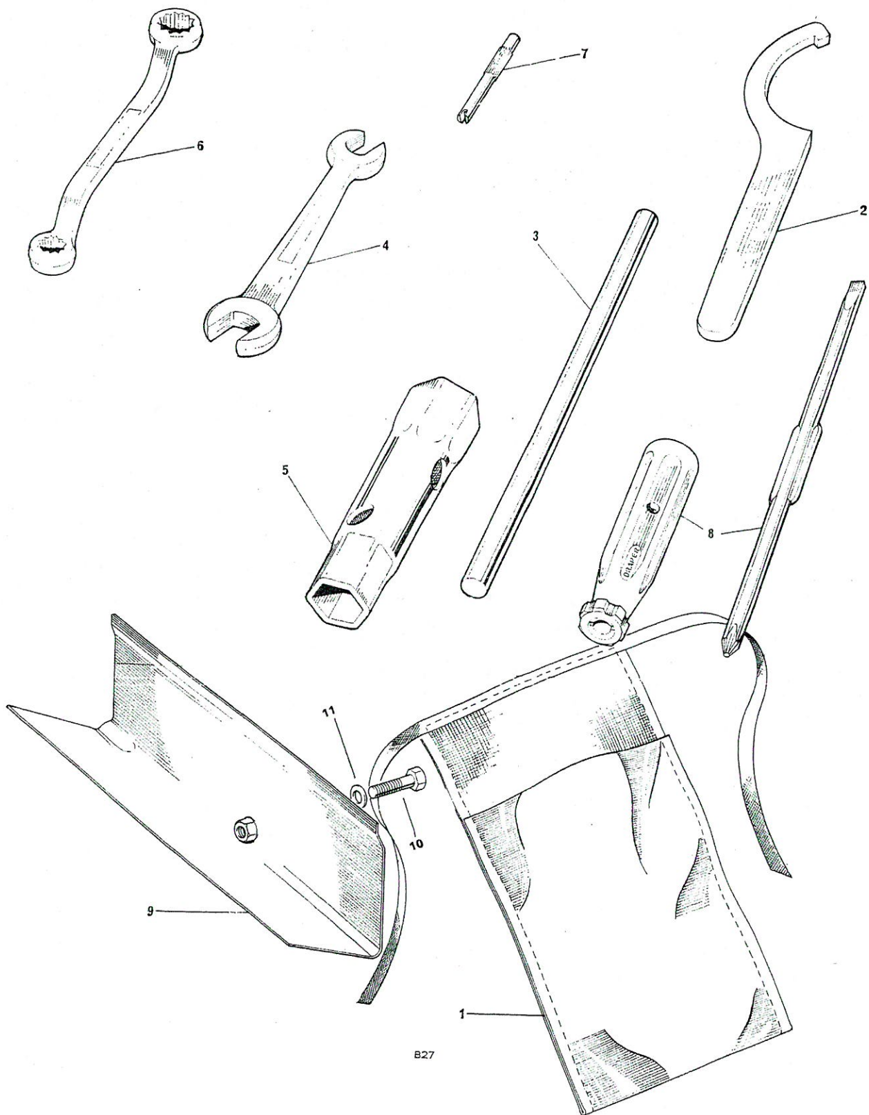
Fig. 31. TOOLKIT
