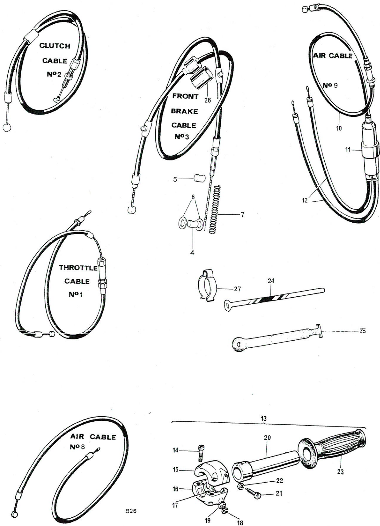
Fig. 30. CONTROL CABLES
