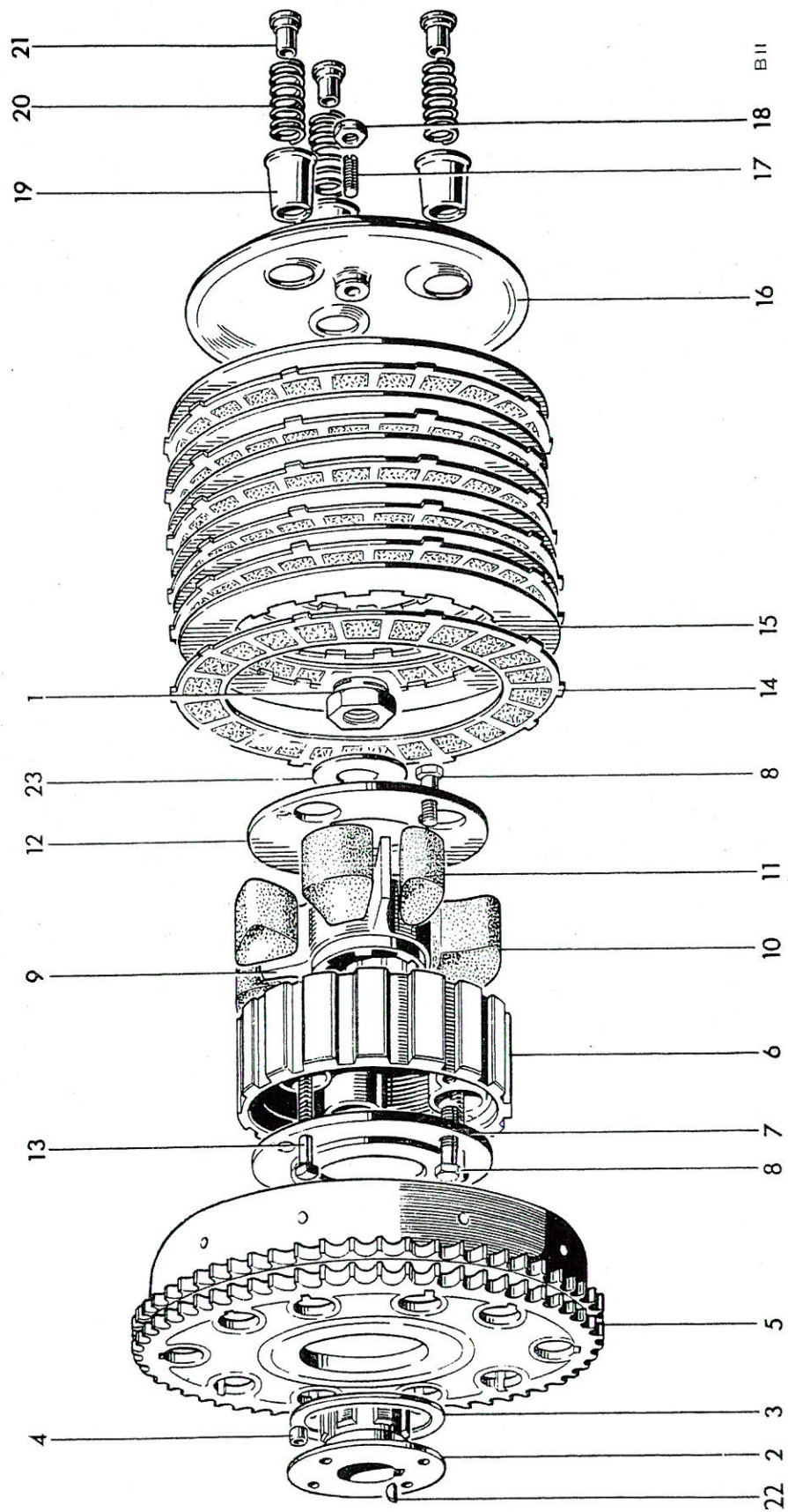
Fig. 15. CLUTCH
