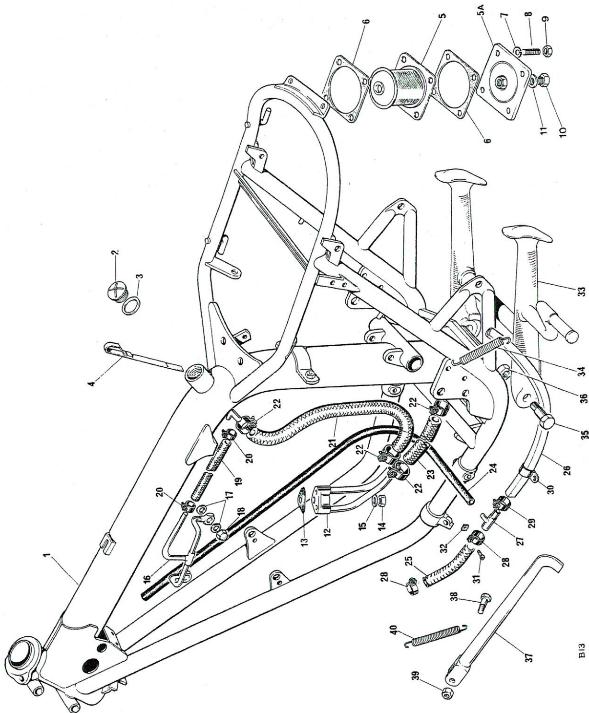
Fig. 17. FRAME
