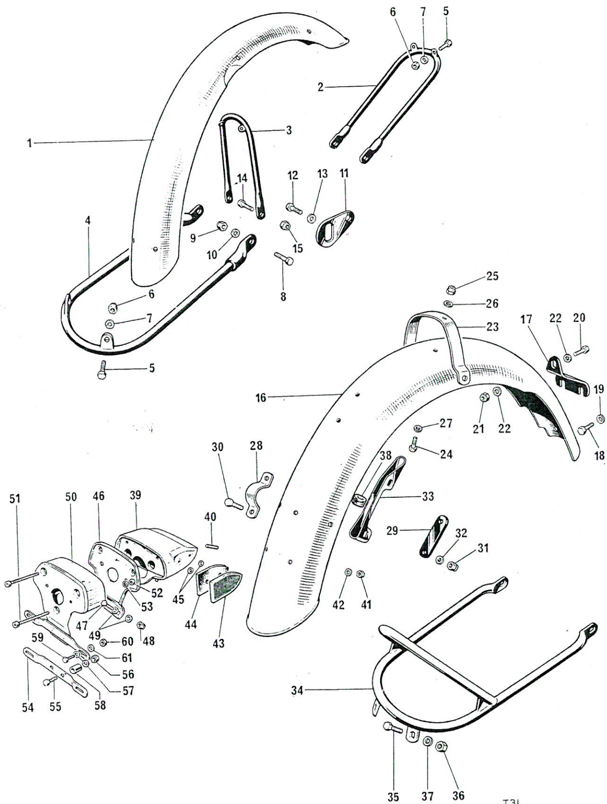
Fig. 27. MUDGUARDS (FENDERS)
