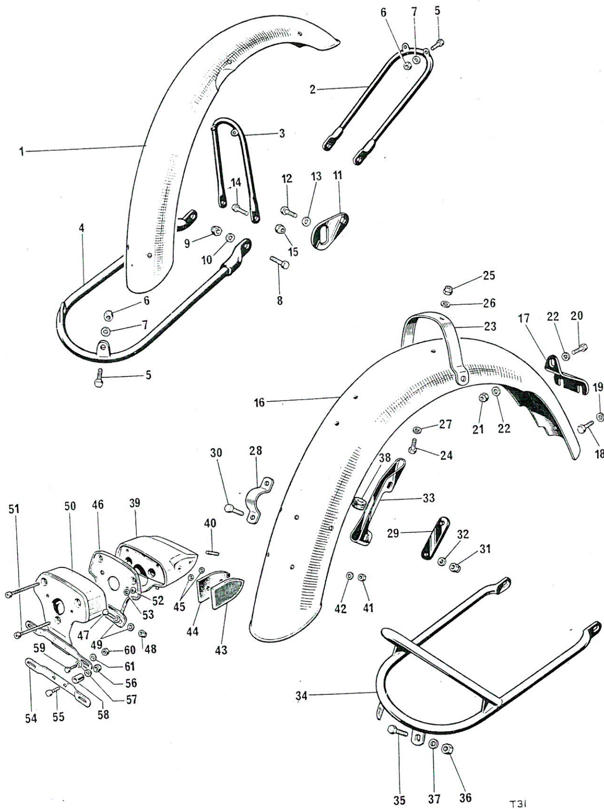
Fig. 28. MUDGUARDS (FENDERS)
