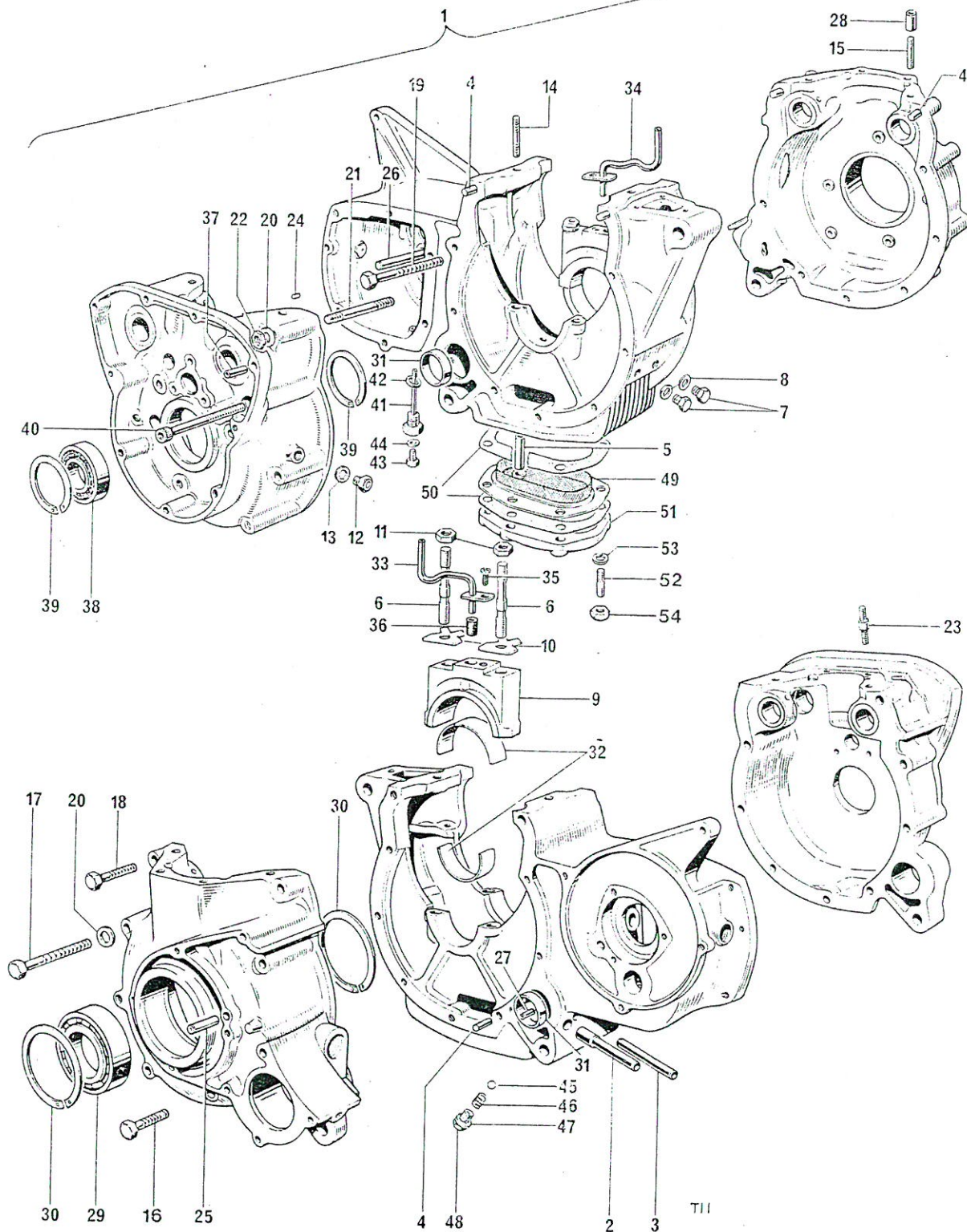
Fig. 2. CRANKCASES
