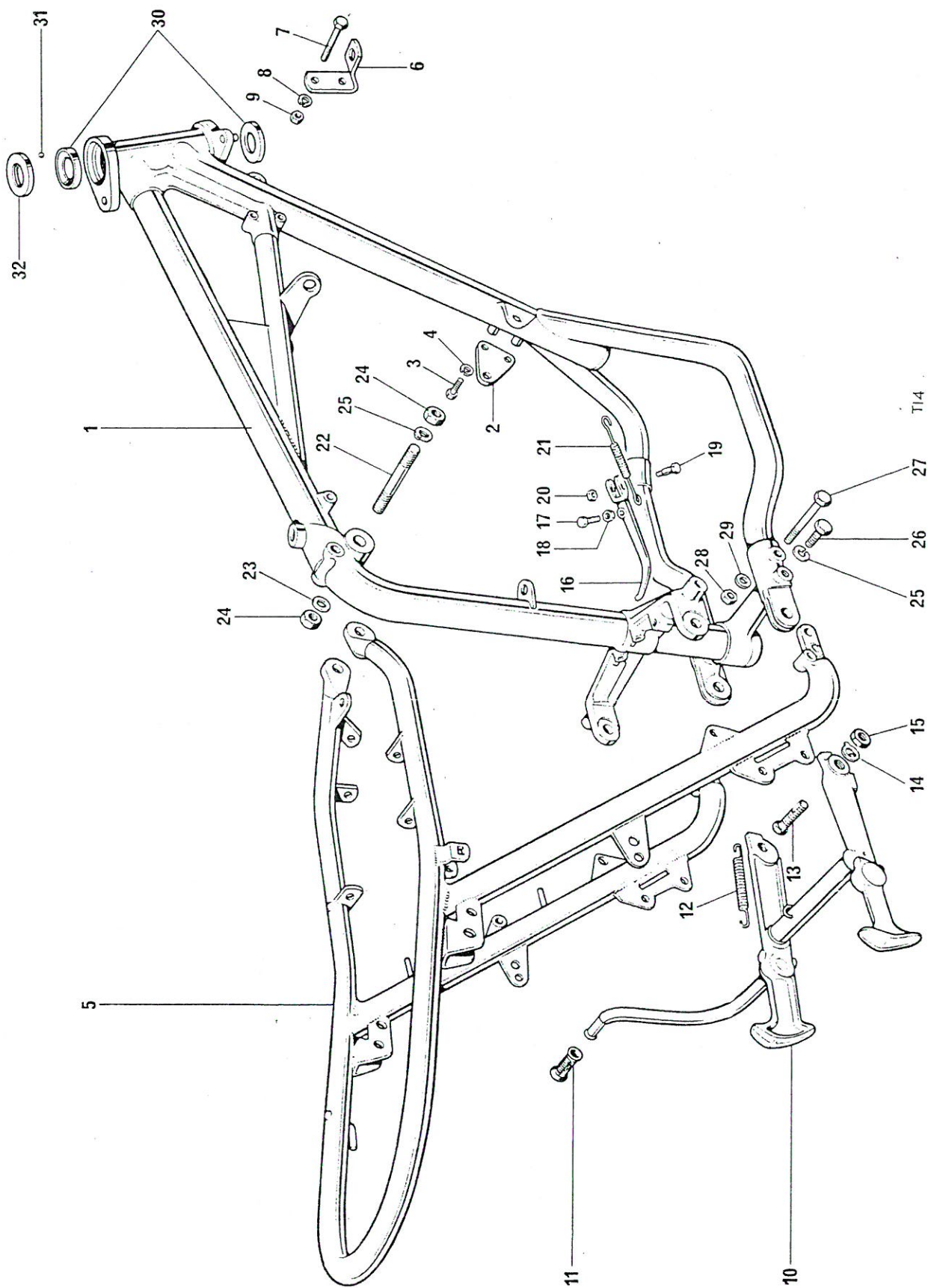
Fig. 14. FRAME
