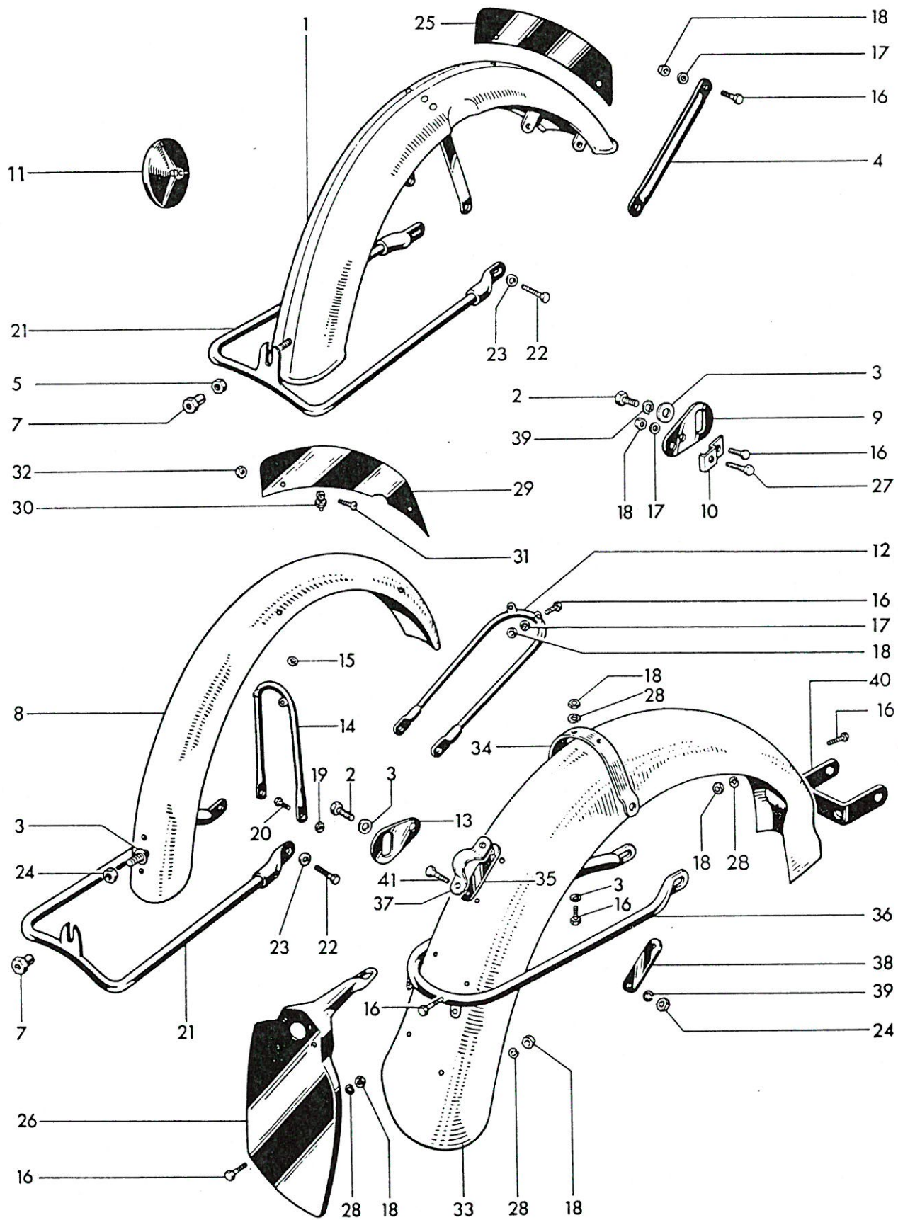
Fig. 20. MUDGUARDS
