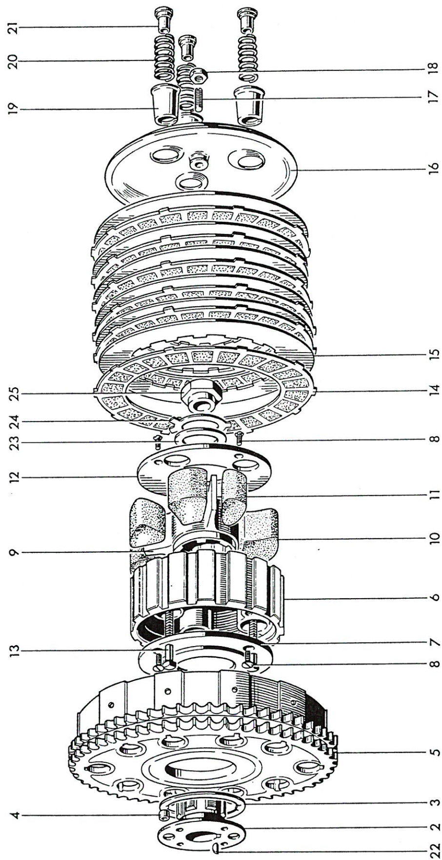
Fig. 9. CLUTCH
