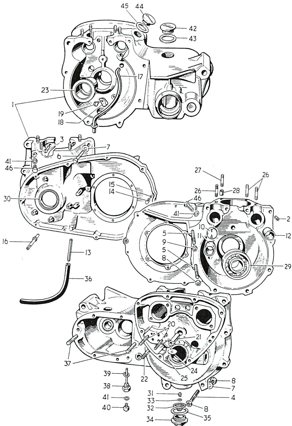
Fig. 2. CRANKCASE
