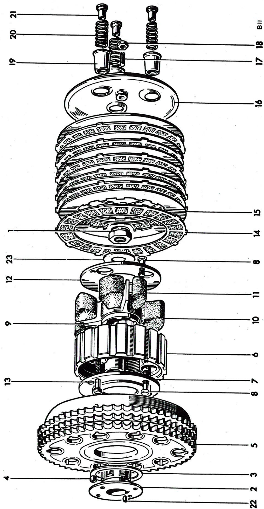
Fig. 14. CLUTCH
