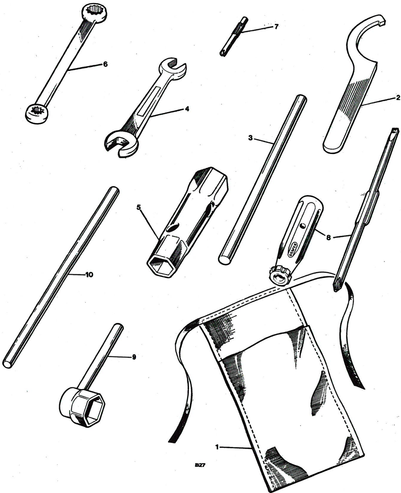
Fig. 31. TOOLKIT
