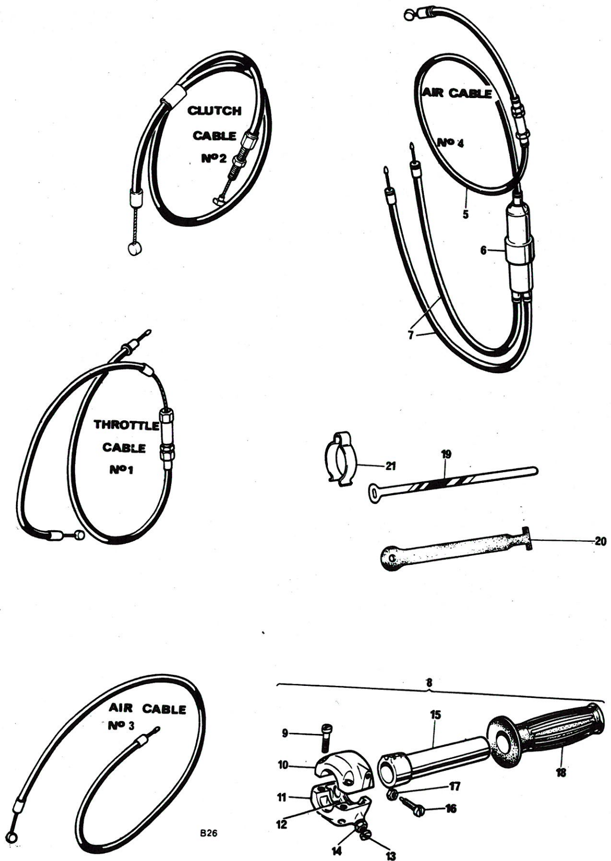
Fig. 30. CONTROL CABLES
