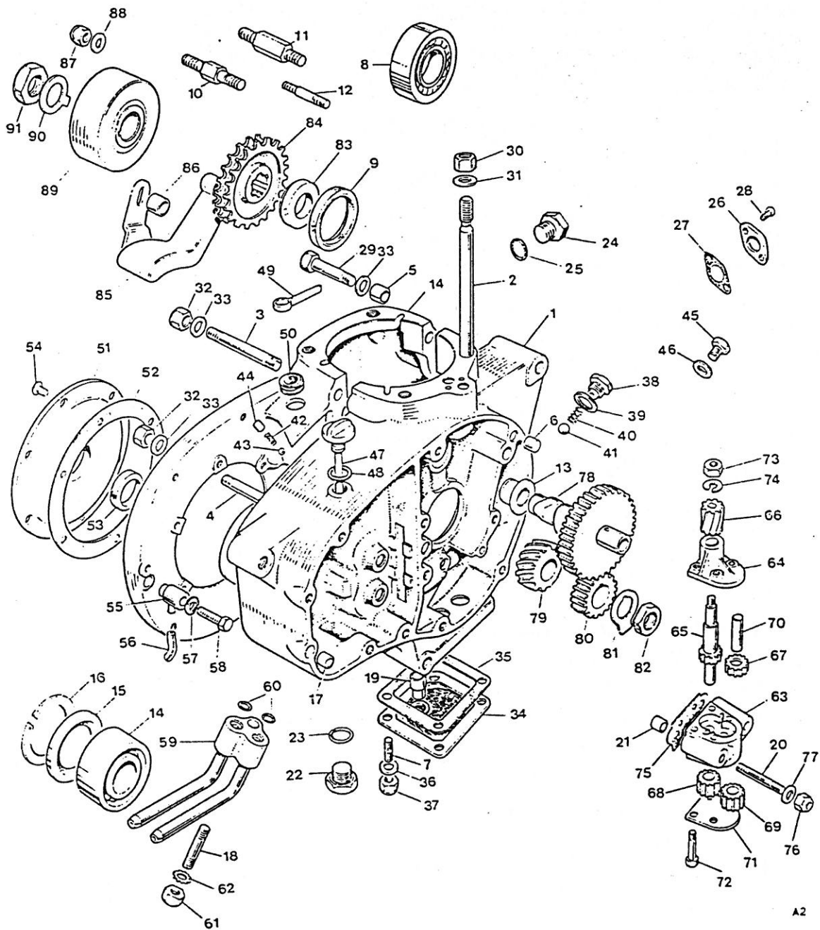
Fig. 2. CRANKCASE
