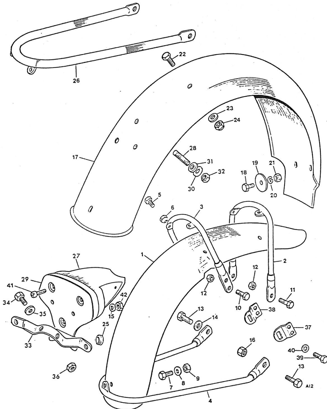
Fig. 12. FENDERS
