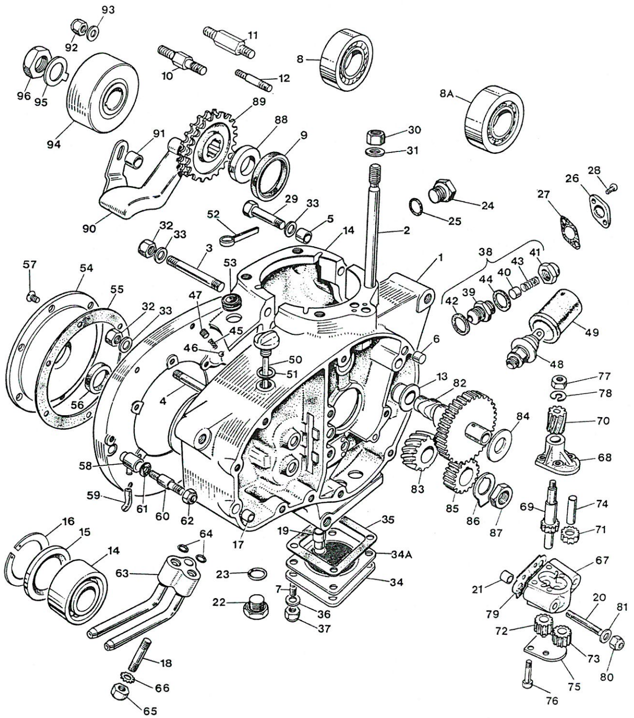
Fig. 2. CRANKCASE
