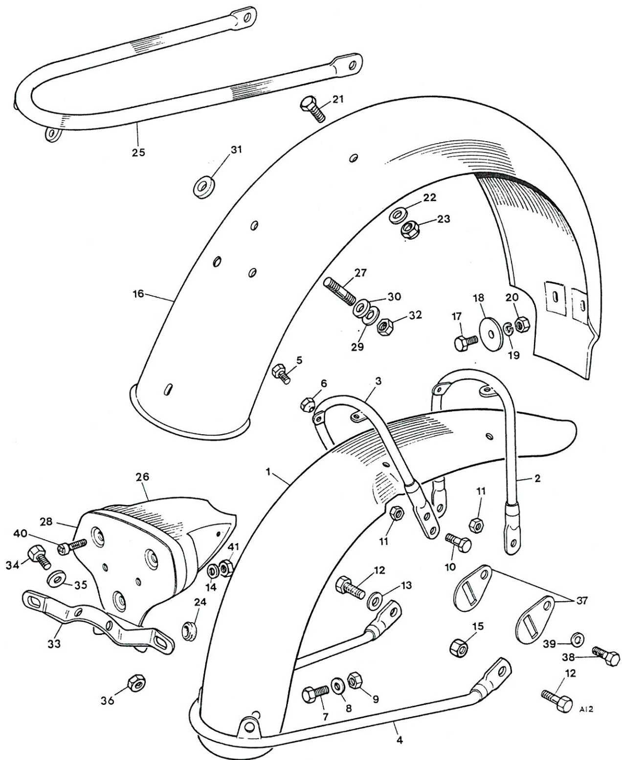
Fig. 12. FENDERS
