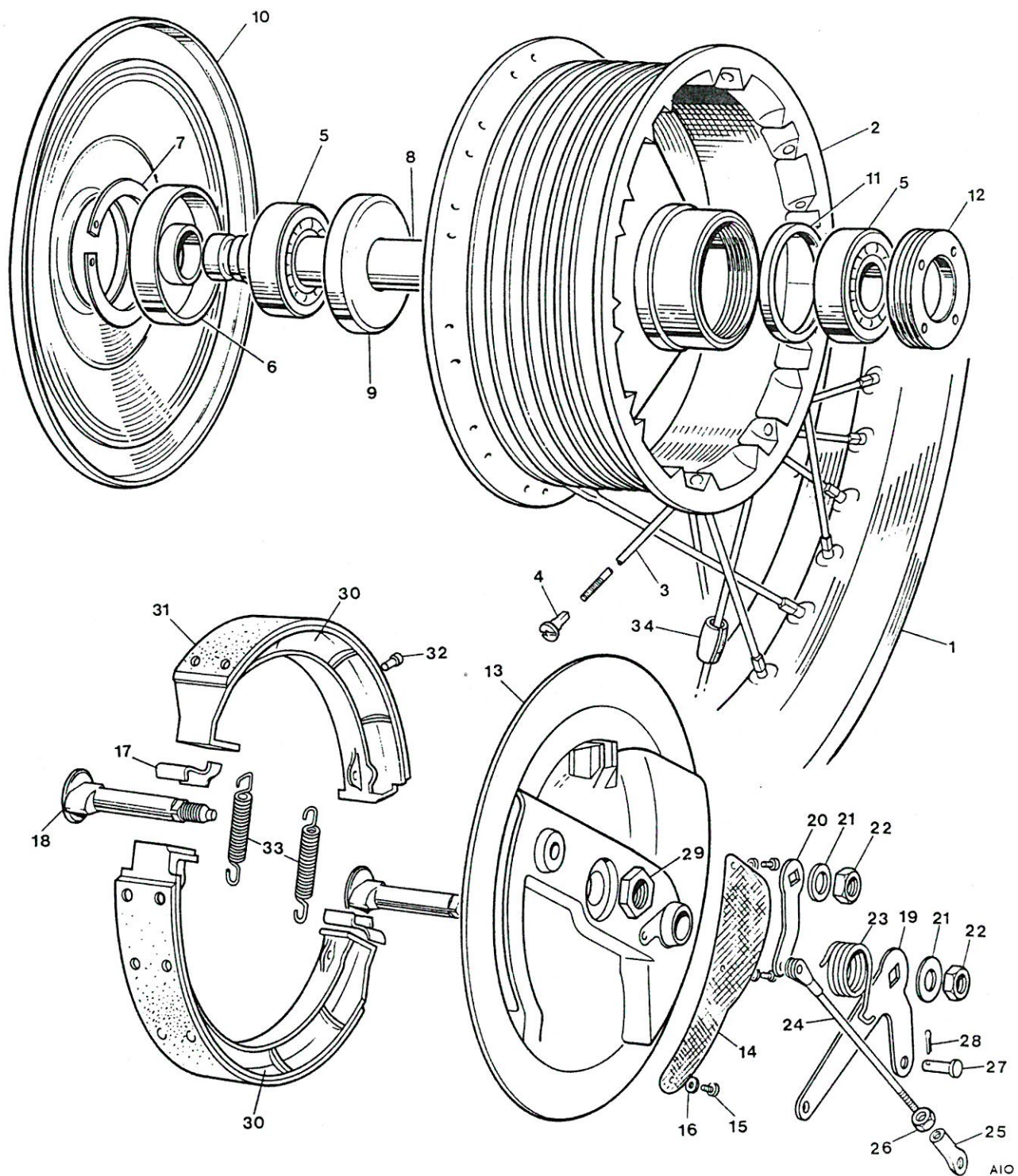
Fig. 10. FRONTWHEEL
