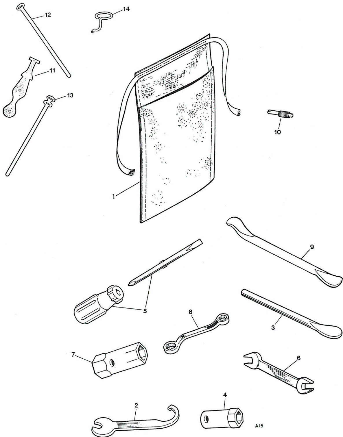
Fig. 17. TOOL KIT
