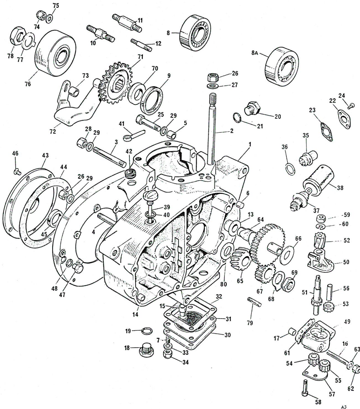
Fig. 3. CRANKCASE
