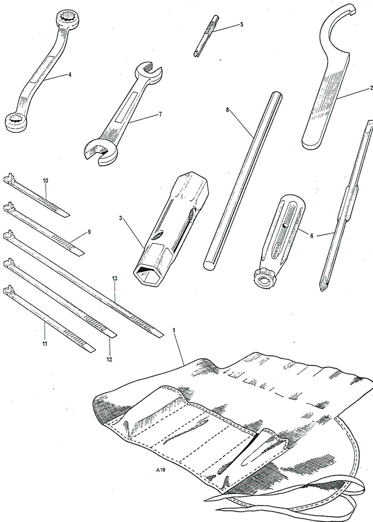
Fig. 19. TOOL KIT
