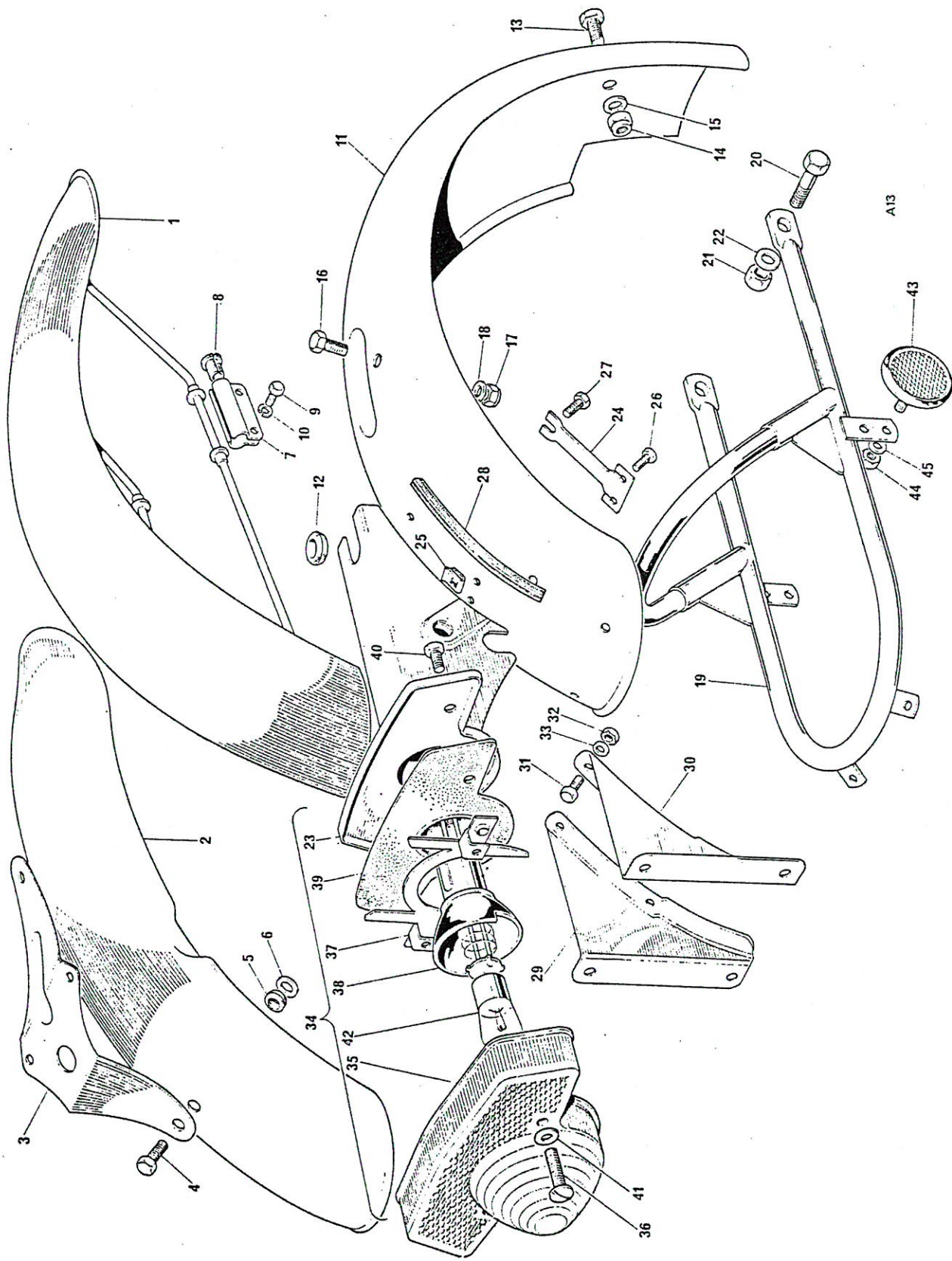
Fig. 13. FENDERS
