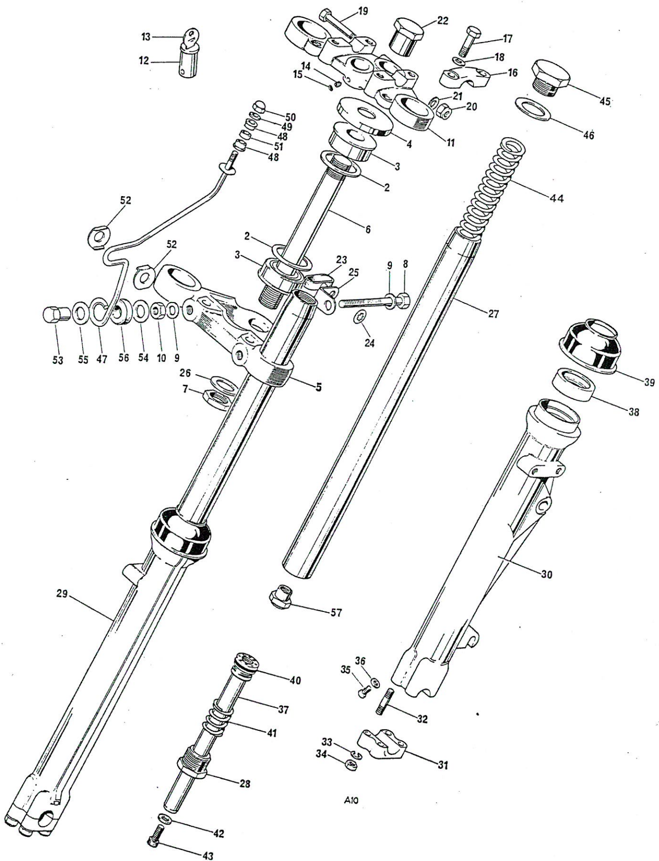
Fig. 10. TELESCOPIC FORKS
