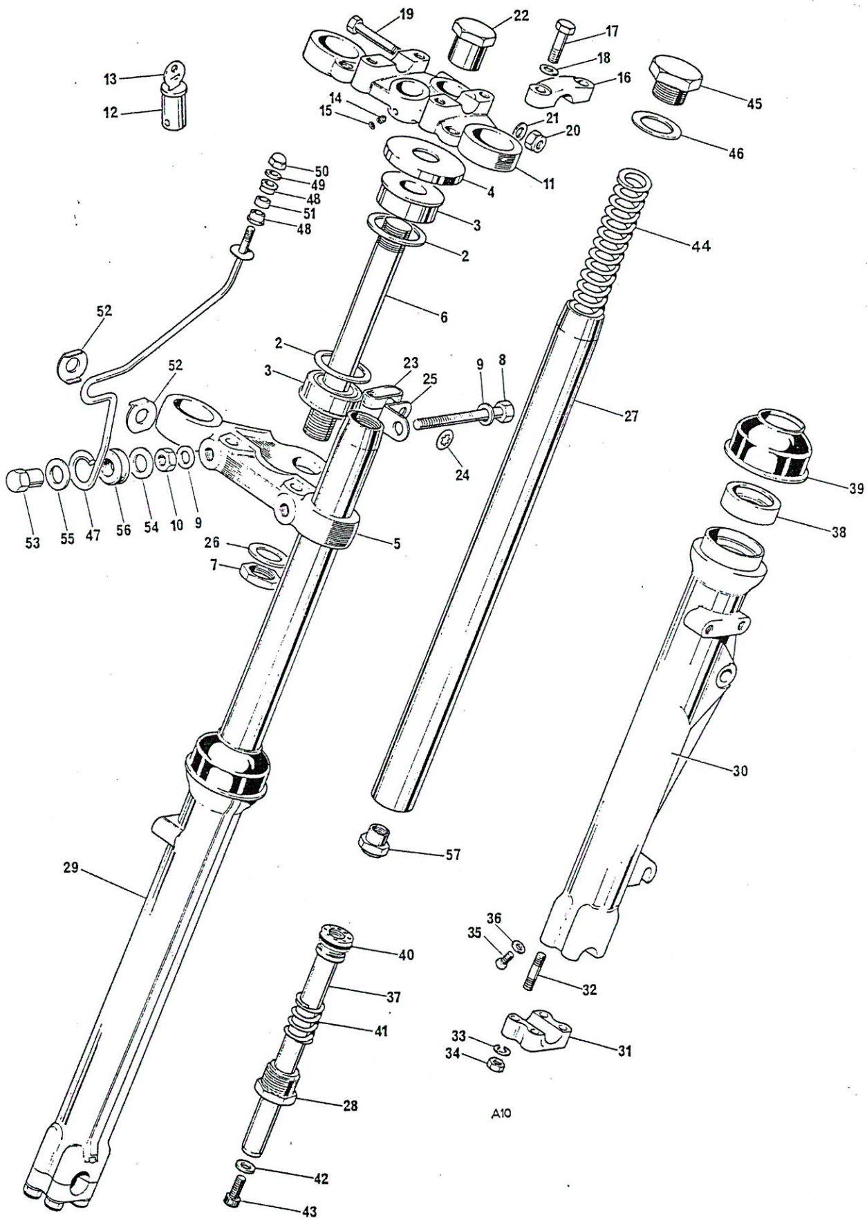
Fig. 10. TELESCOPIC FORKS
