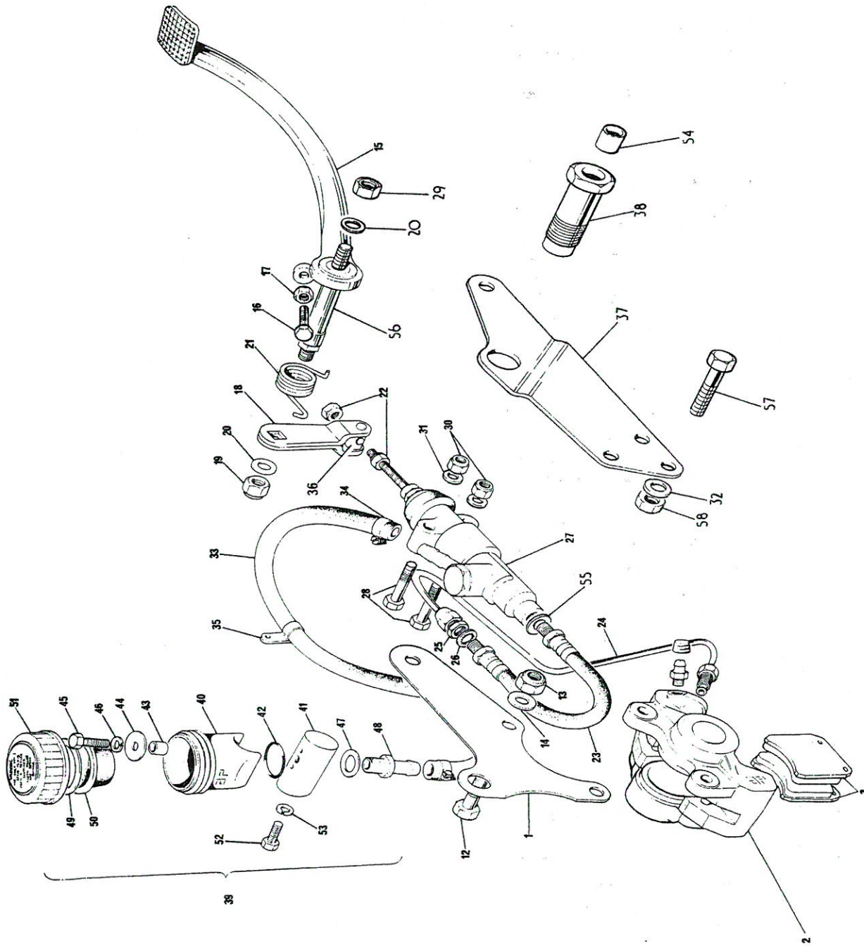
Fig. 25. REAR BRAKE
