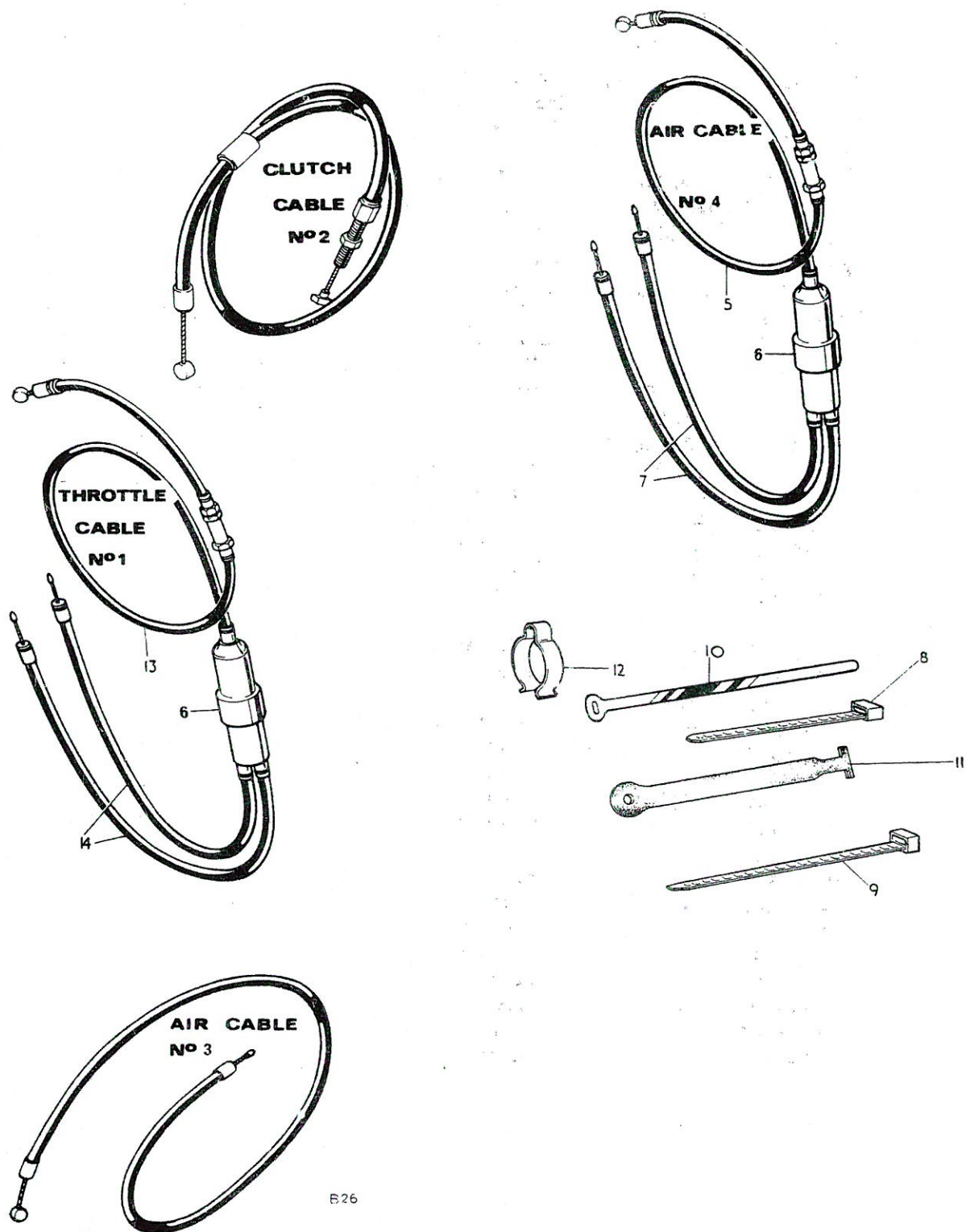
Fig. 30. CONTROL CABLES
