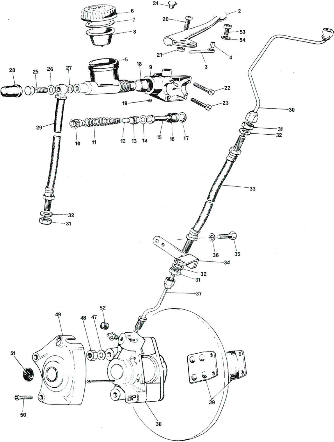
Fig. 23. FRONT BRAKE
