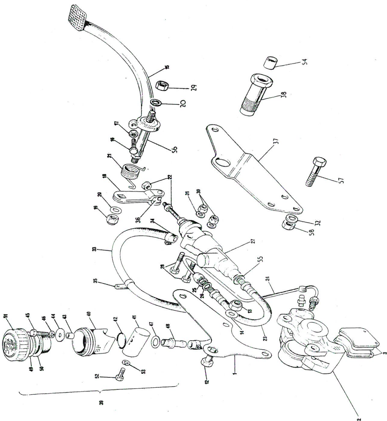
Fig. 25. REAR BRAKE
