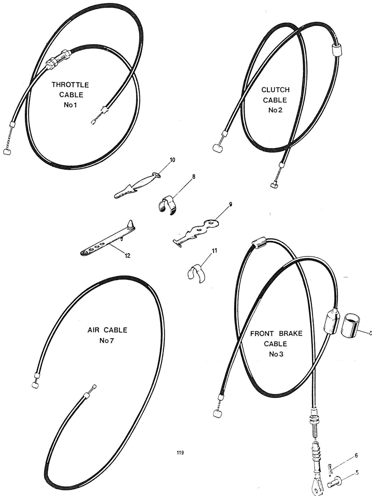
Fig. 21. CONTROL CABLES
