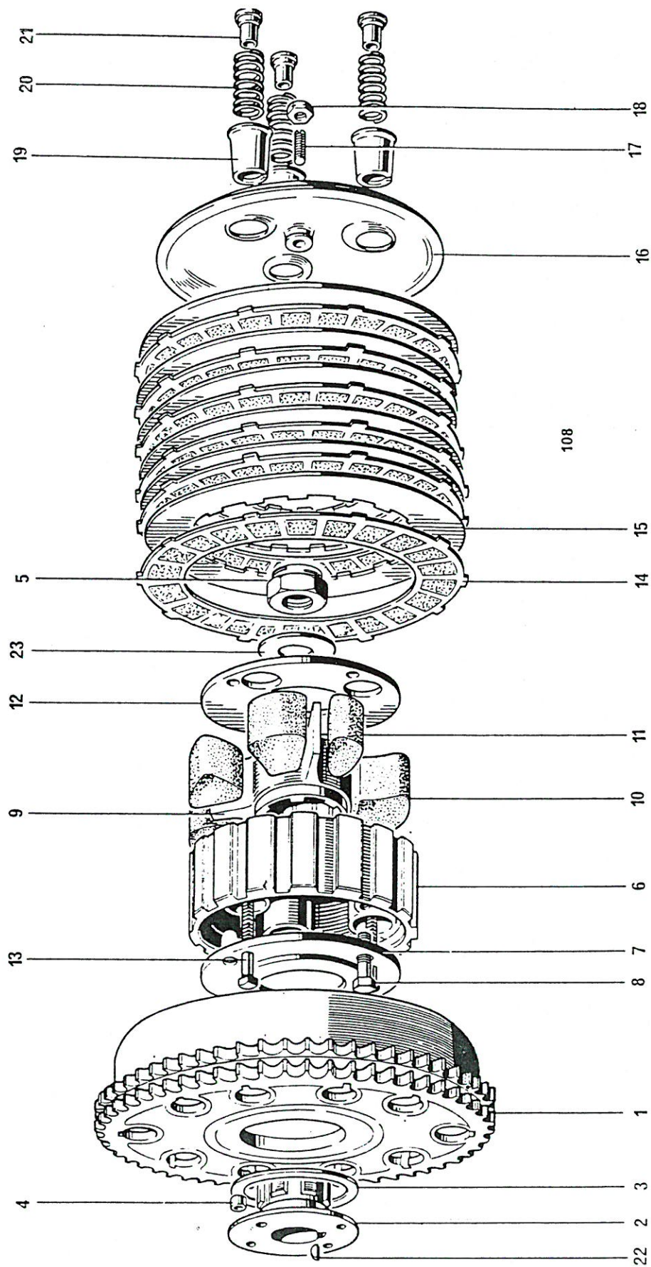
Fig. 10. CLUTCH
