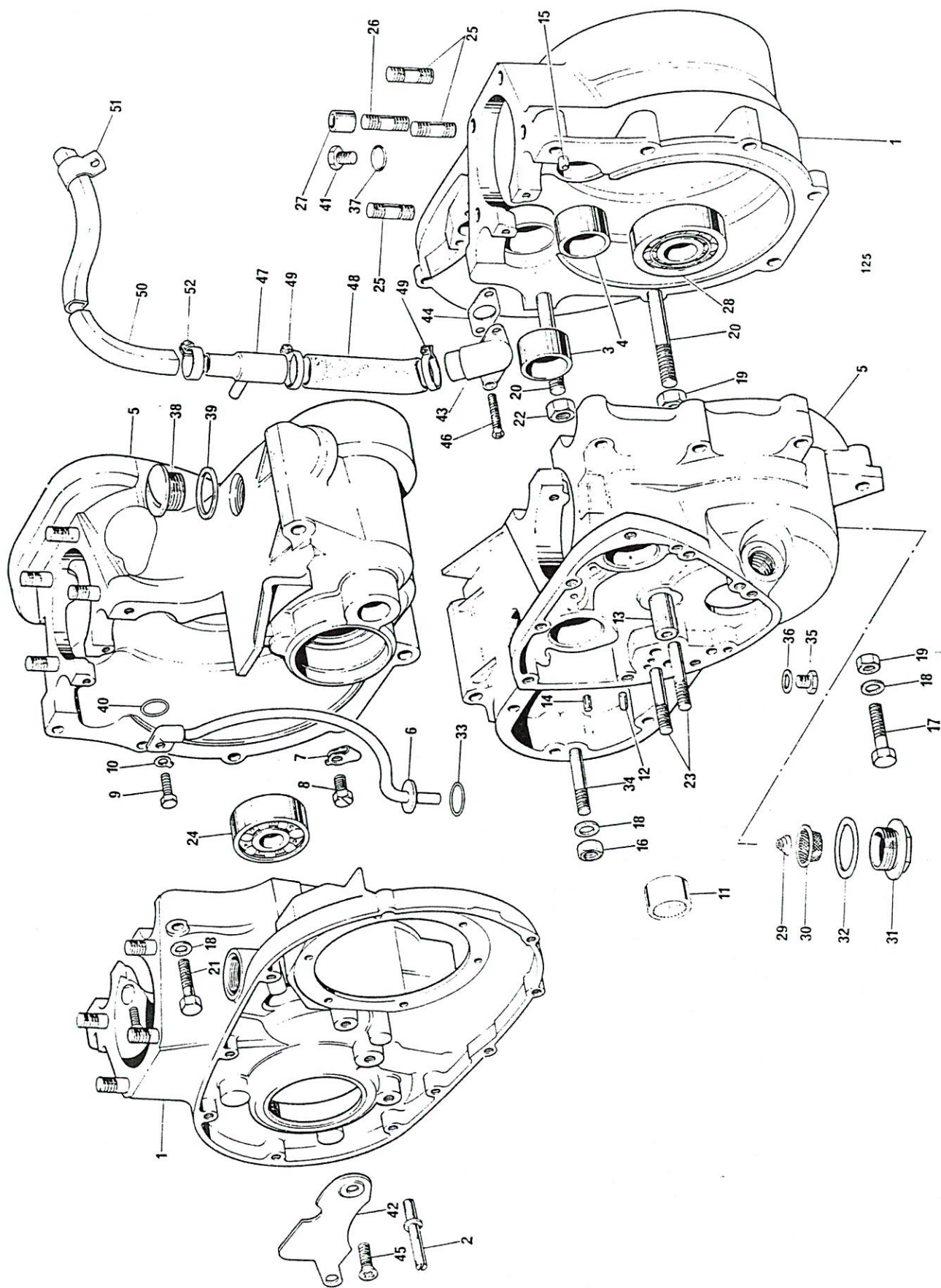
Fig. 2. CRANKCASE
