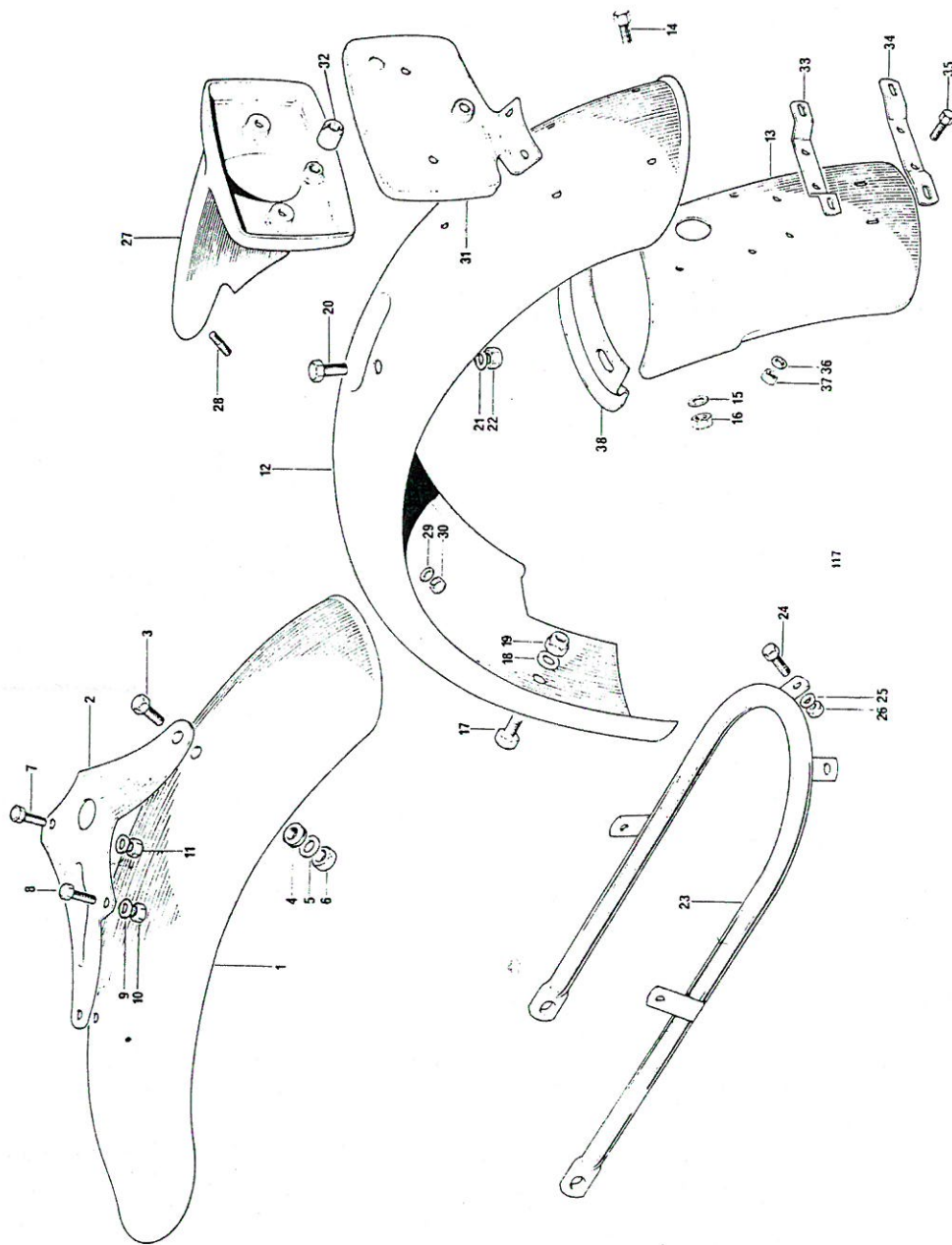
Fig. 18. FENDERS
