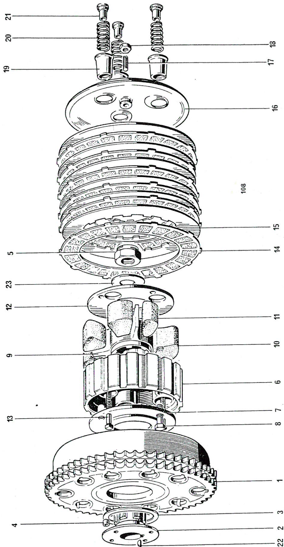
Fig. 9. CLUTCH
