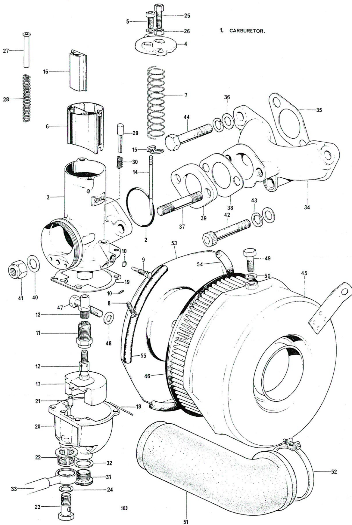
Fig. 4. CARBURETOR
