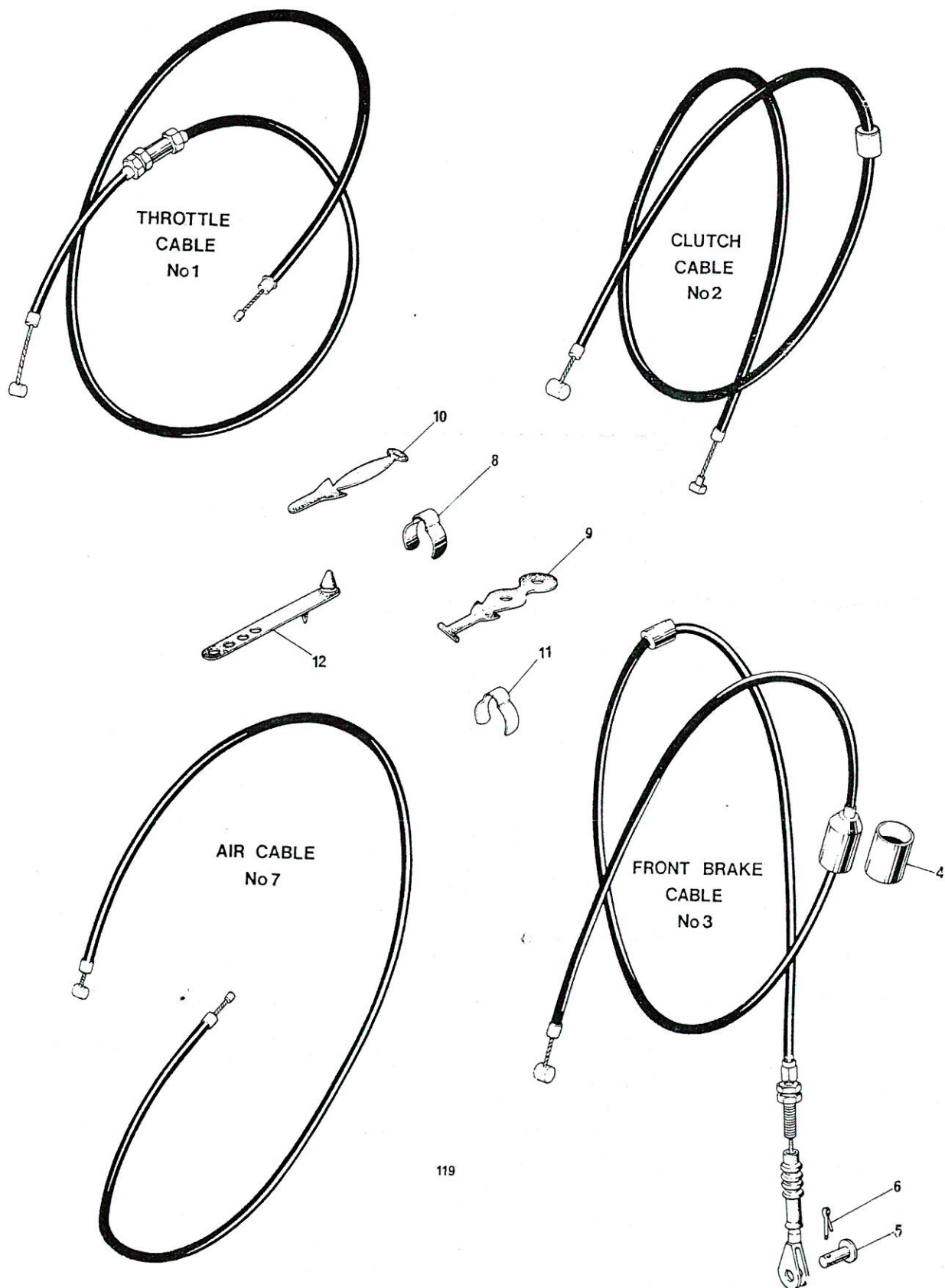
Fig. 20. CONTROL CABLES
