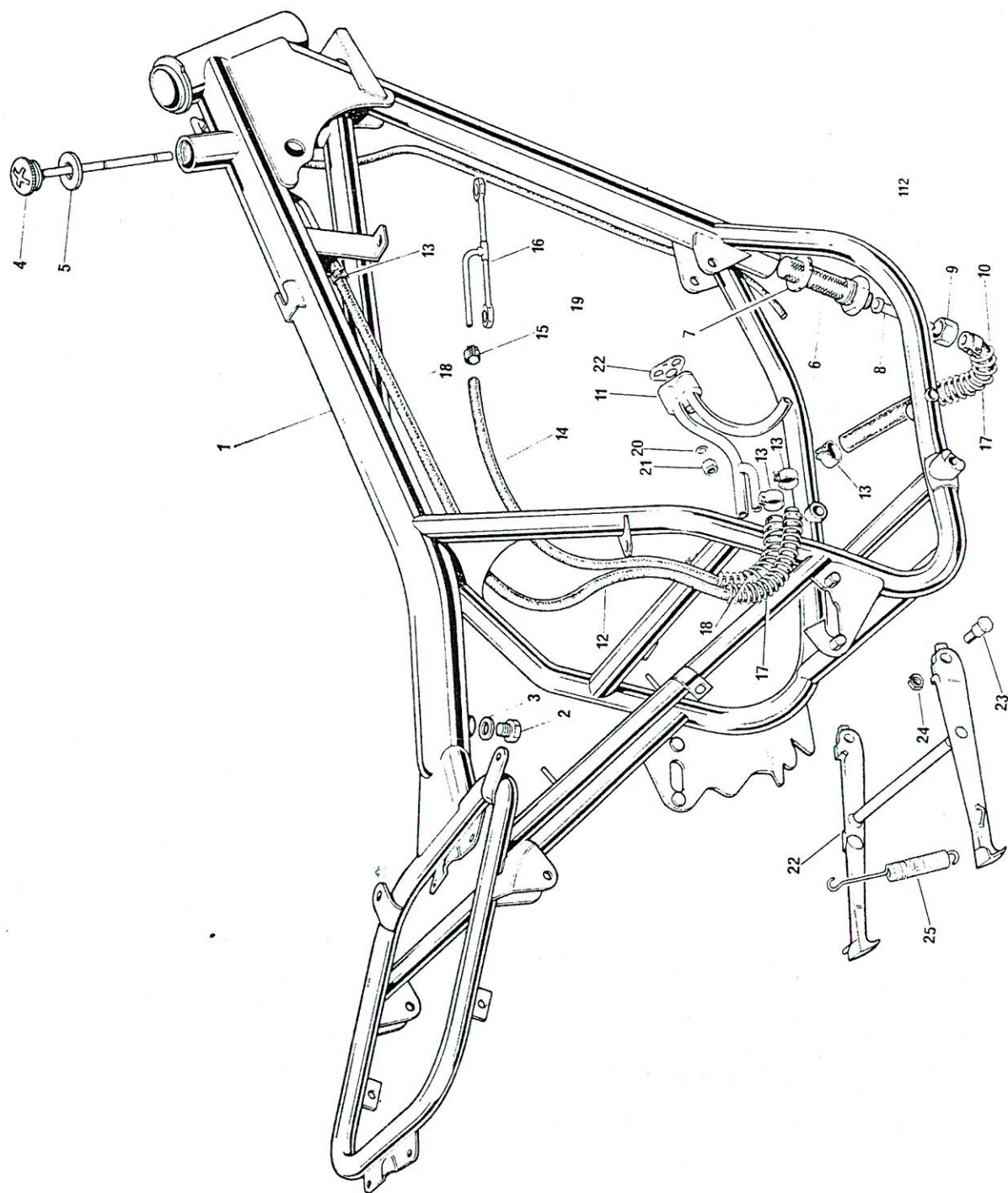
Fig. 13. FRAME
