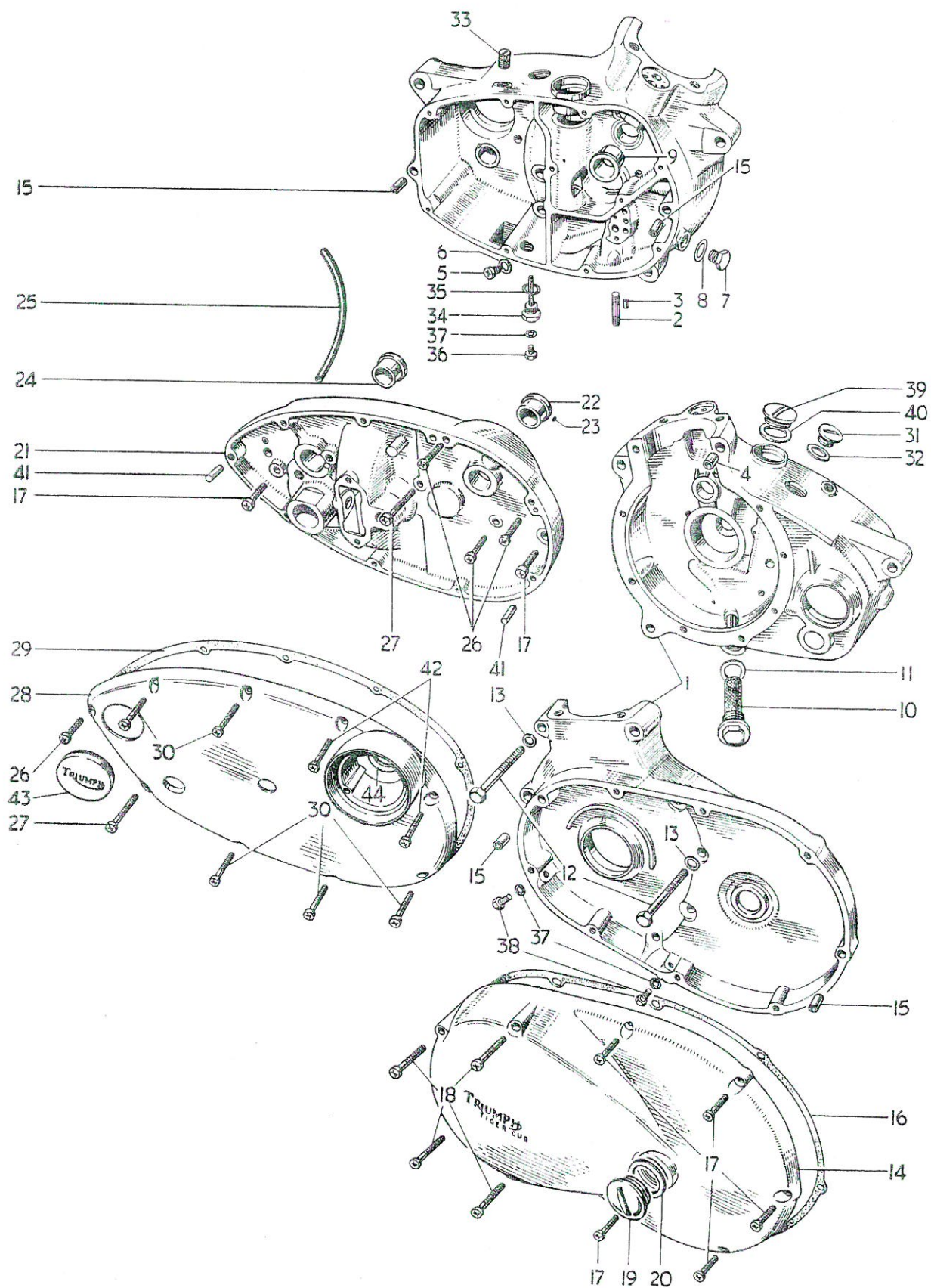
Fig. 2. CRANKCASE
