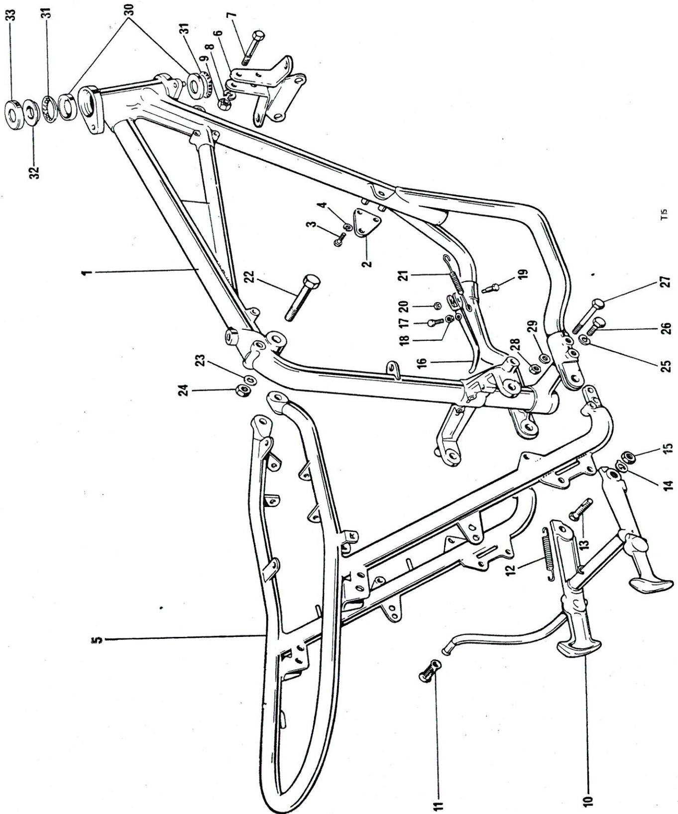
Fig. 15. FRAME
