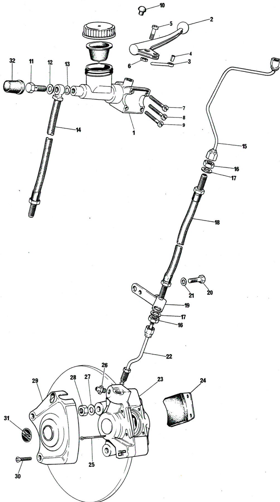
Fig. 21. FRONT BRAKE
