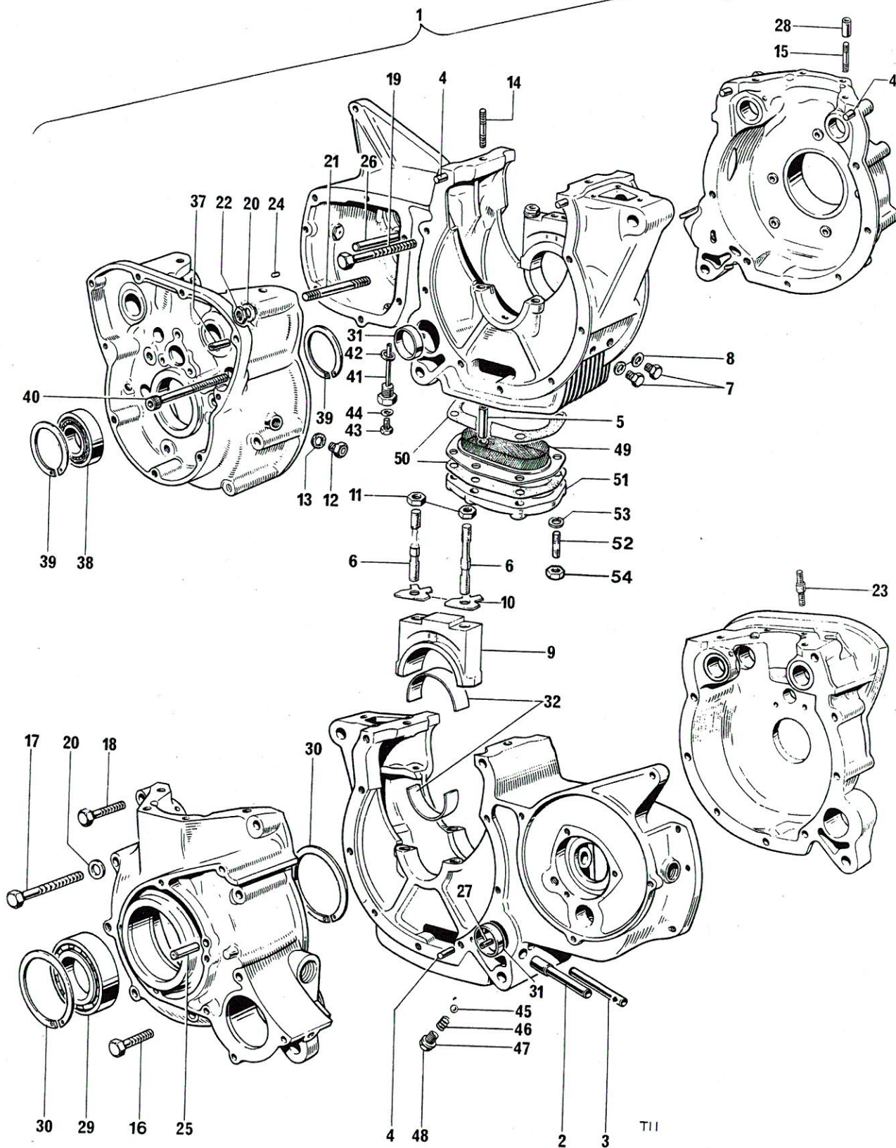
Fig. 2. CRANKCASES
