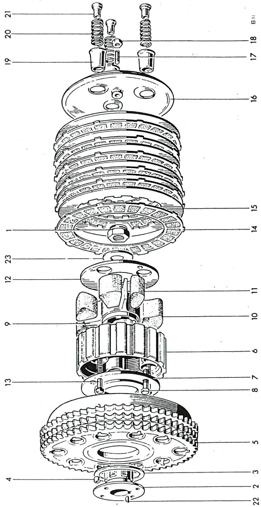
Fig. 14. CLUTCH
