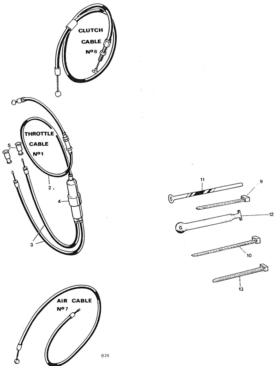
Fig. 30. CONTROL CABLES
