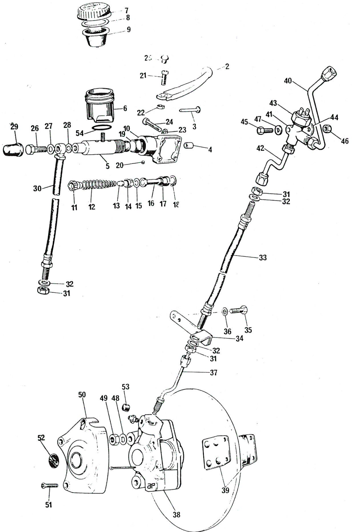
Fig. 23. FRONT BRAKE
