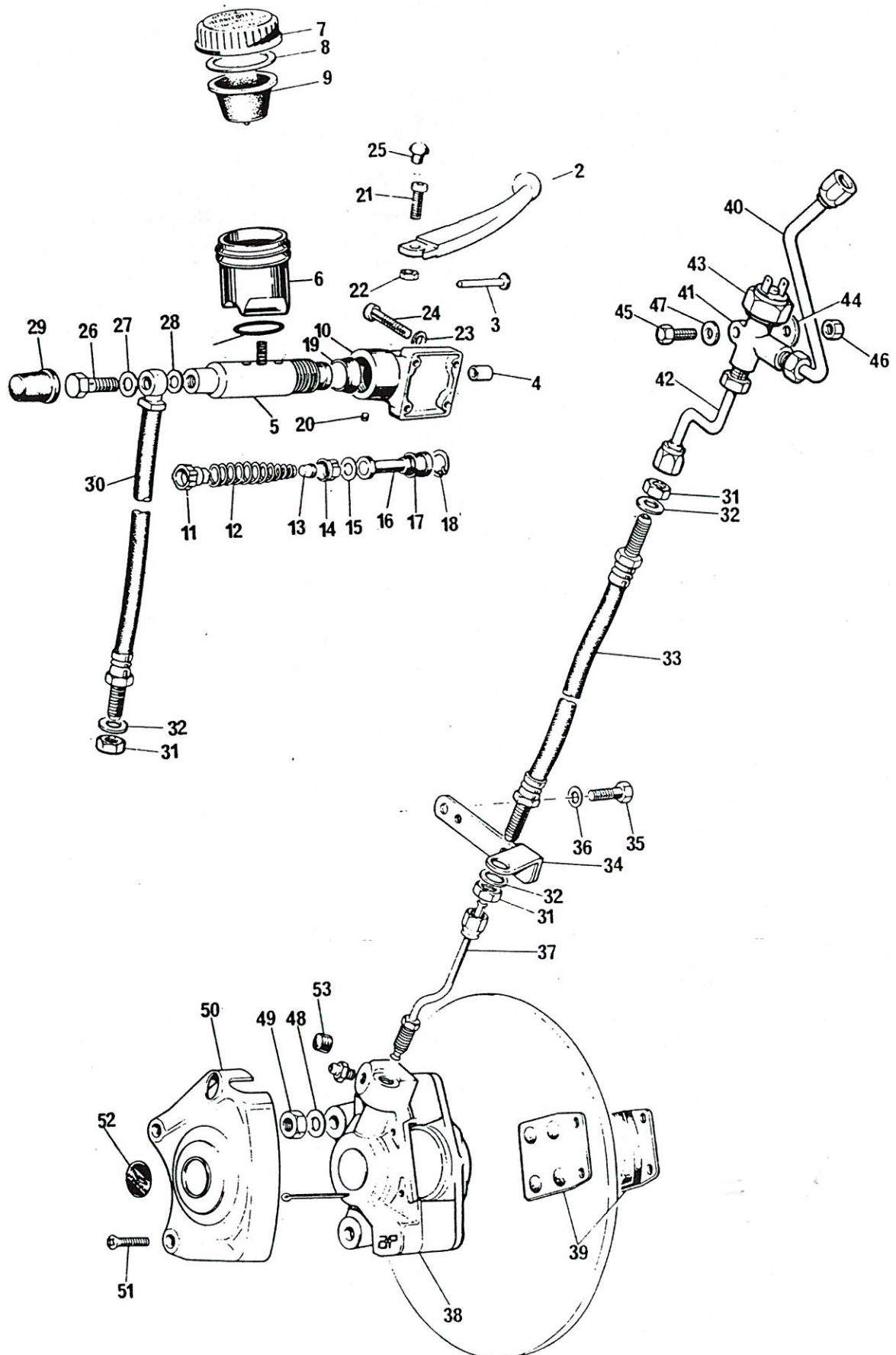
Fig. 23. FRONT BRAKE
