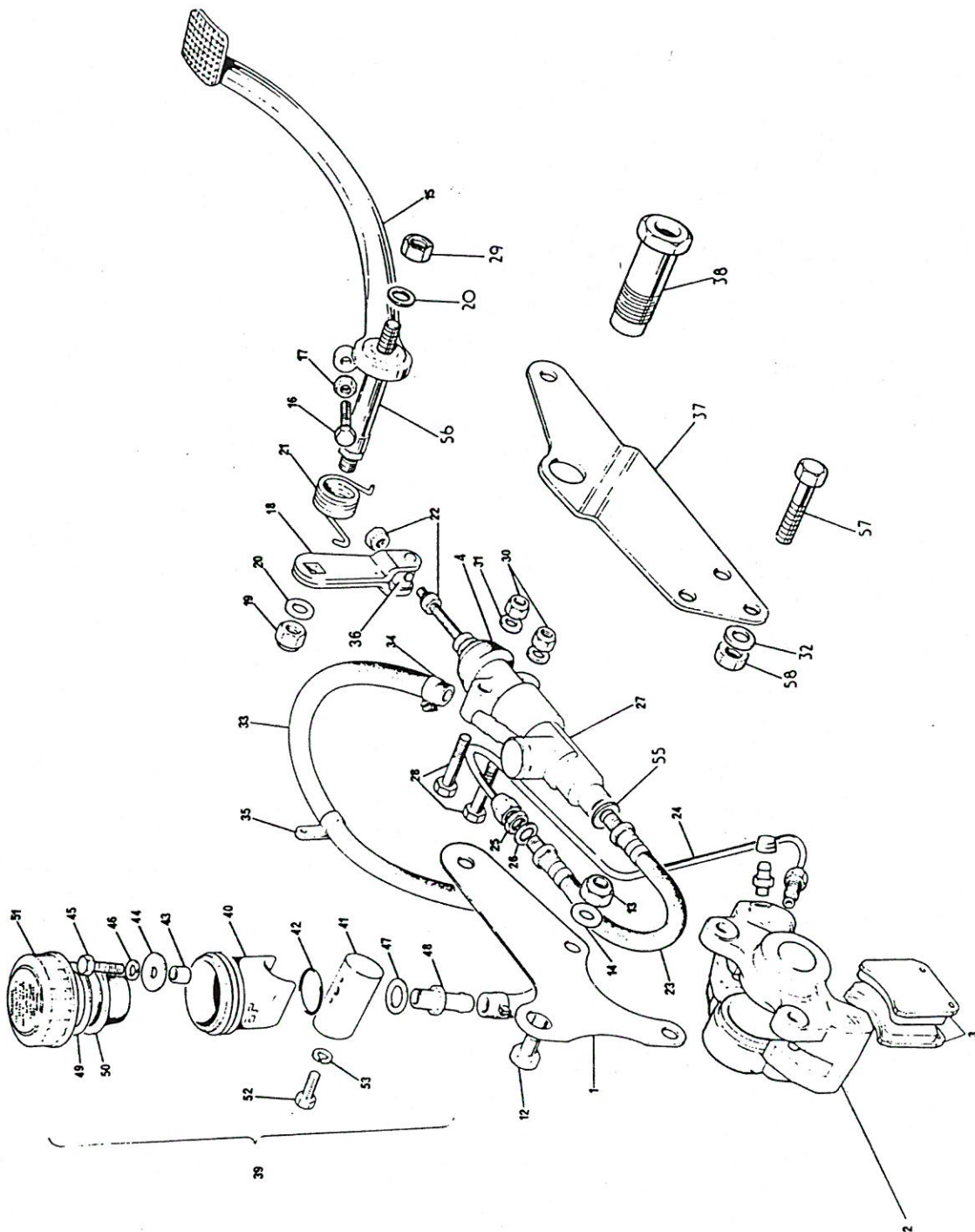
Fig. 25. REAR BRAKE
