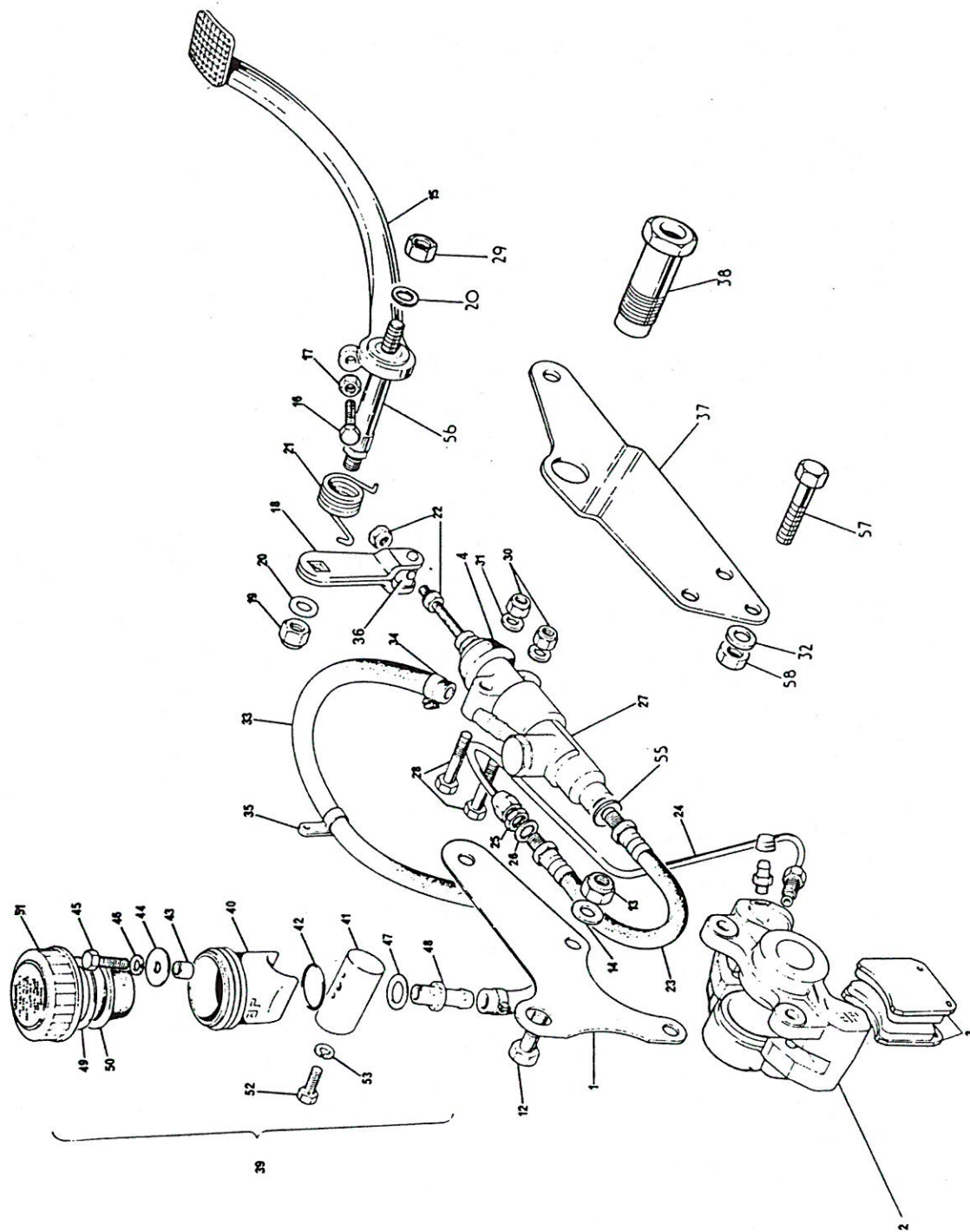
Fig. 25. REAR BRAKE
