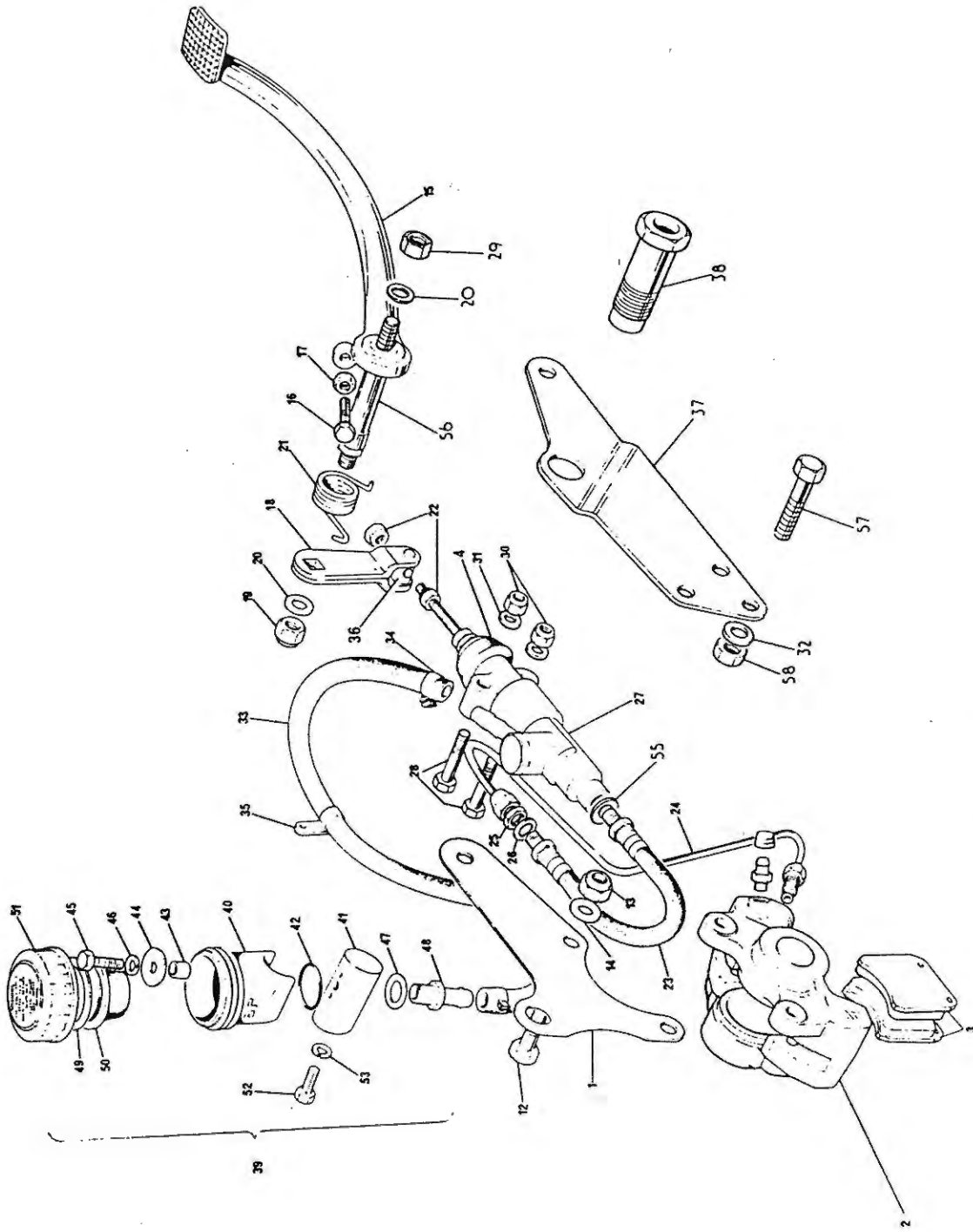
Fig. 25. REAR BRAKE
