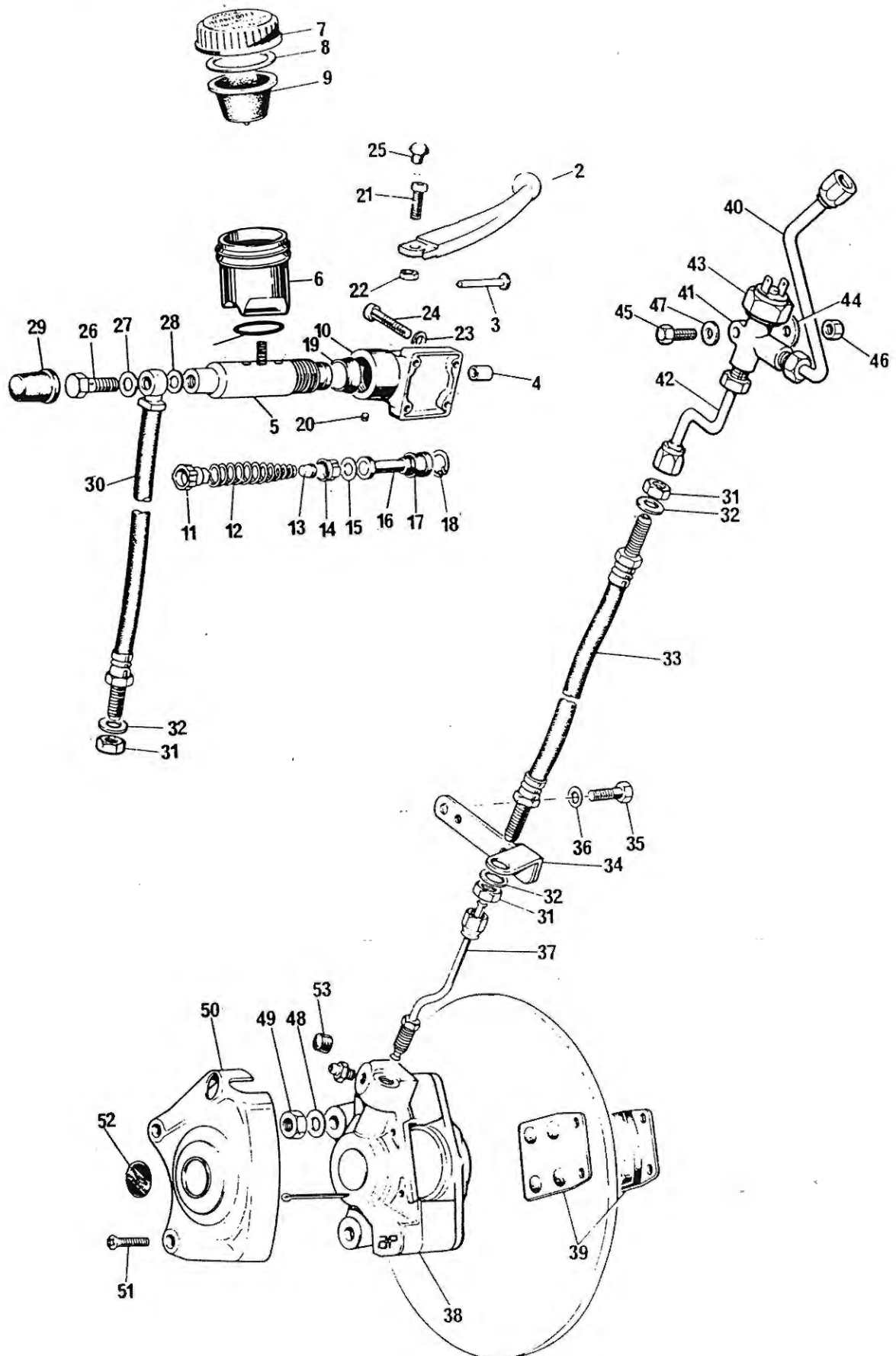
Fig. 23. FRONT BRAKE
