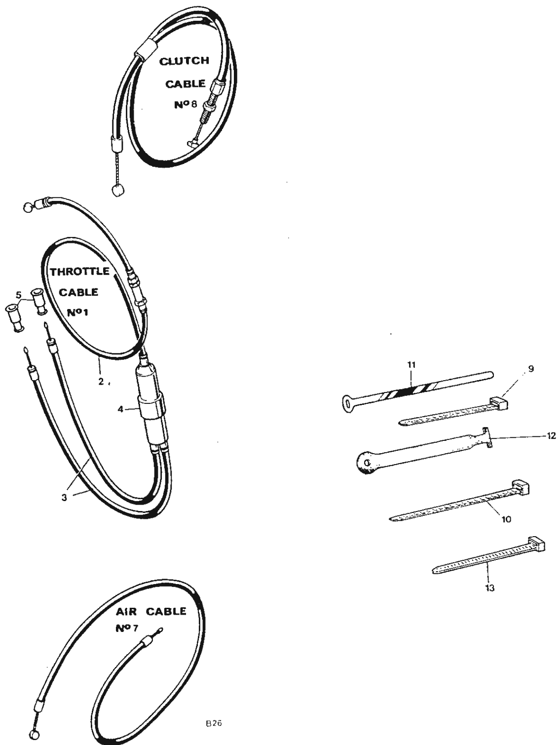
Fig. 30. CONTROL CABLES
