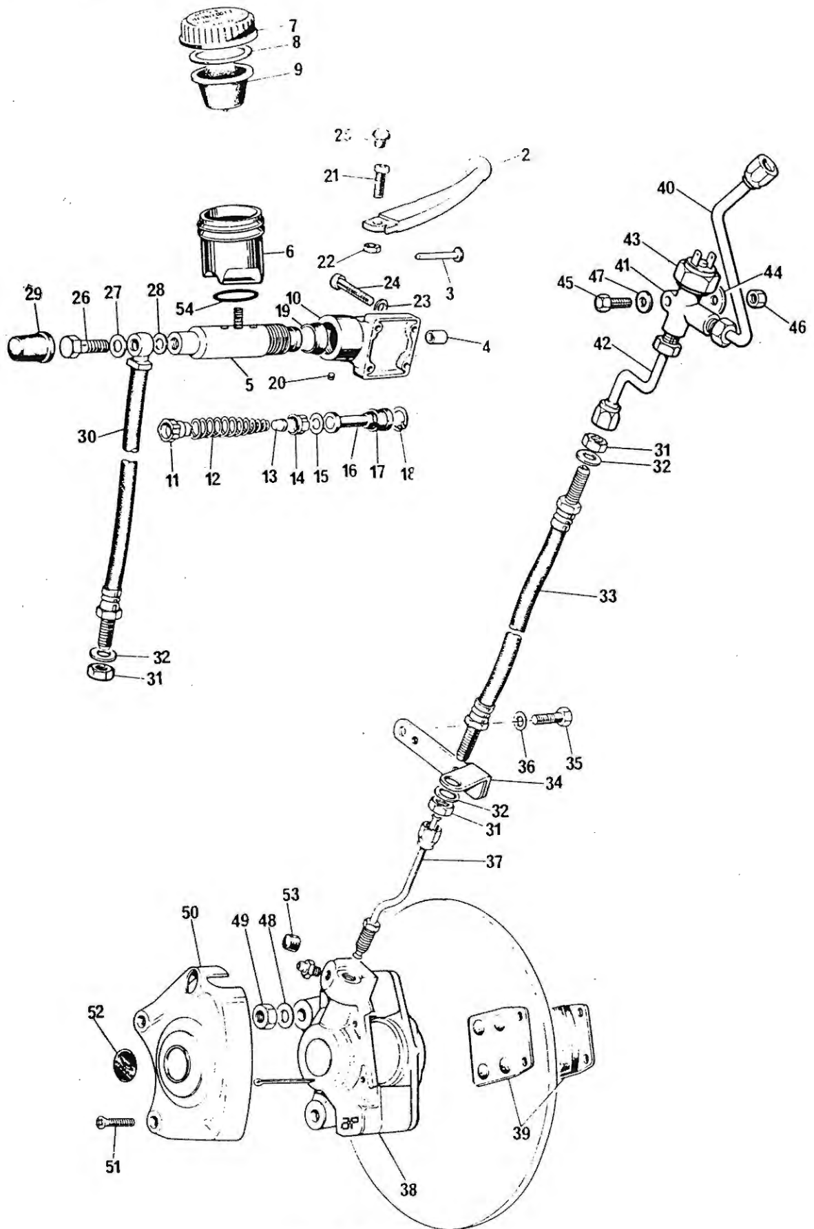
Fig. 23. FRONT BRAKE
