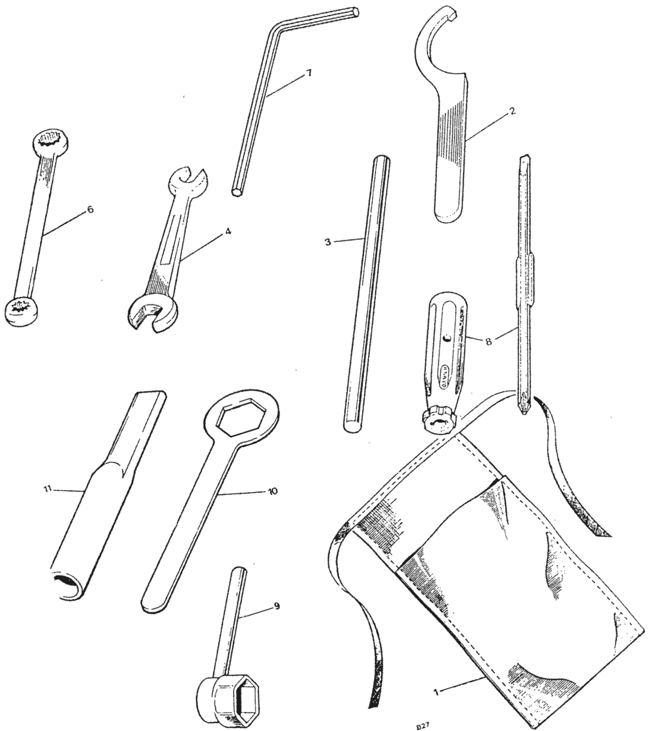
Fig. 31. TOOLKIT
