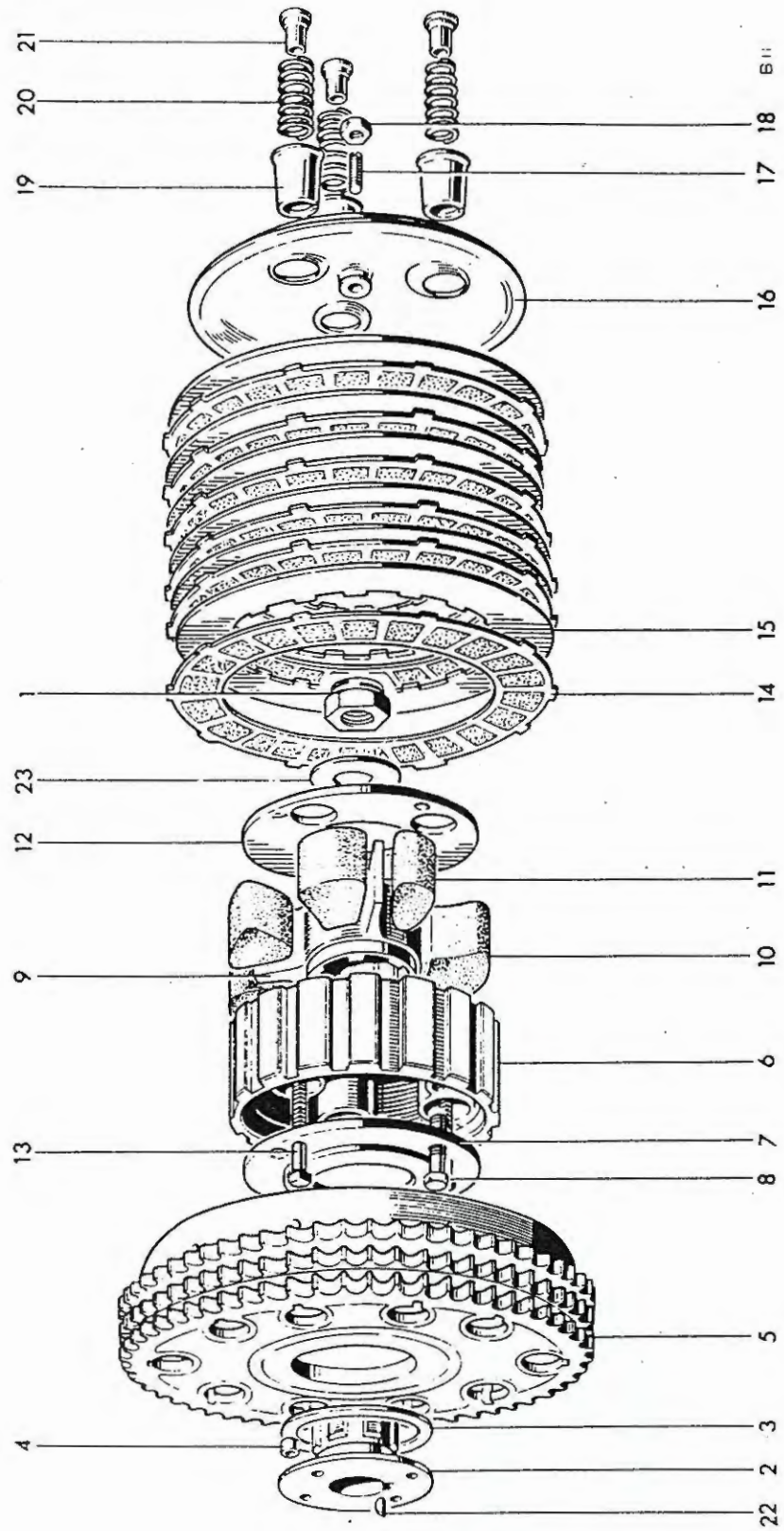
Fig. 14. CLUTCH
