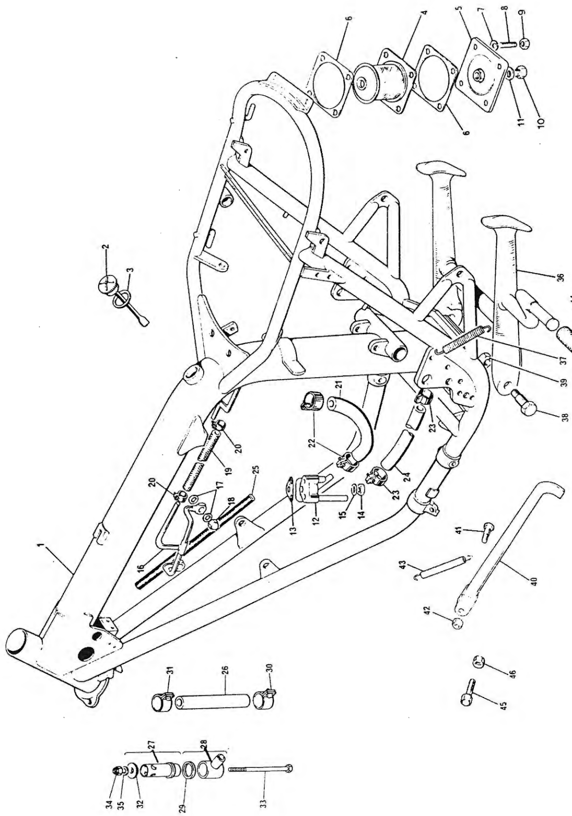
Fig. 16. FRAME
