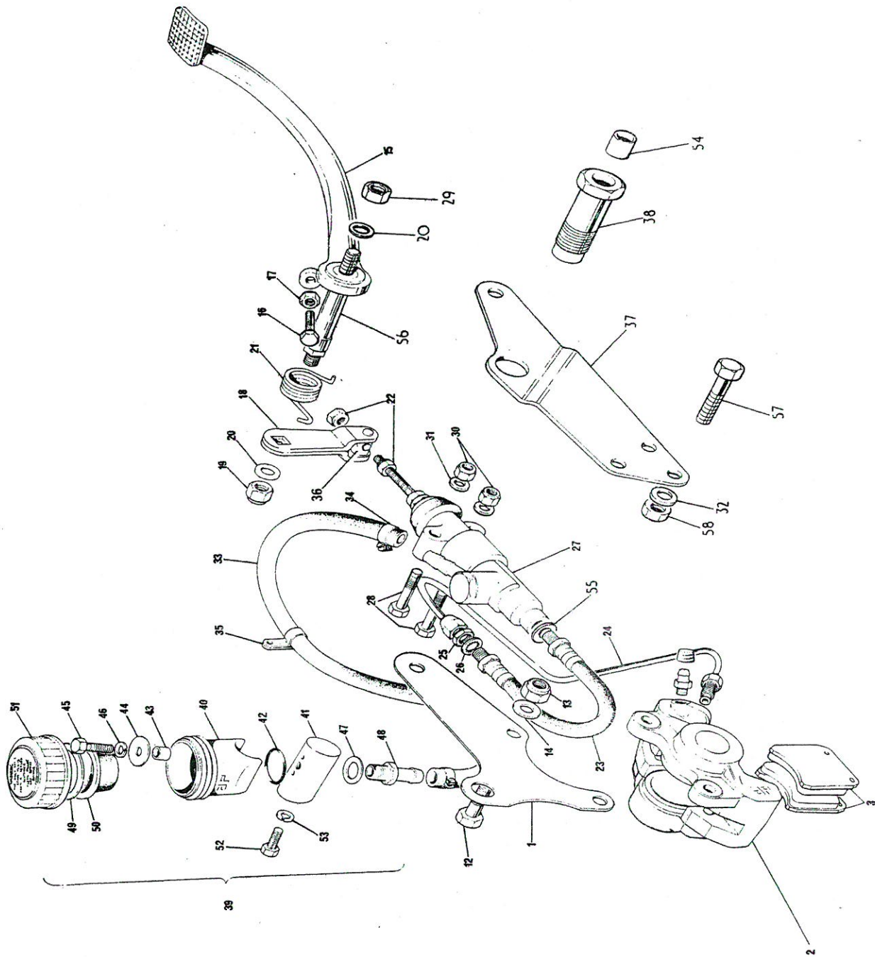
Fig. 25. REAR BRAKE
