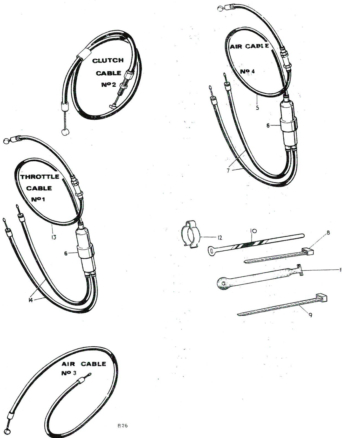
Fig. 30. CONTROL CABLES
