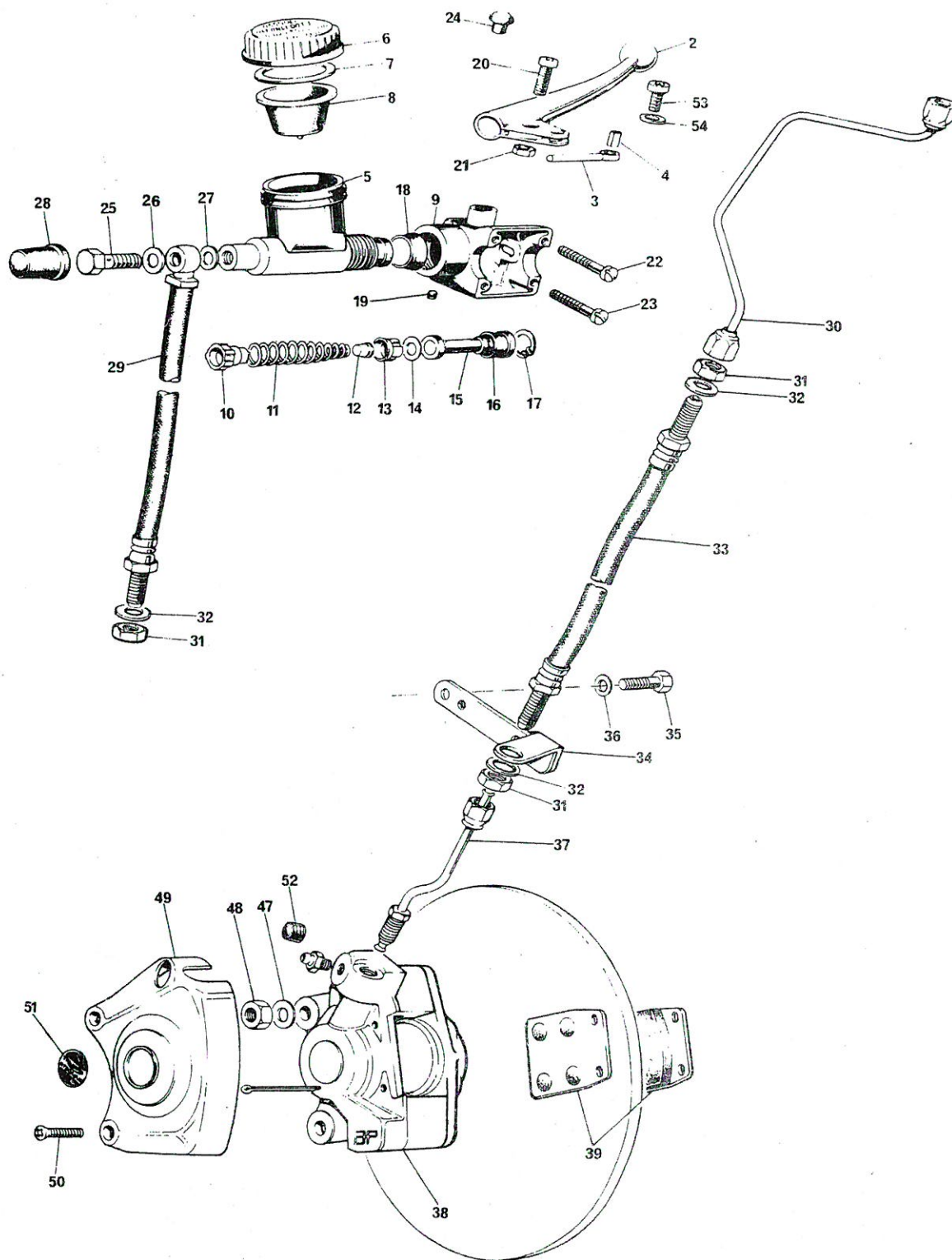
Fig. 23. FRONT BRAKE
