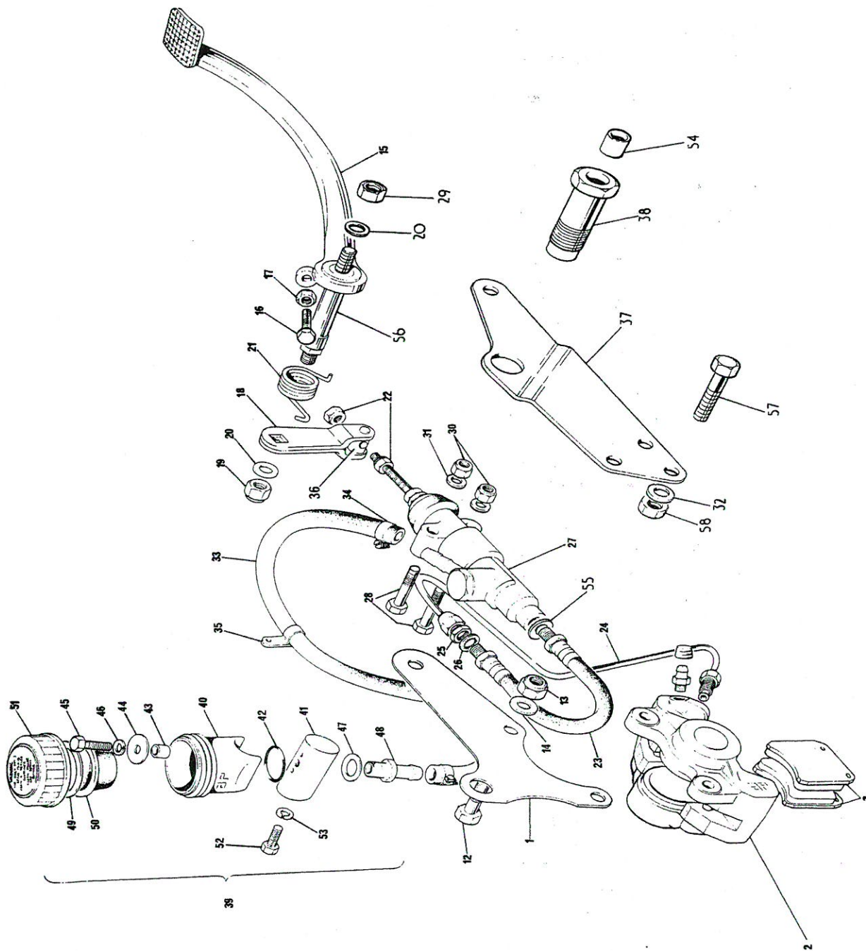
Fig. 25. REAR BRAKE
