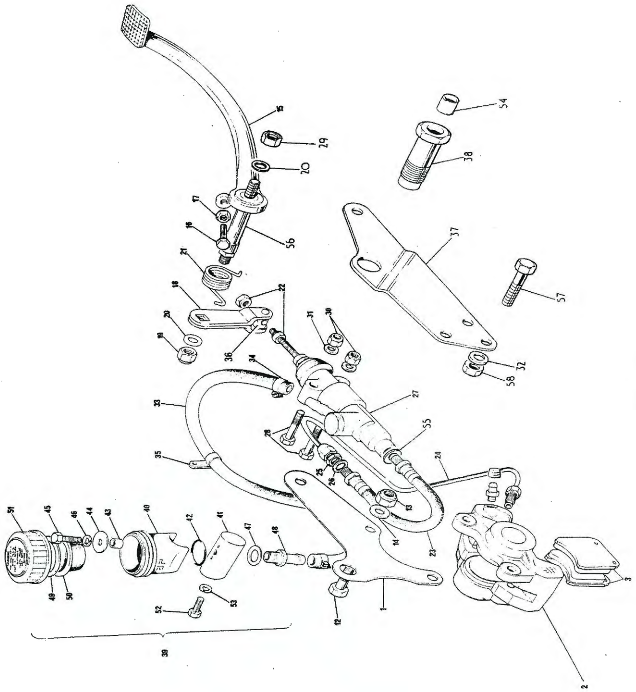
Fig. 25. REAR BRAKE
