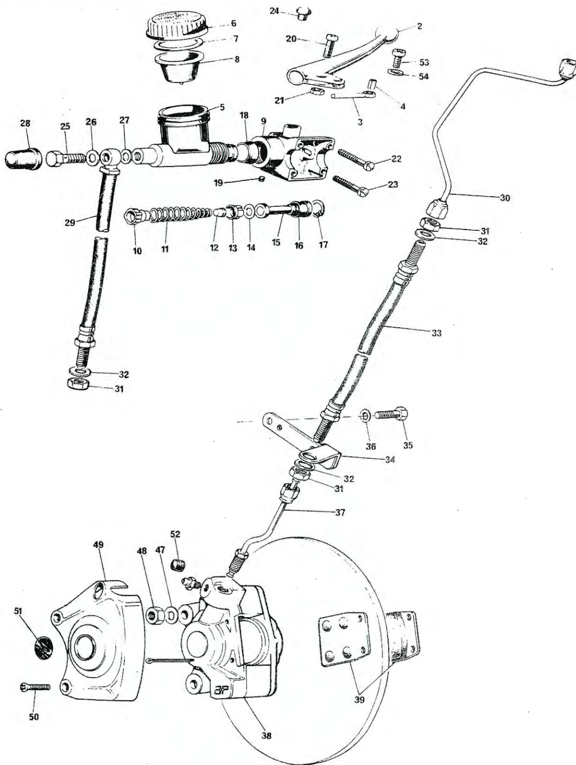
Fig. 23. FRONT BRAKE
