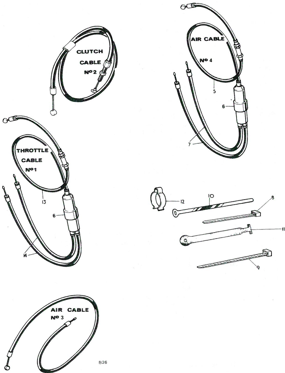
Fig. 30. CONTROL CABLES
