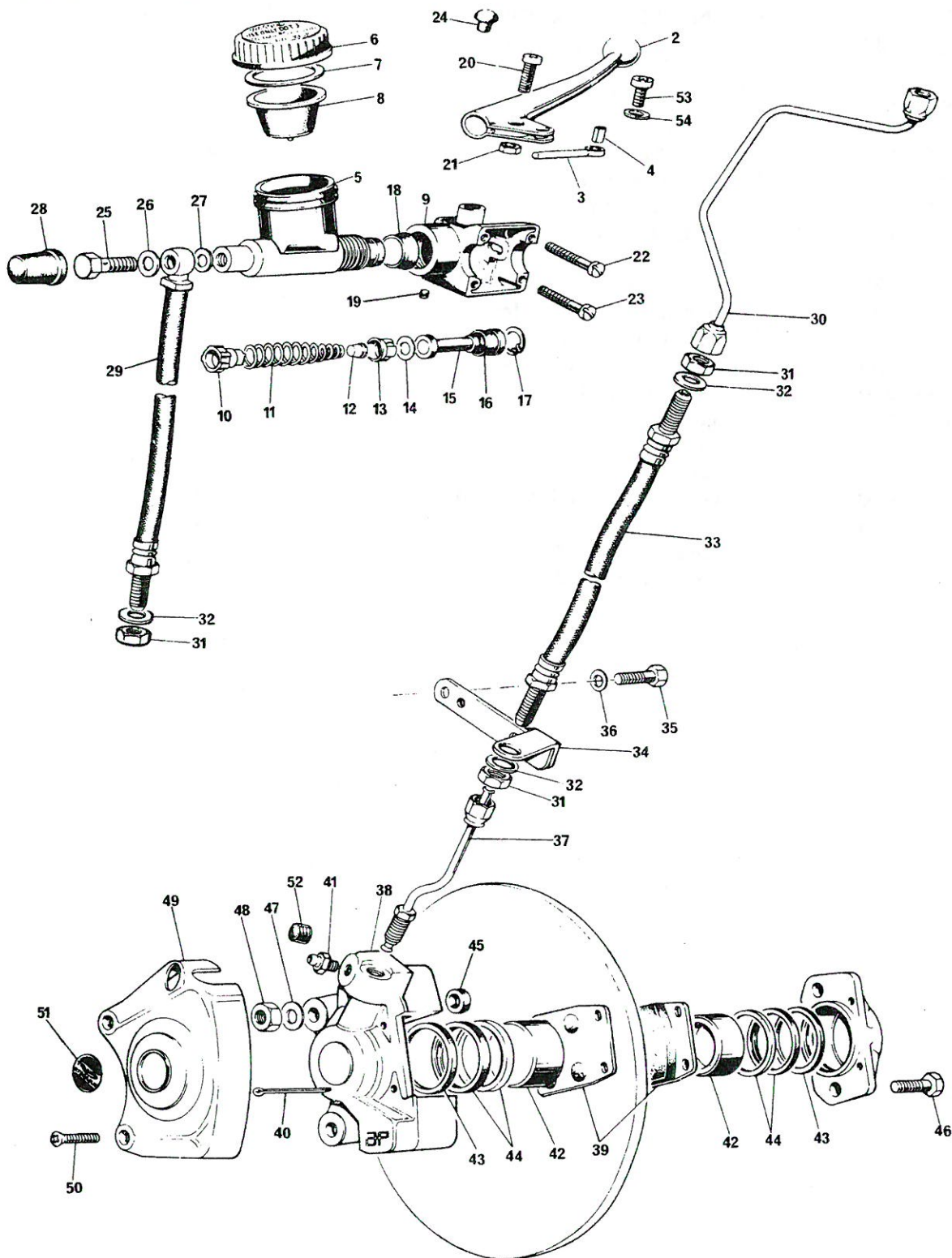
Fig. 23. FRONT BRAKE
