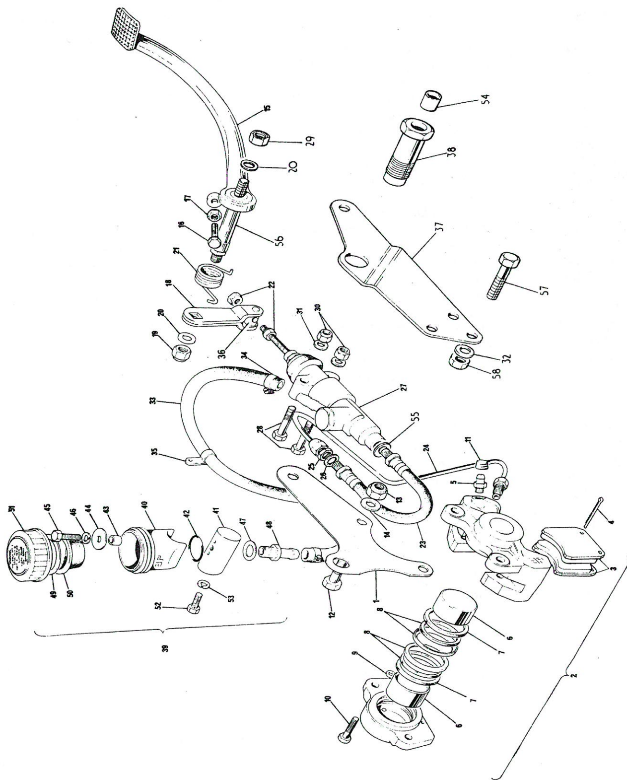
FIG. 25. REAR BRAKE
