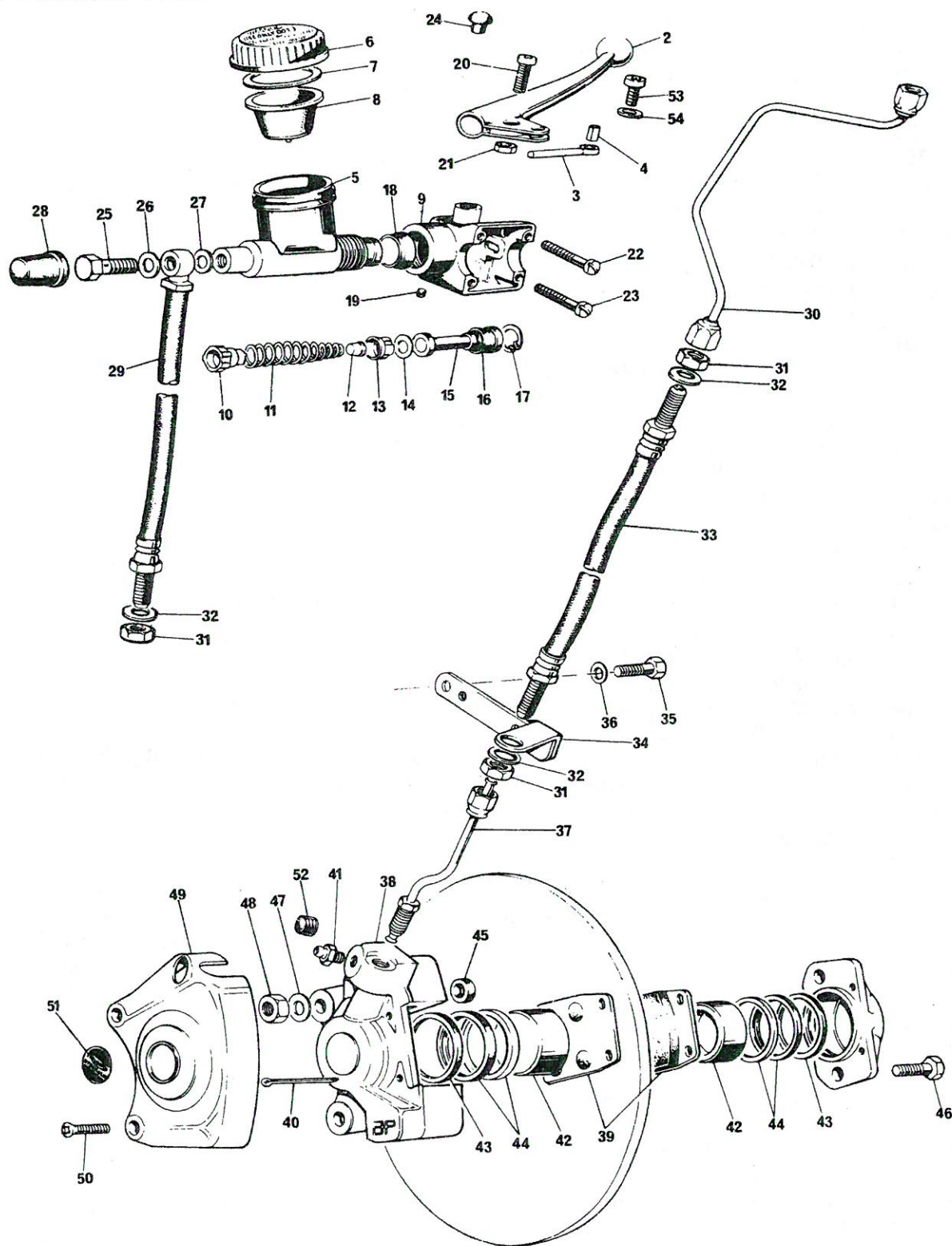
Fig. 23. FRONT BRAKE
