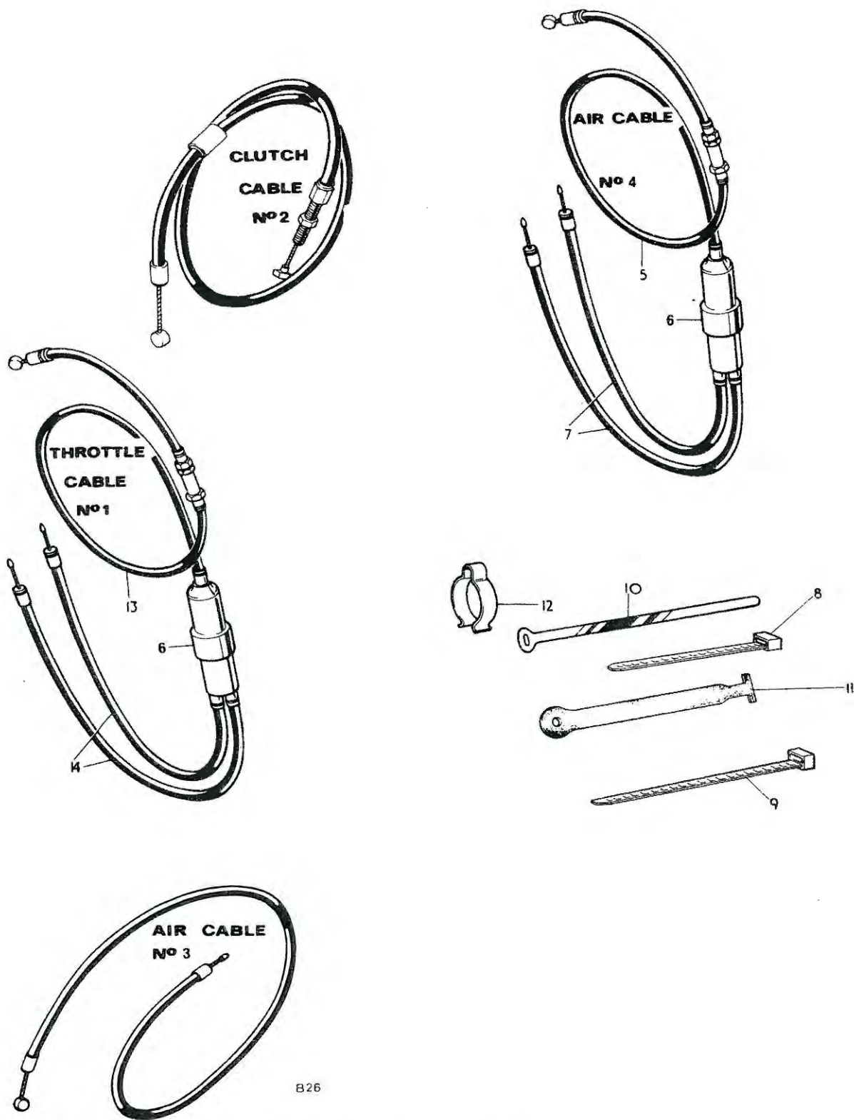
Fig. 30. CONTROL CABLES
