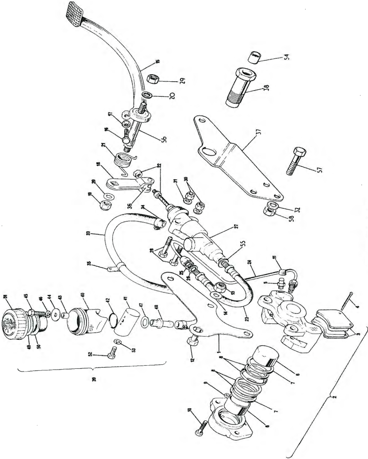
Fig. 25. REAR BRAKE
