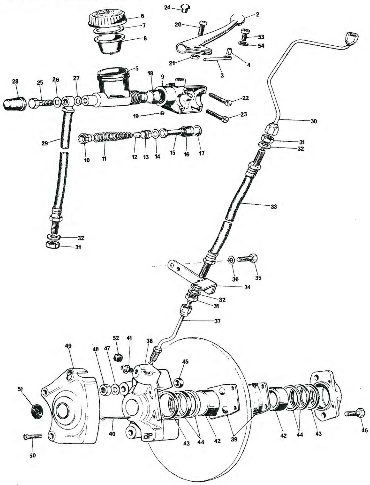
Fig. 23. FRONT BRAKE
