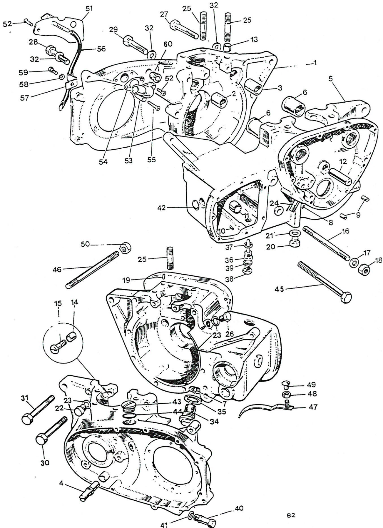
Fig. 2. CRANKCASE
