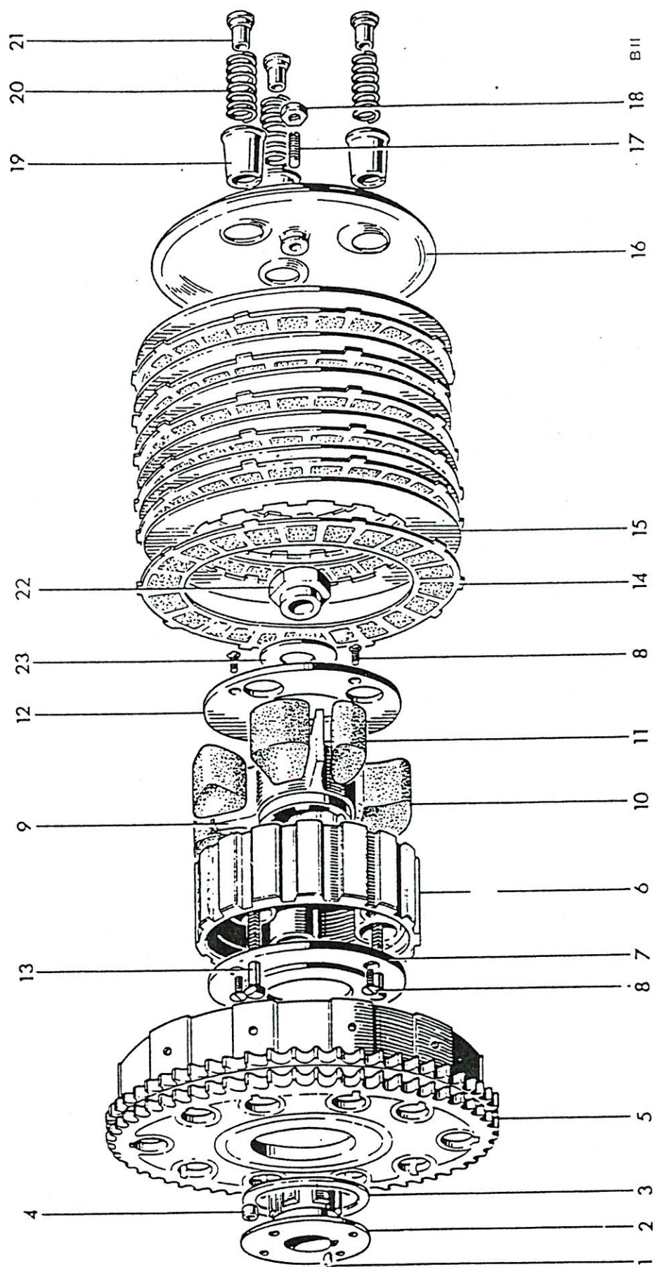
Fig. 12. CLUTCH
