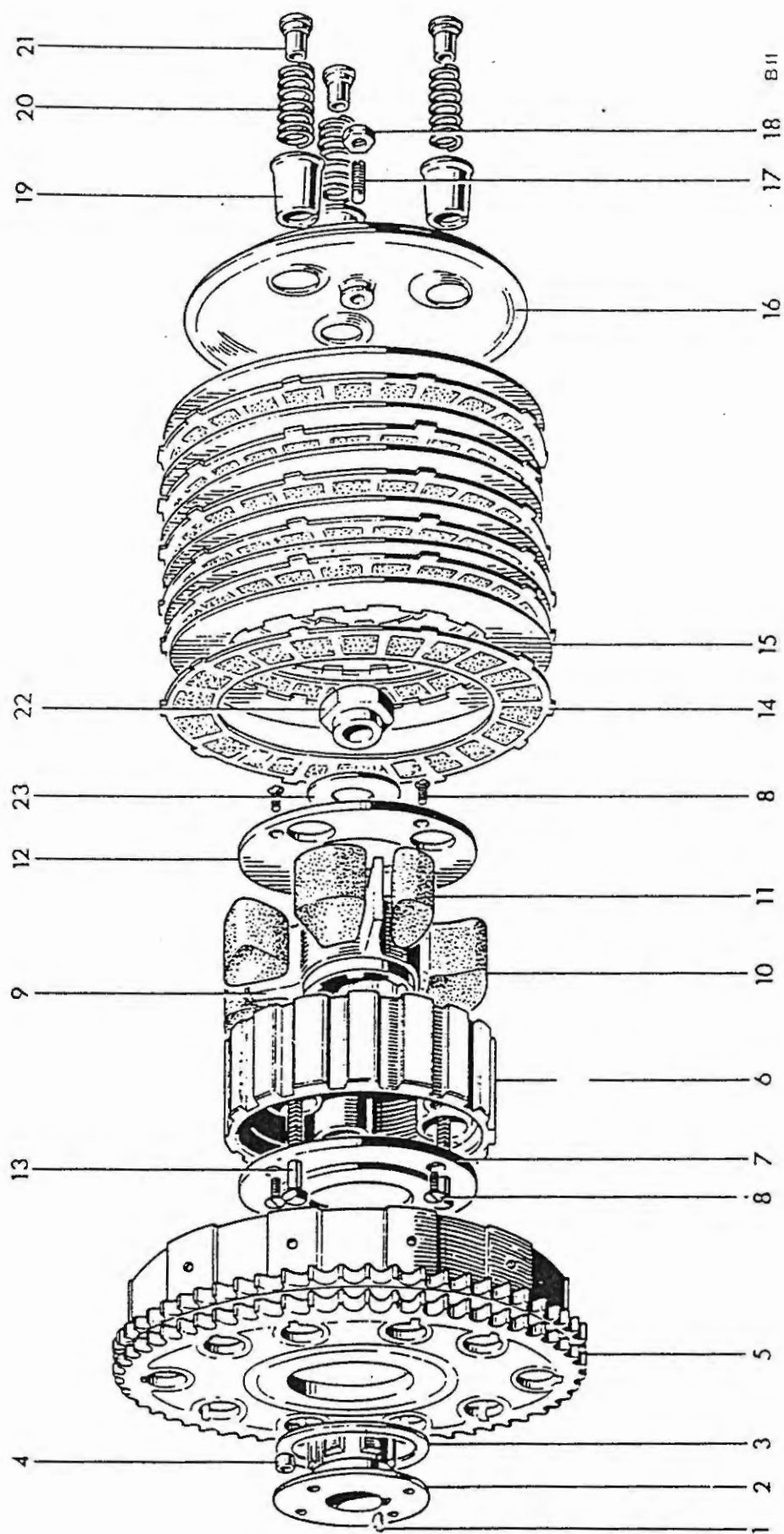
Fig. 12. CLUTCH
