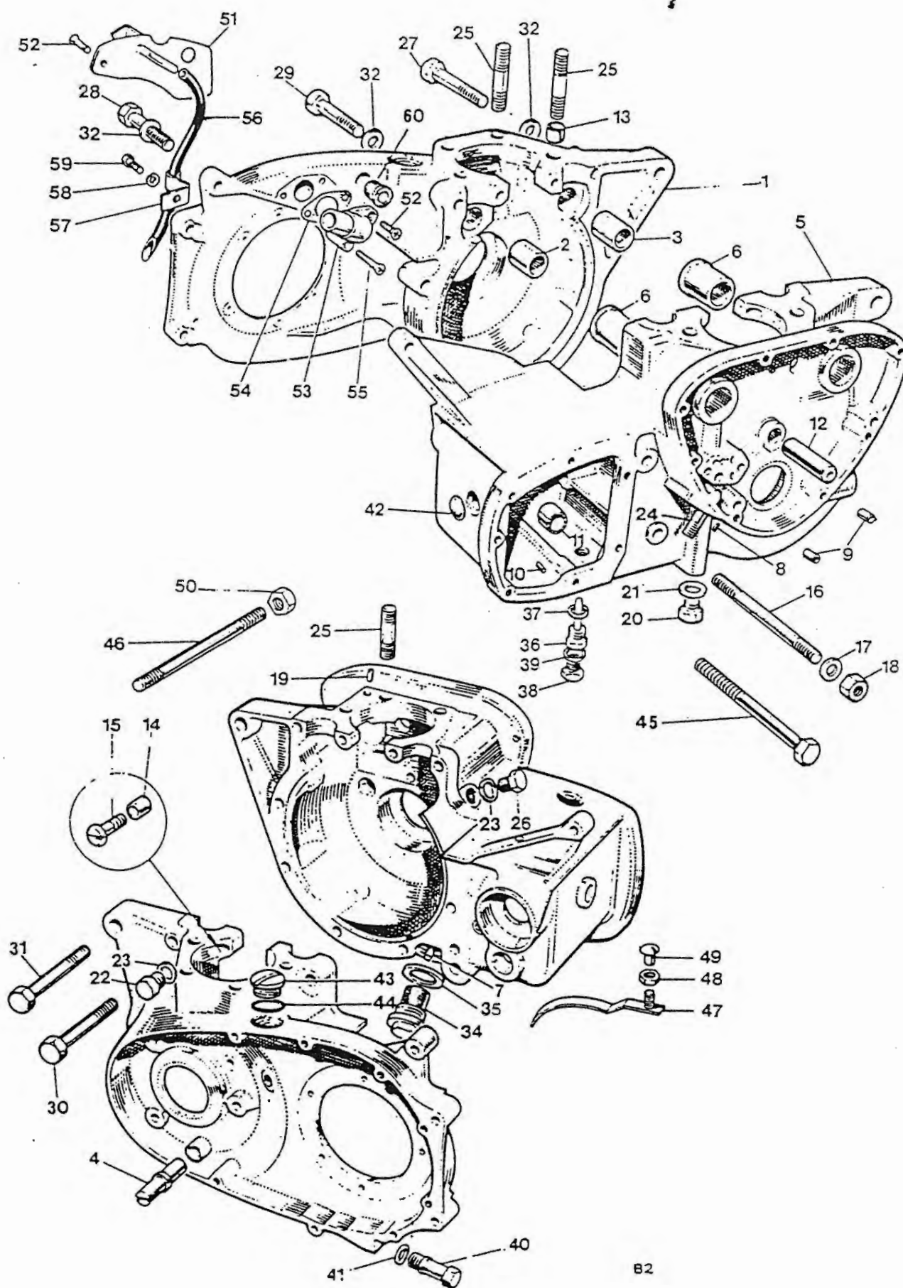
Fig. 2. CRANKCASE
