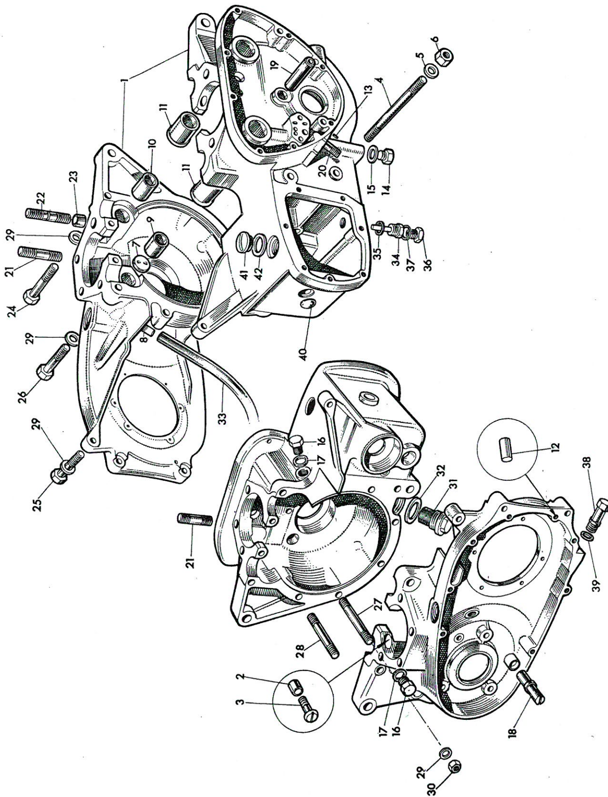
Fig. 2. CRANKCASE
