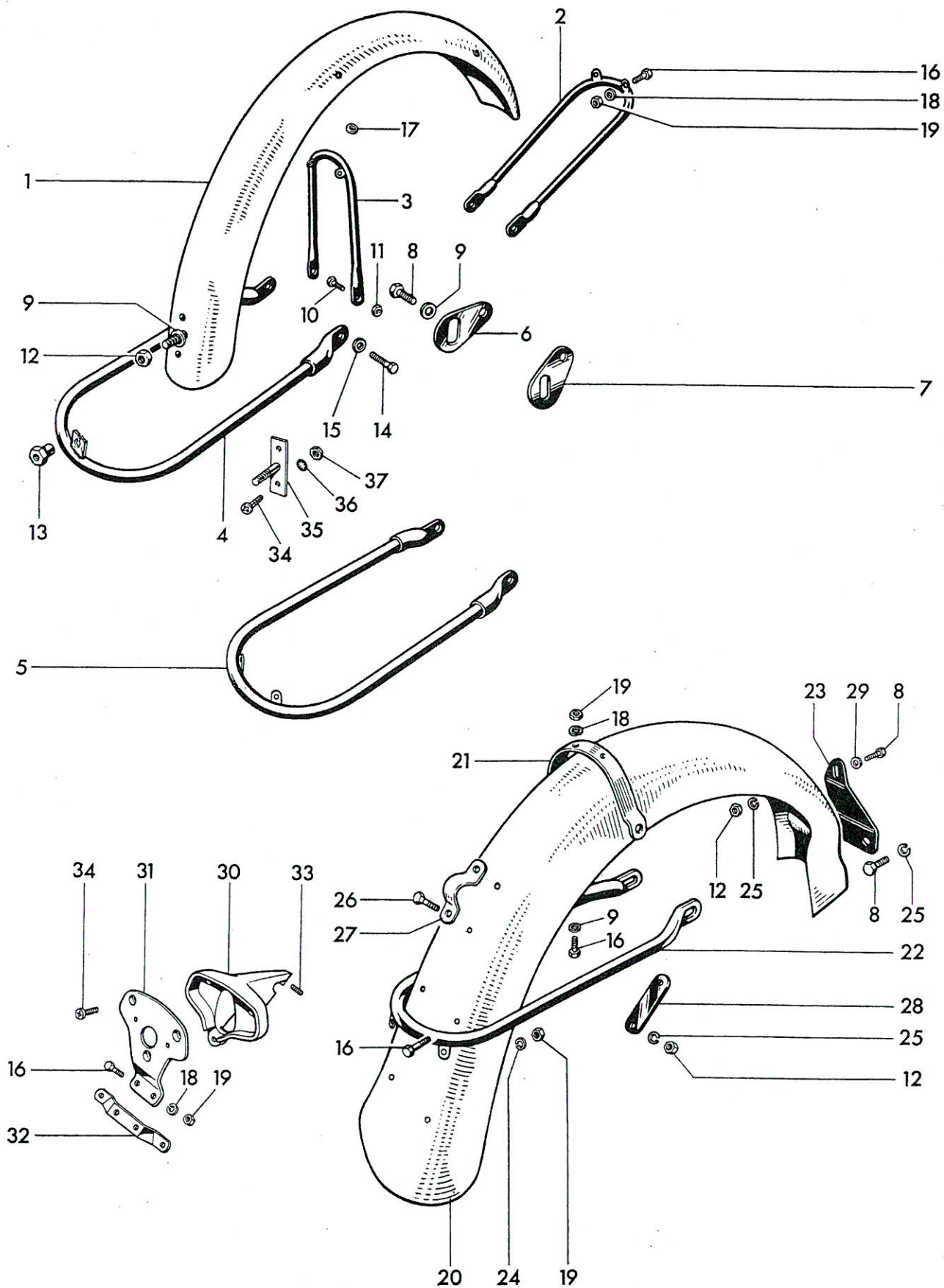
Fig. 30. FENDERS (U.S.A.)
