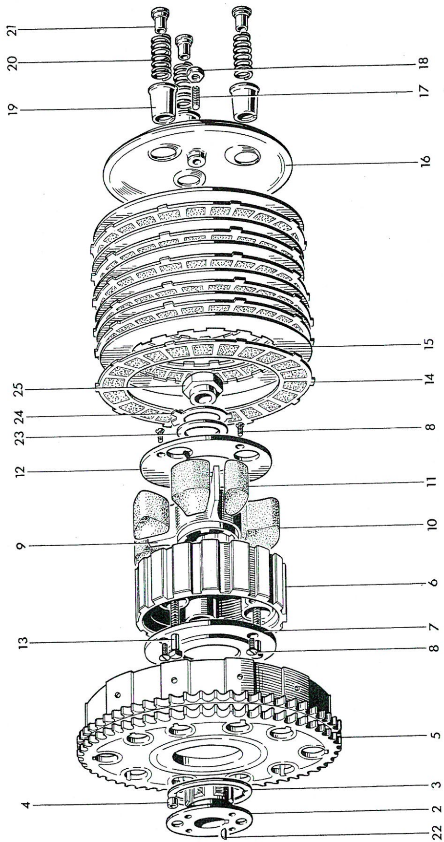
Fig. 10. CLUTCH
