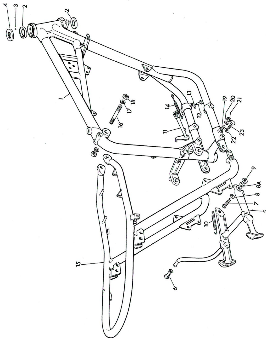
Fig. 12. FRAME
