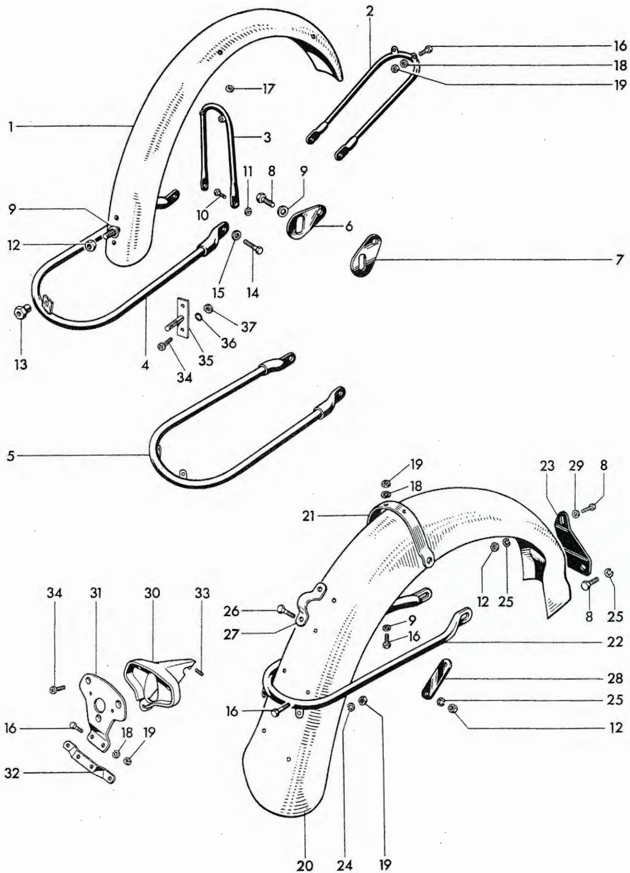
Fig. 30. FENDERS (U.S.A.)
