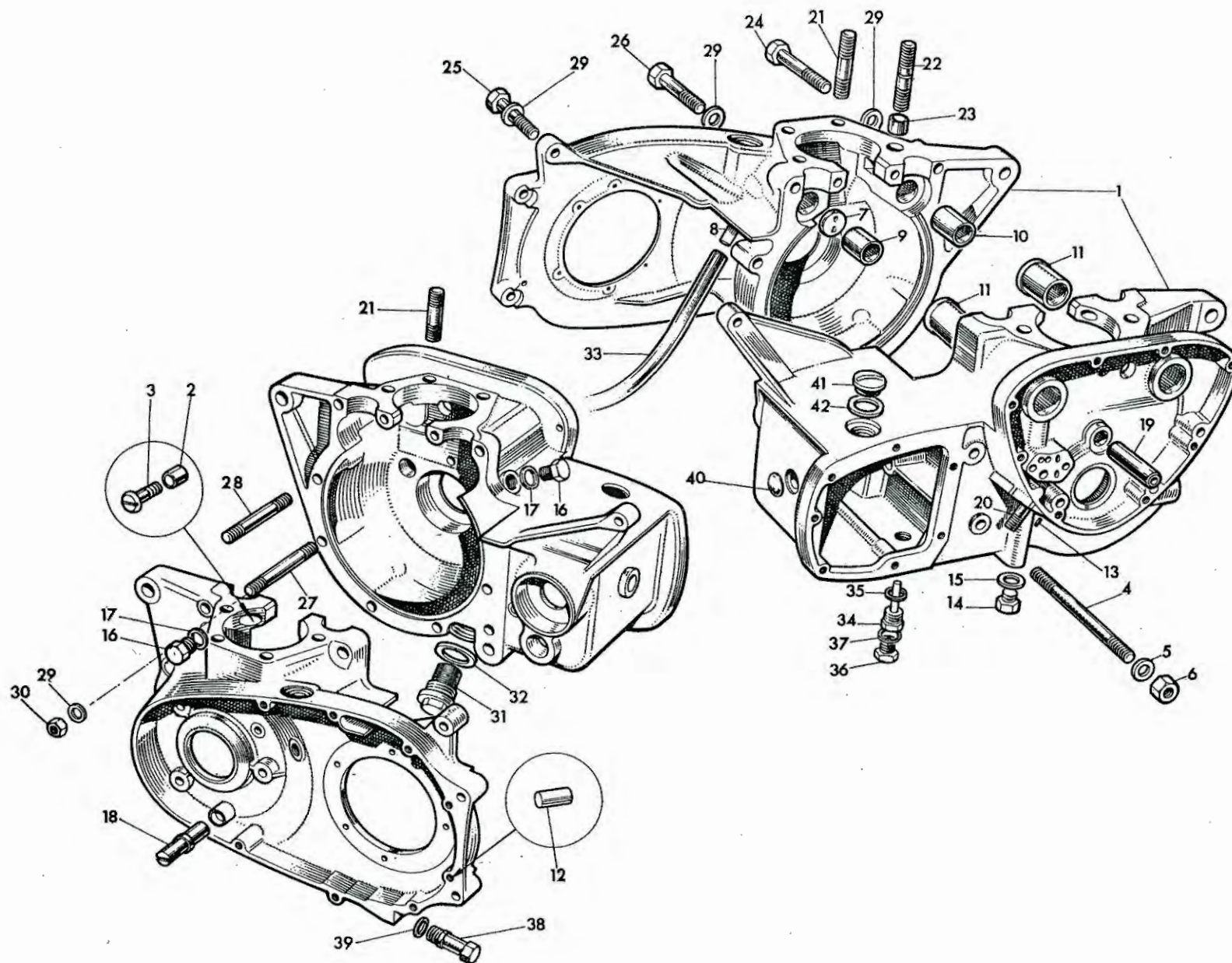
Fig. 2. CRANKCASE
