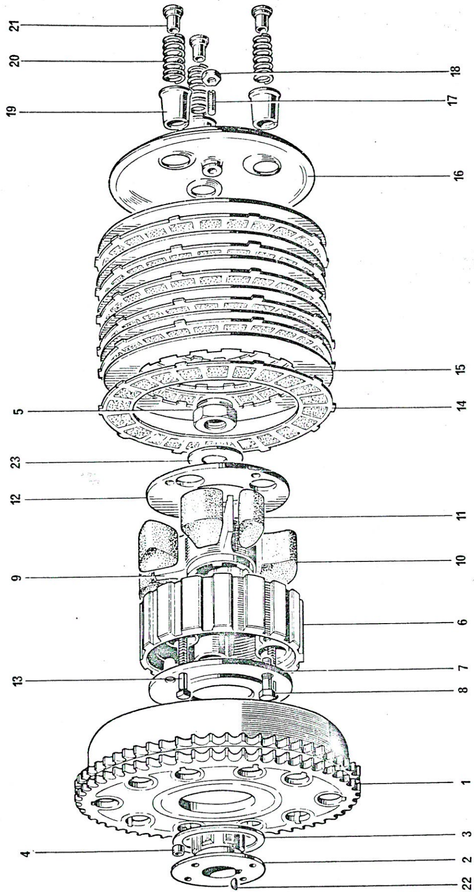
Fig. 10. CLUTCH
