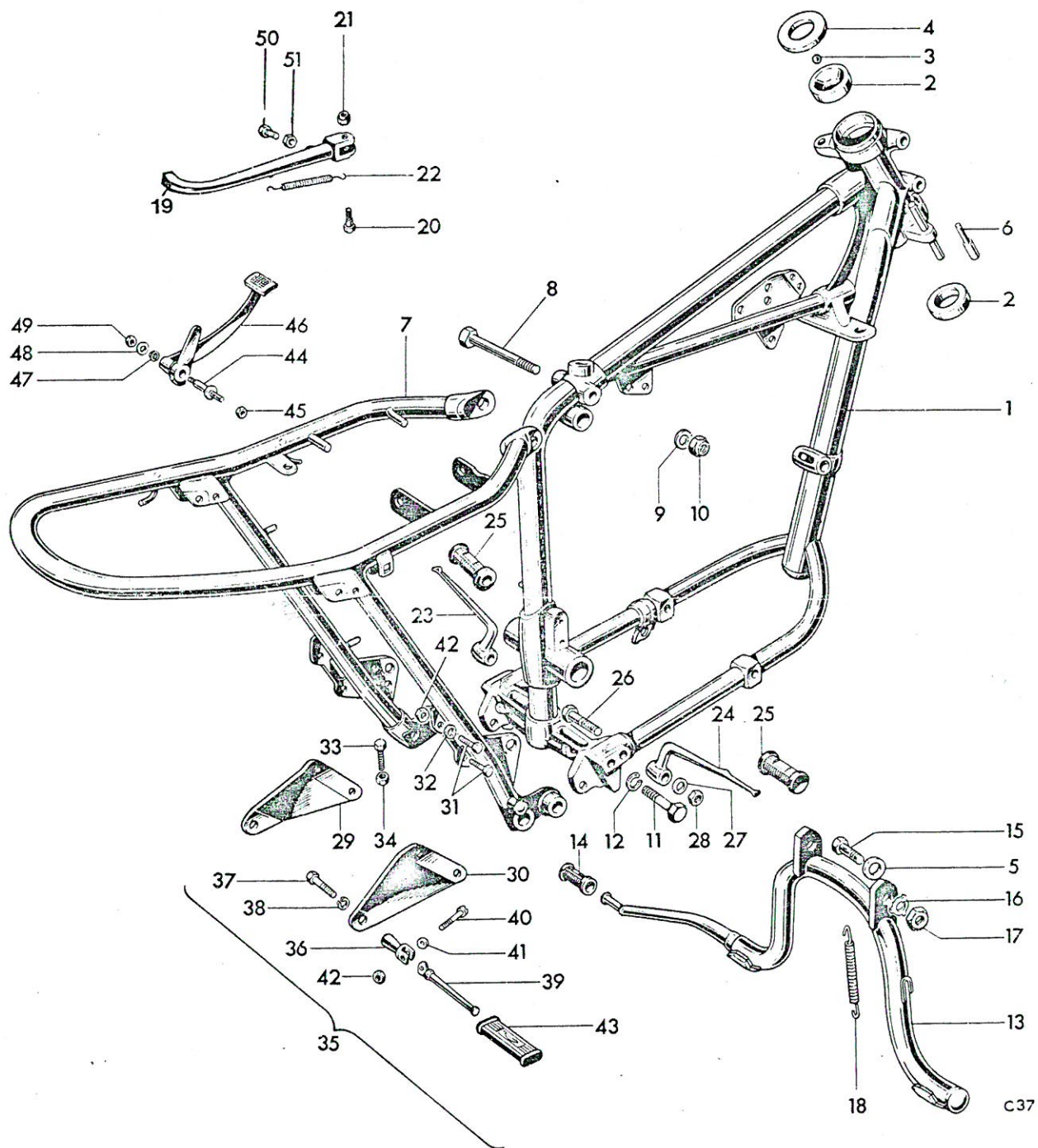
Fig. 14. FRAME
