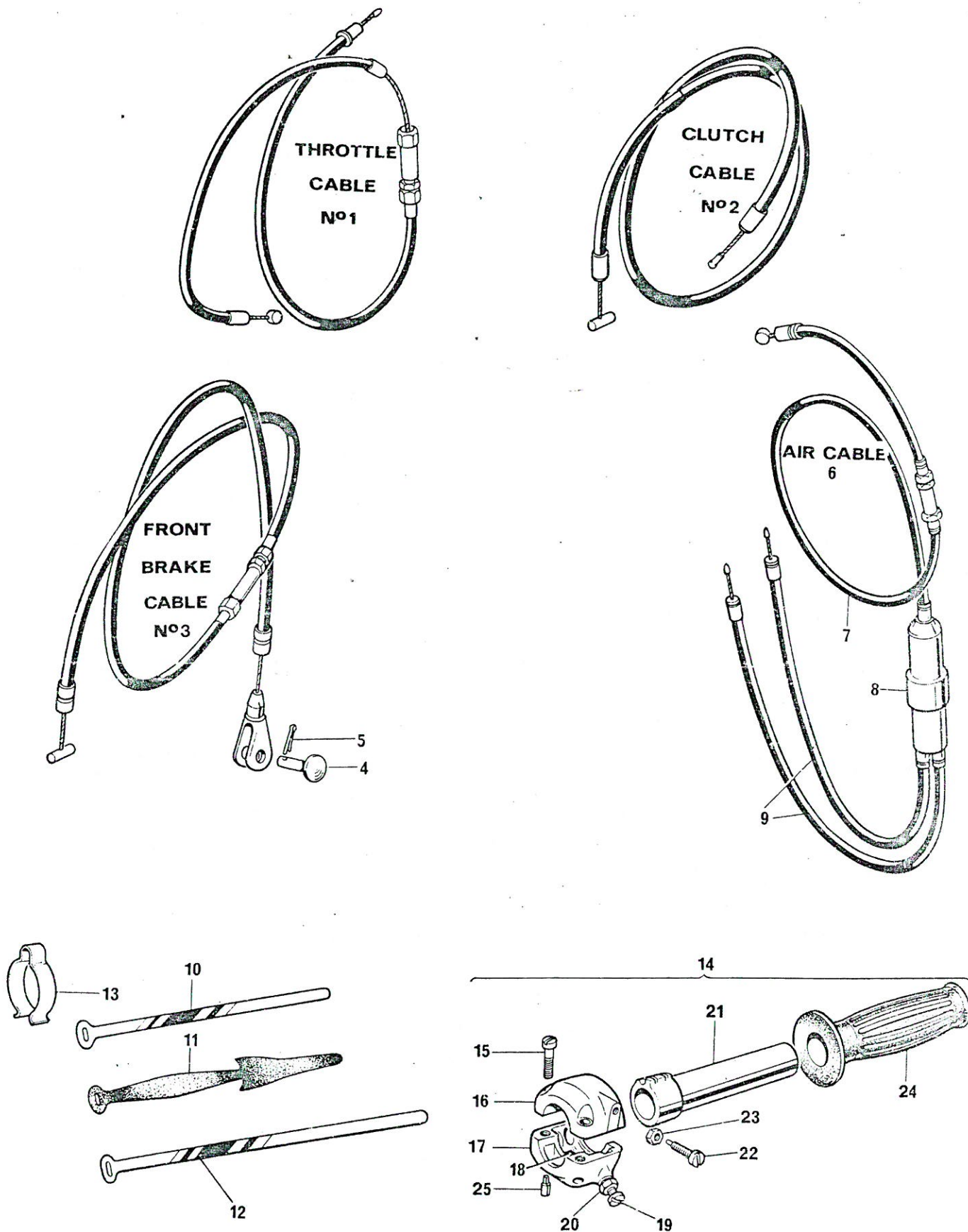
Fig. 26. CONTROL CABLES
