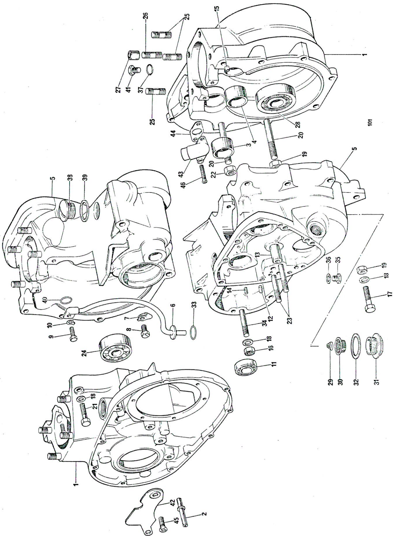
Fig. 2. CRANKCASE
