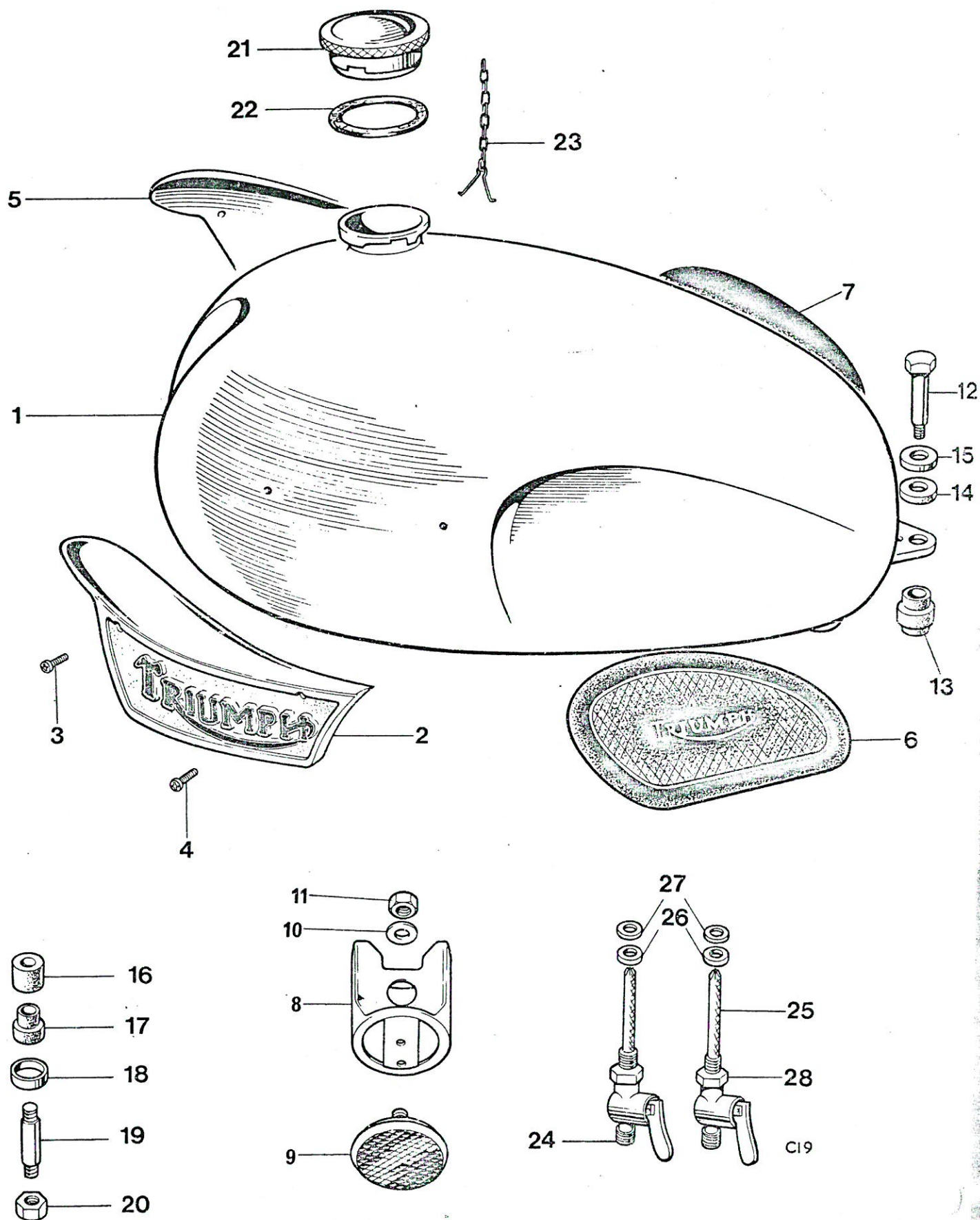
Fig. 22. GAS TANK
