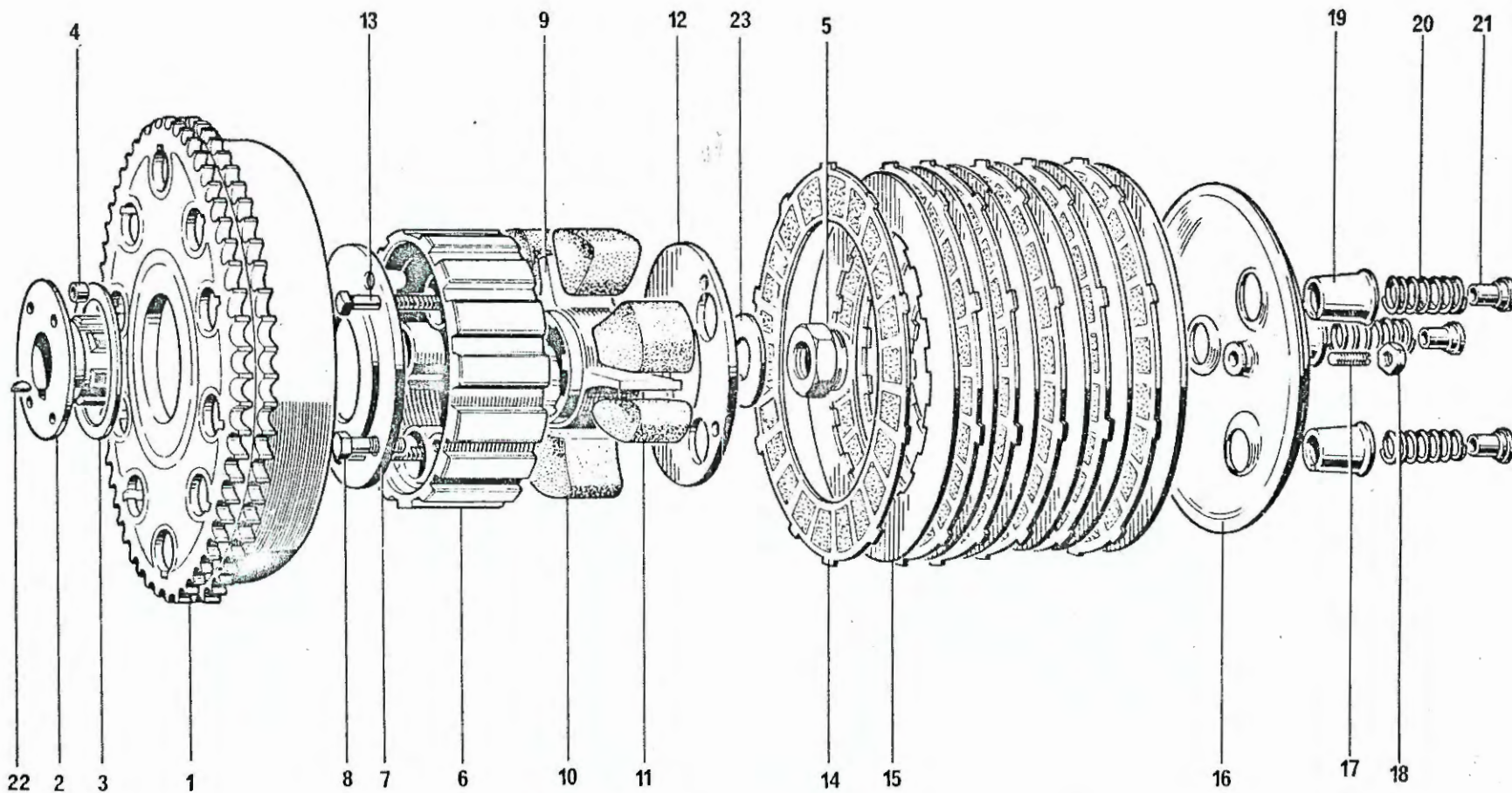
Fig. 10. CLUTCH
