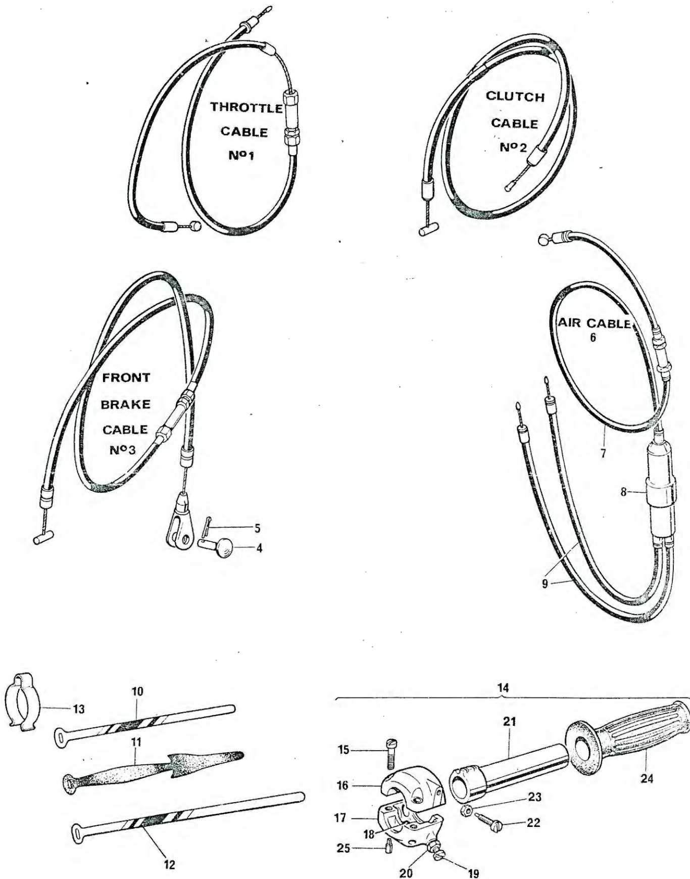
Fig. 26. CONTROL CABLES
