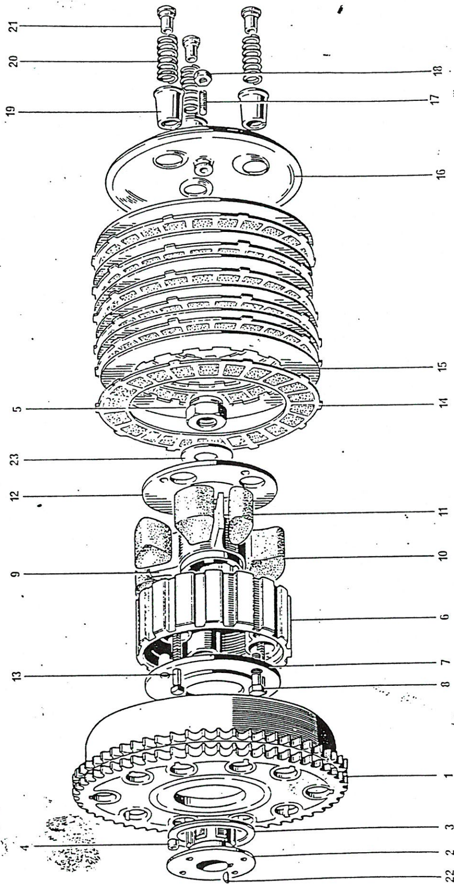
Fig. 13. CLUTCH
