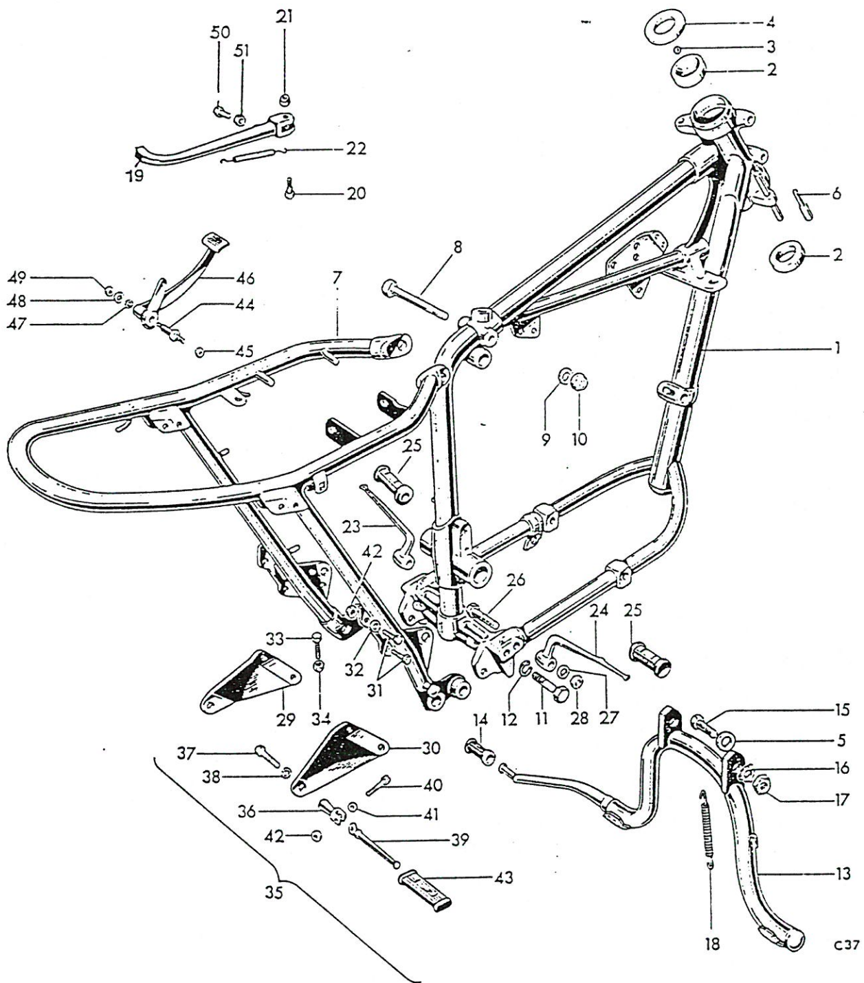
Fig. 18. FRAME
