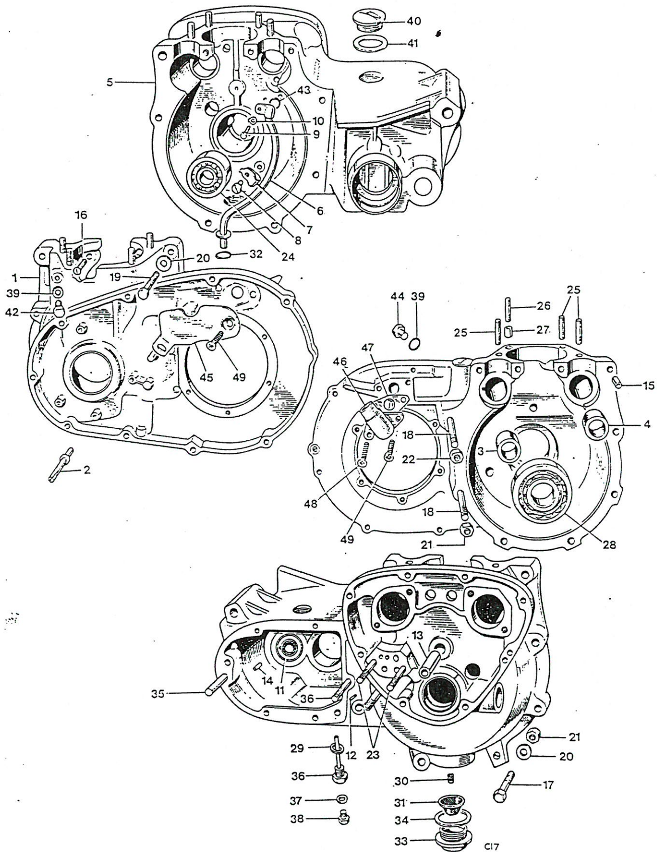
Fig. 2. CRANKCASE
