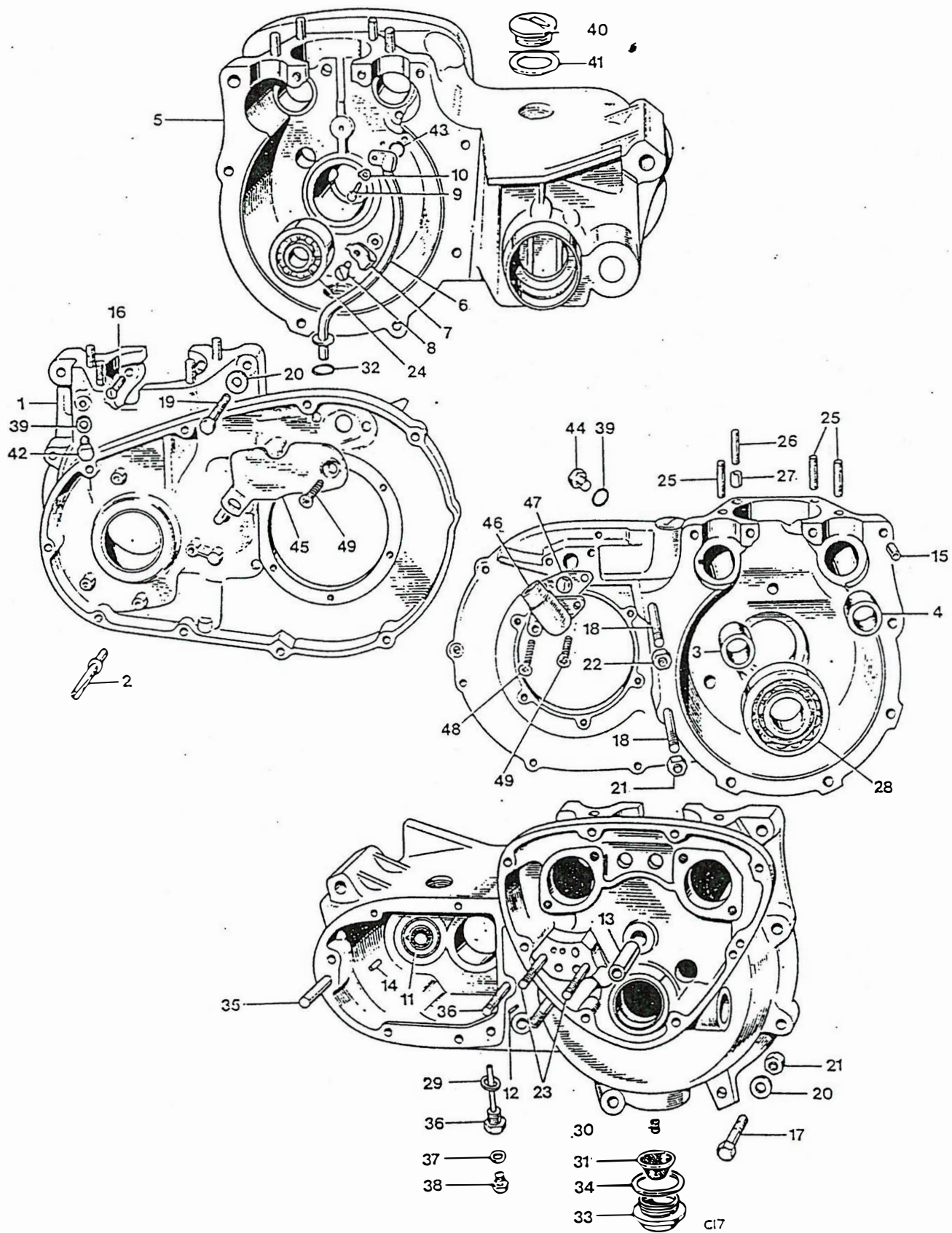
Fig. 2. CRANKCASE
