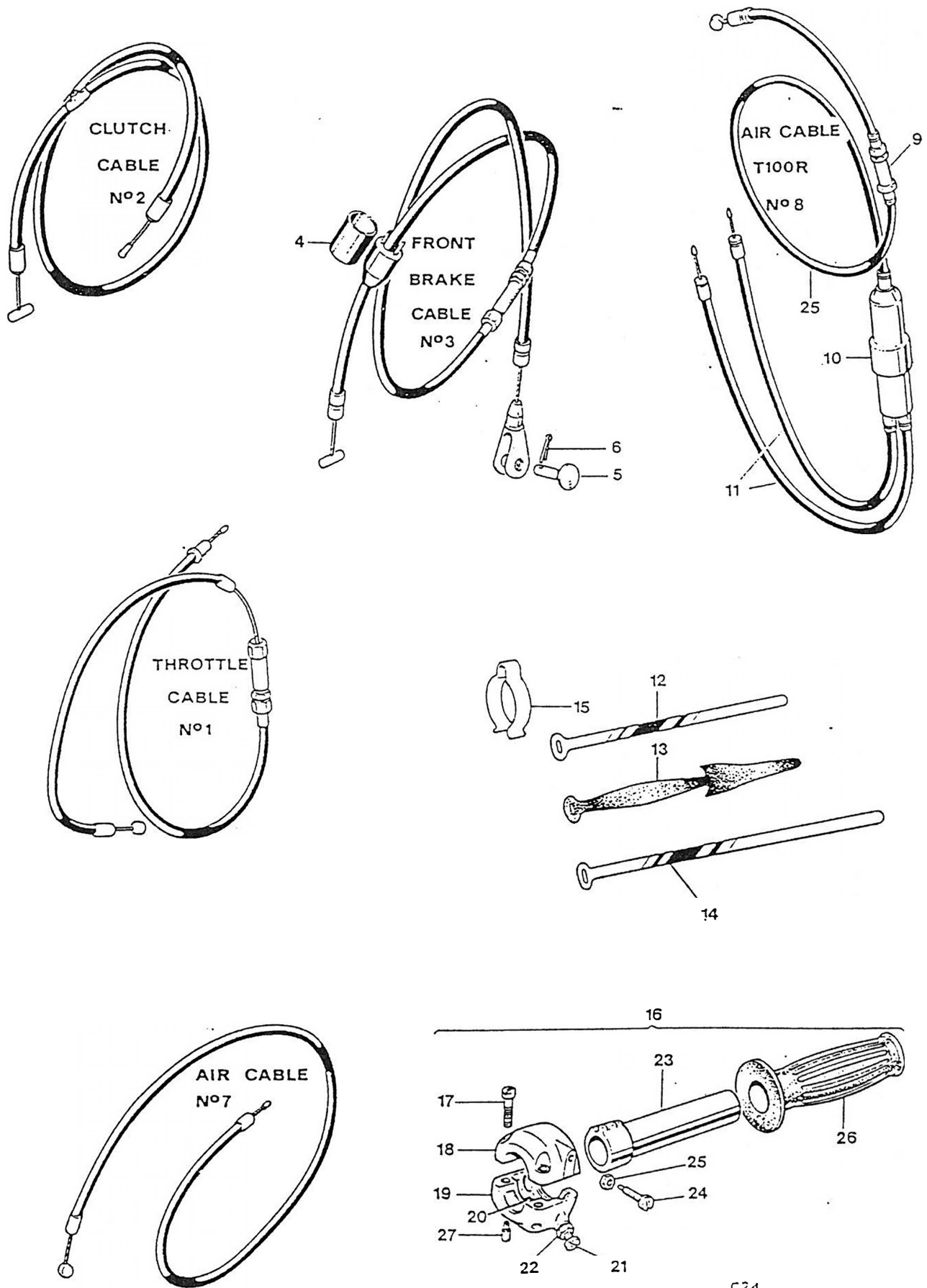
Fig. 31. CONTROL CABLES
