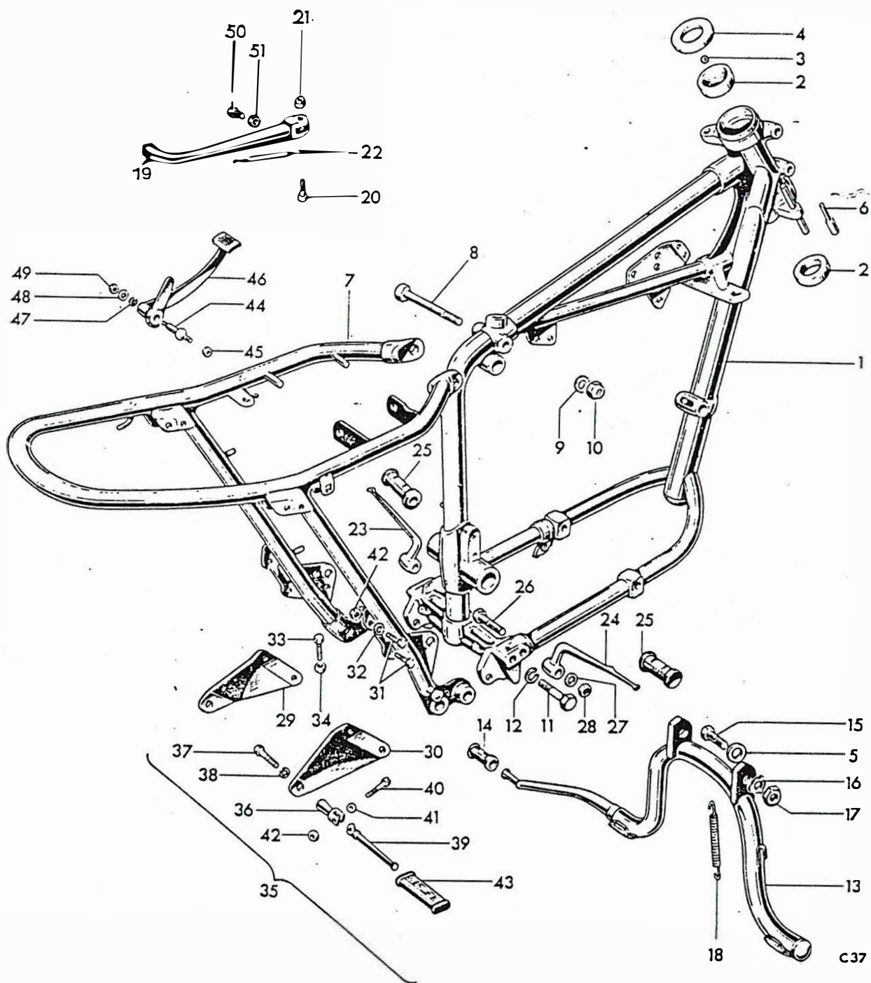
Fig. 18. FRAME
