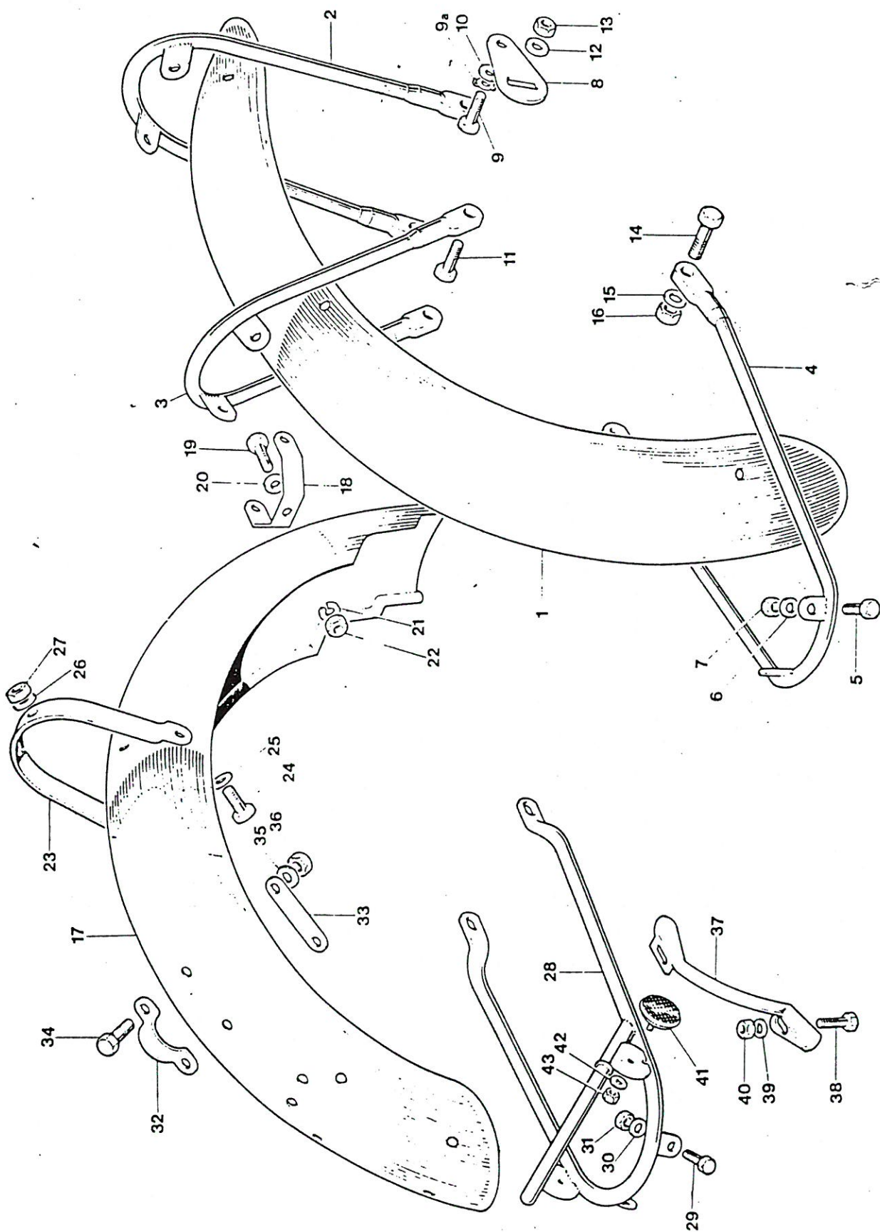
Fig. 24. FENDERS
