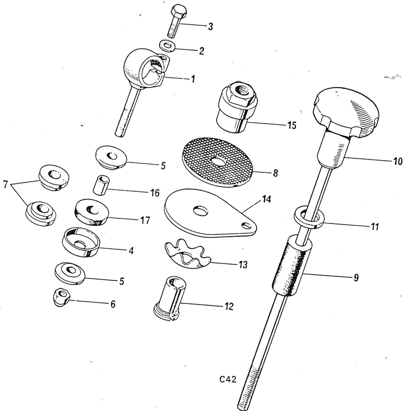
Fig. 30. STEERING DAMPER
