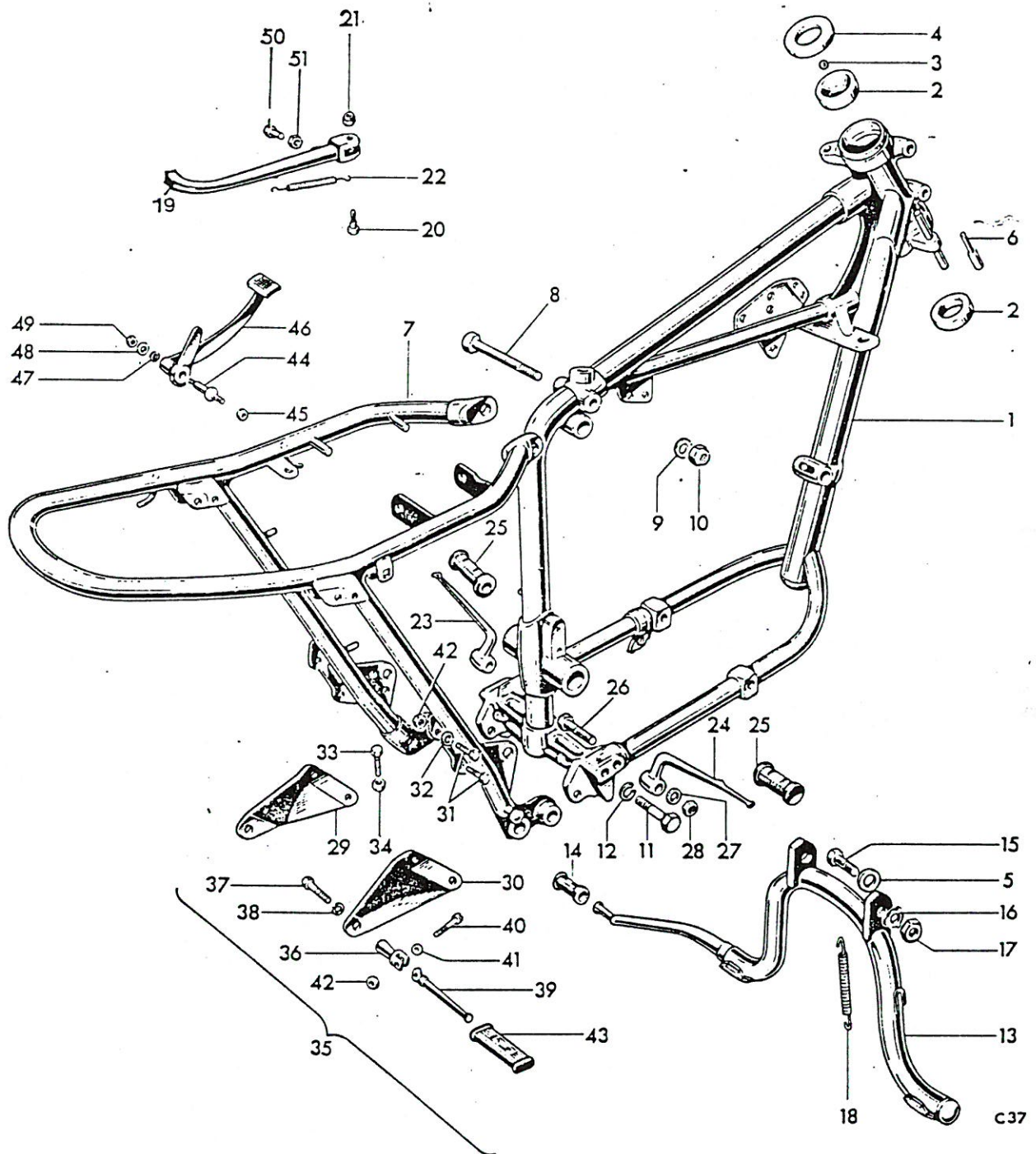
Fig. 18. FRAME
