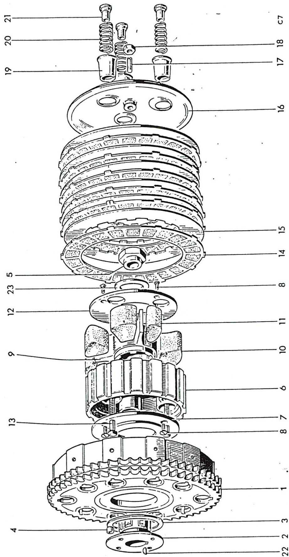
Fig. 13. CLUTCH
