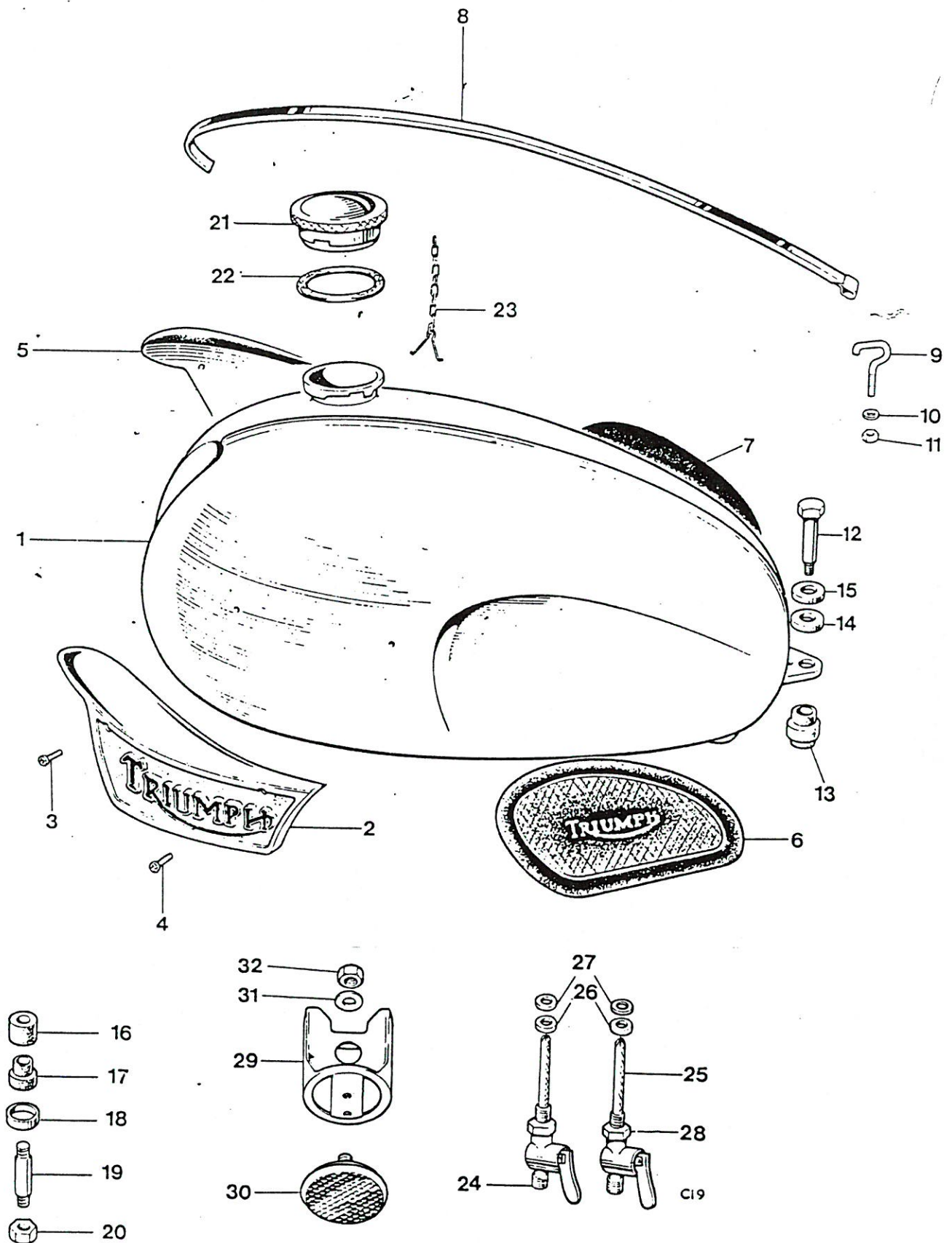
Fig. 27. GAS TANK
