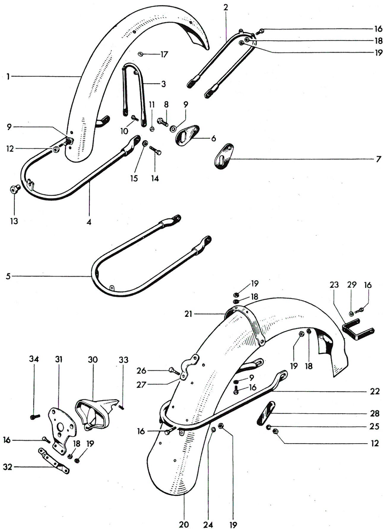
Fig. 23. FENDERS (U.S.A.)
