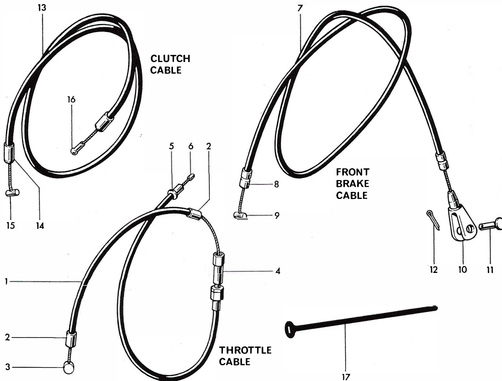
Fig. 29. CONTROL CABLES
