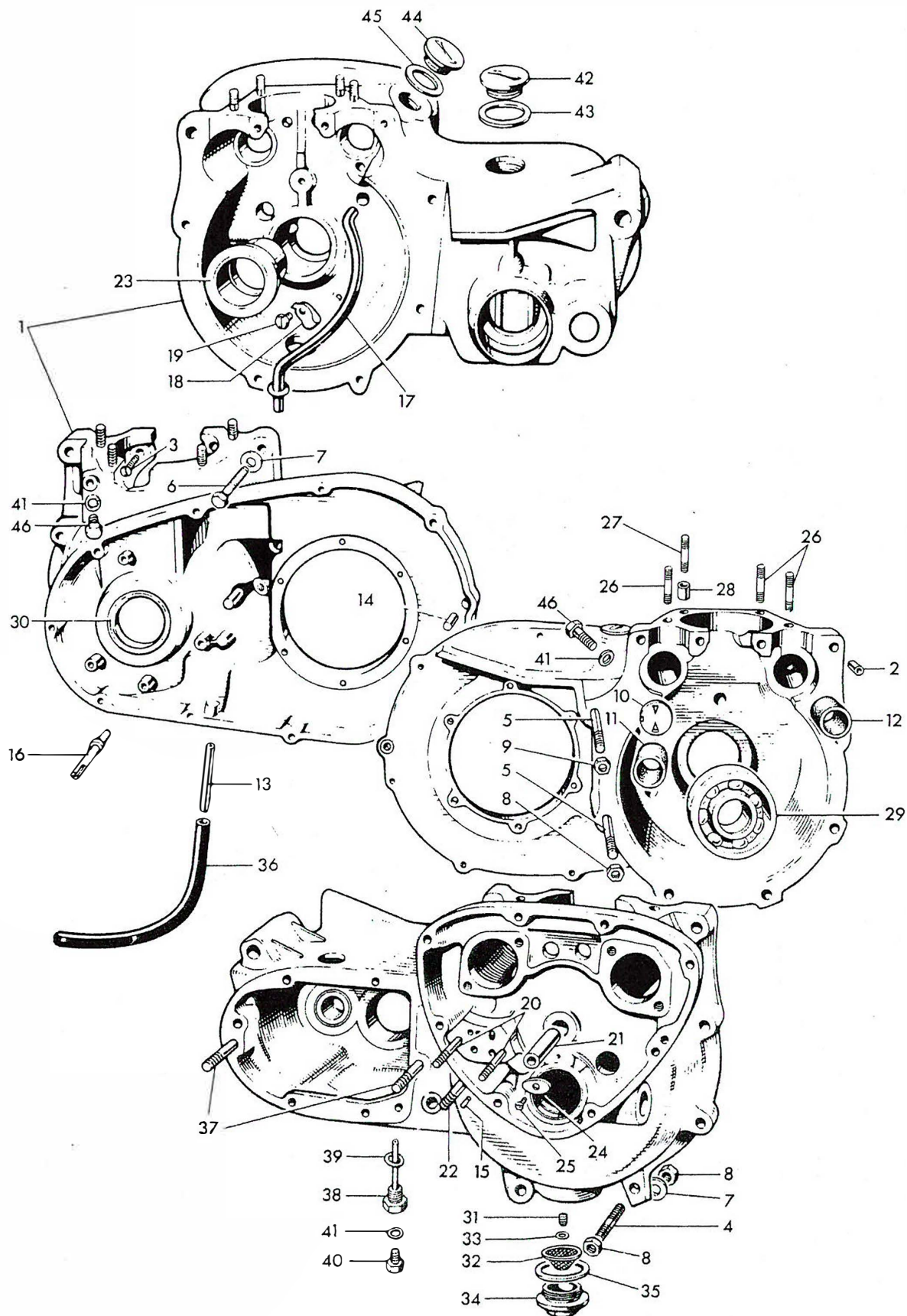
Fig. 2. CRANKCASE
