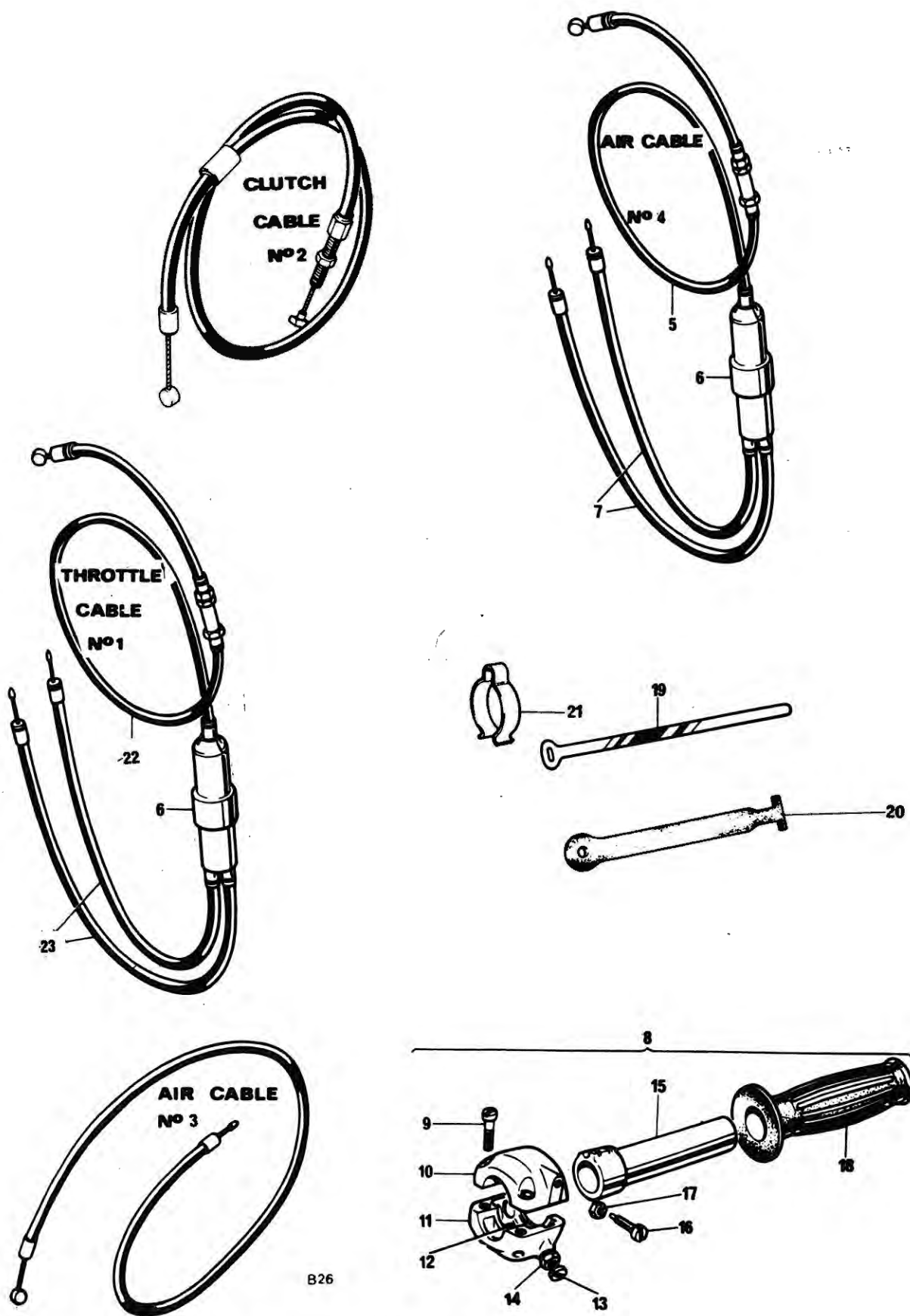
Fig. 30. CONTROL CABLES
