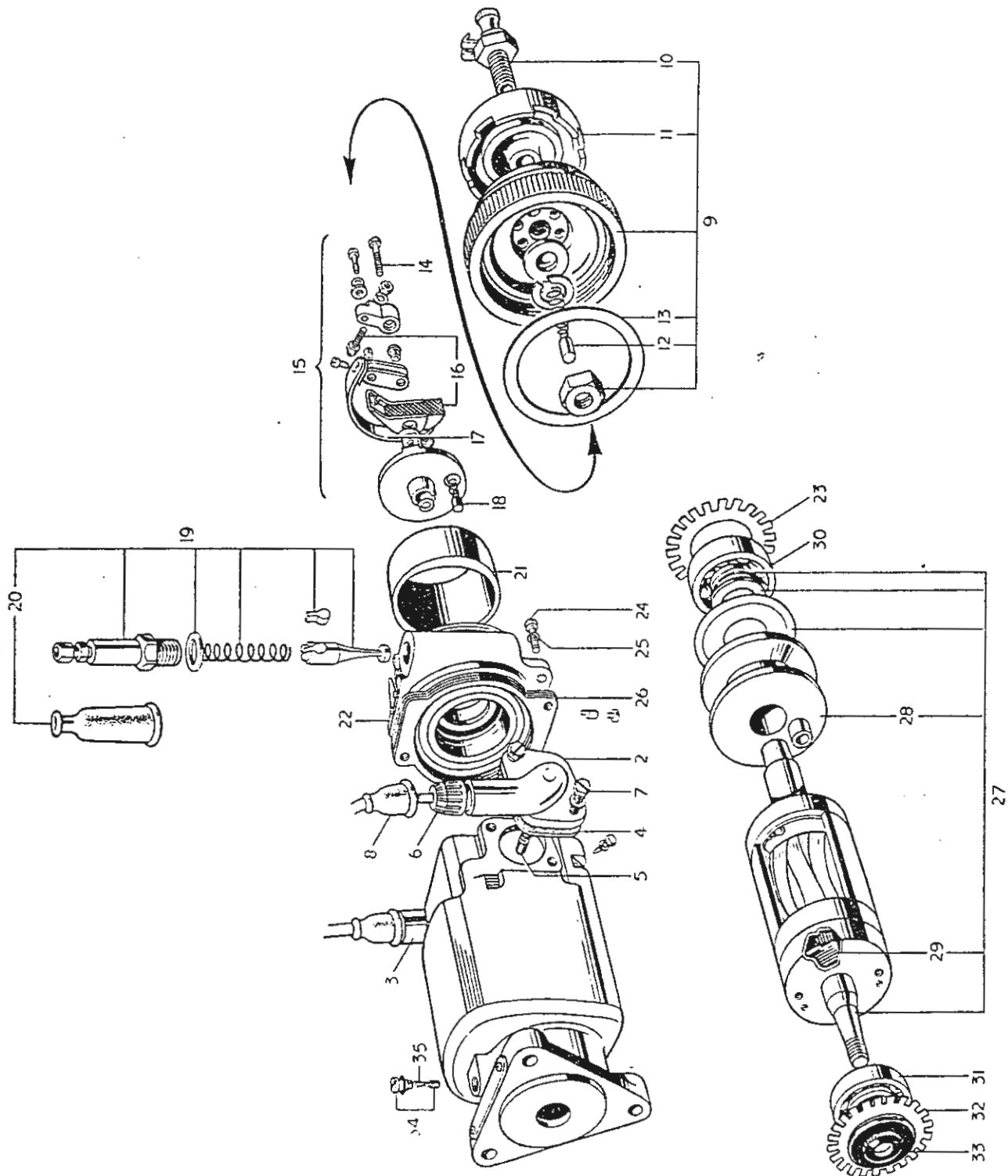
FIG. 32. LUCAS MAGNETO
