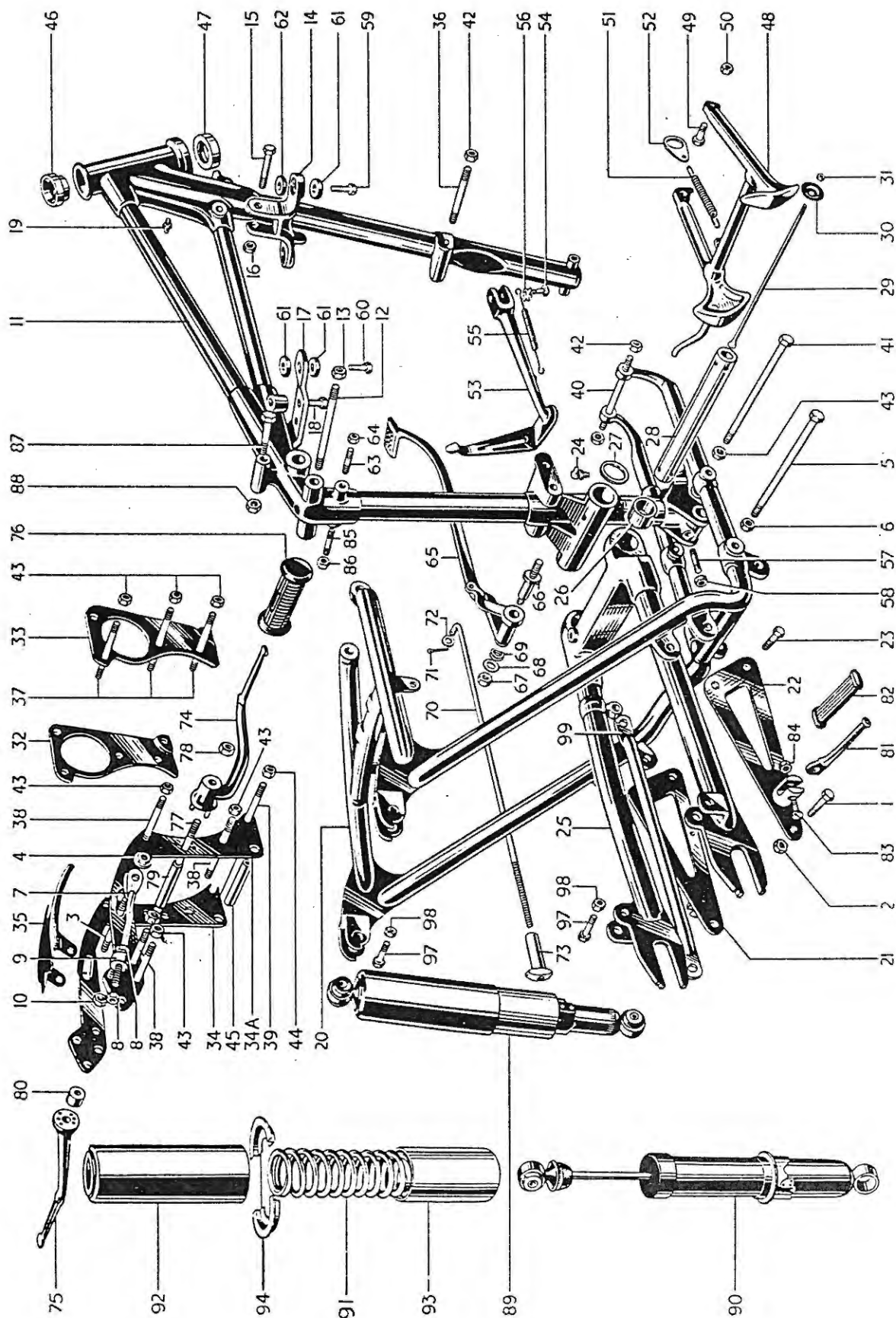
FIG. 13. FRAME
