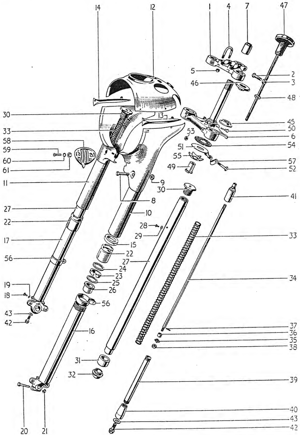
FIG. 15. TELESCOPIC FORK
