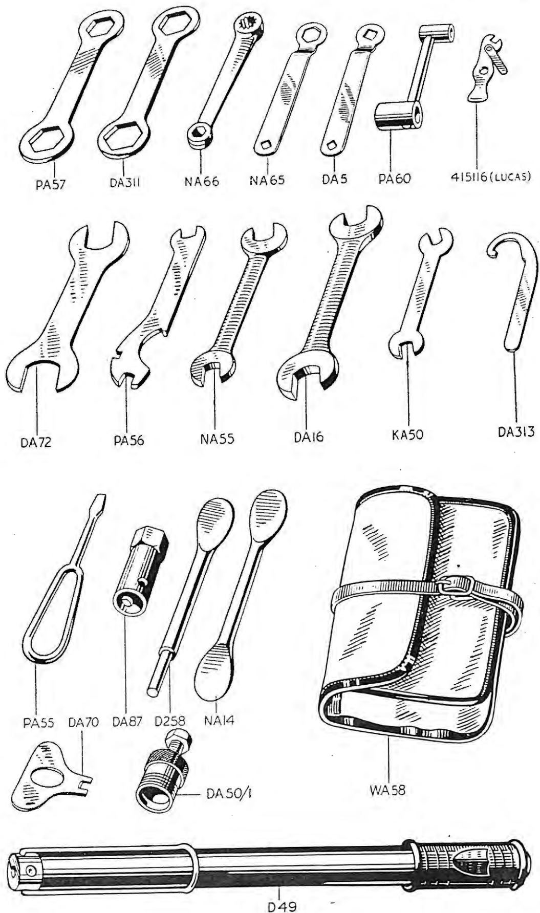
FIG. 27. TOOL KIT
