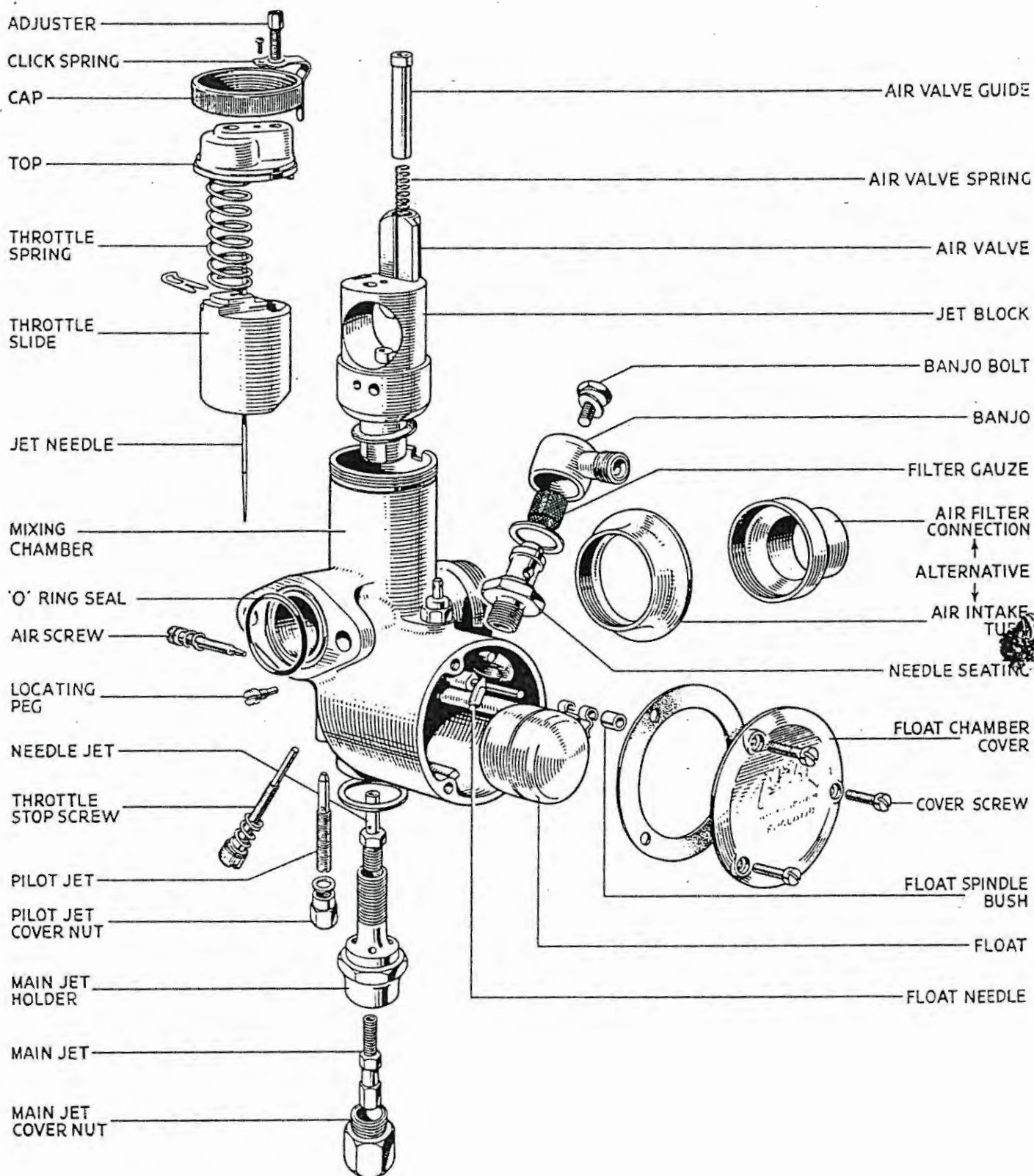
FIG. 29. AMAL CARBURETTER
