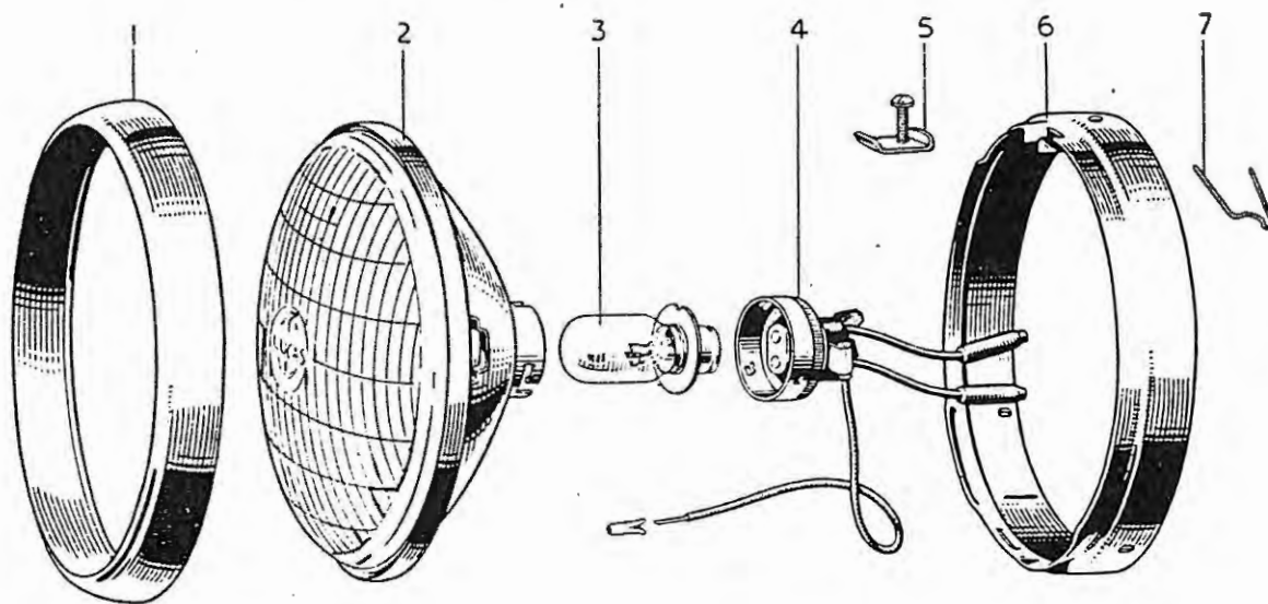
FIG. 31. HEAD LAMP
