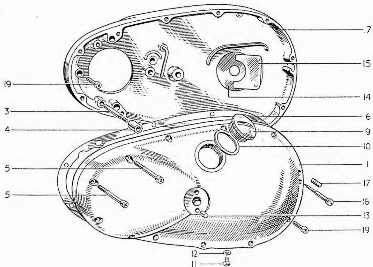
FIG. 24. PRIMARY CHAINCASE
