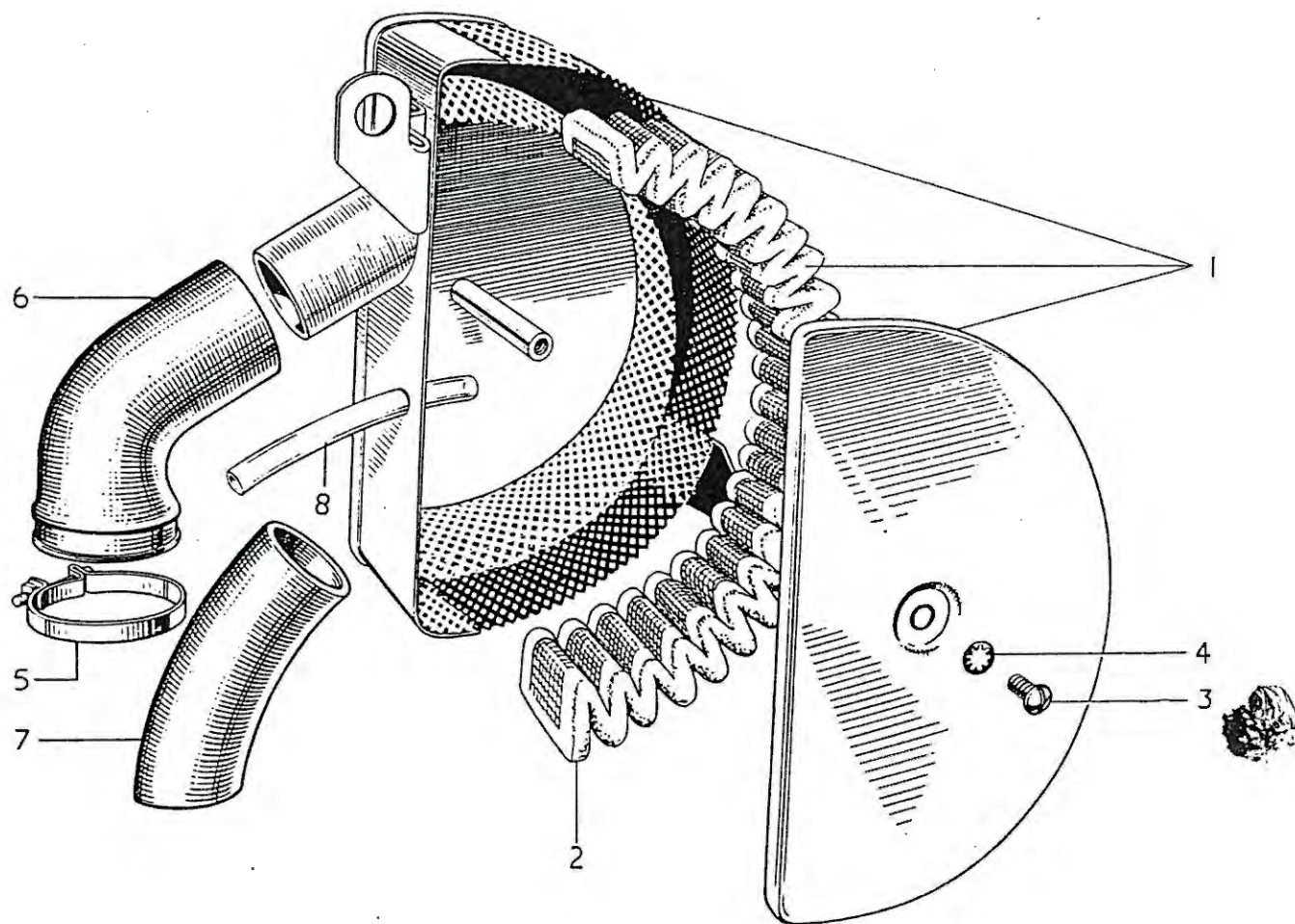
FIG. 28. AIR FILTER
