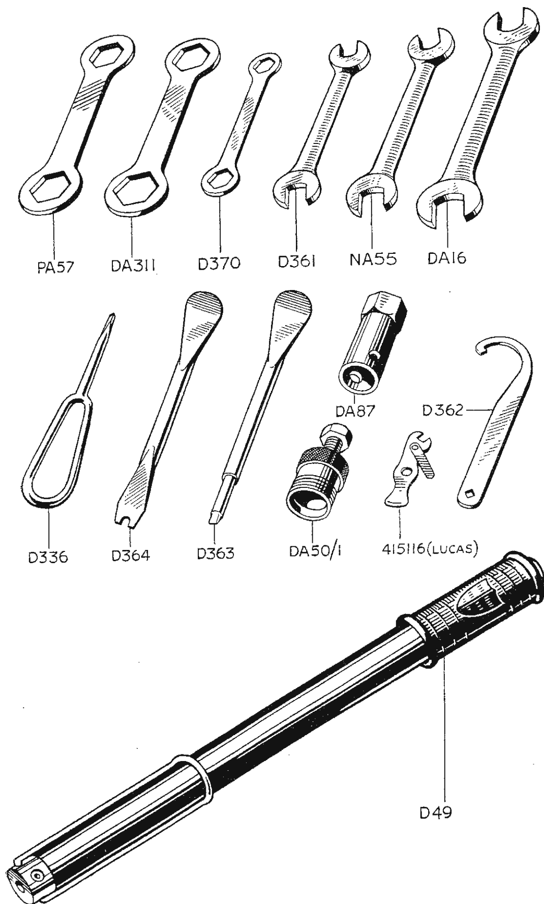
FIG. 27. TOOL KIT
