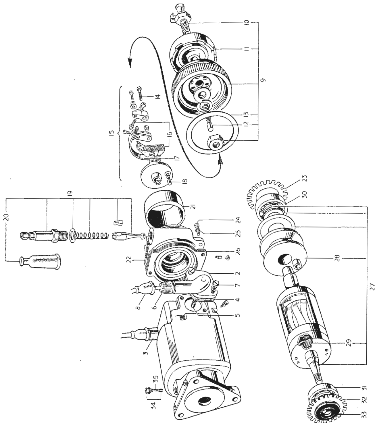
FIG. 32. LUCAS MAGNETO
