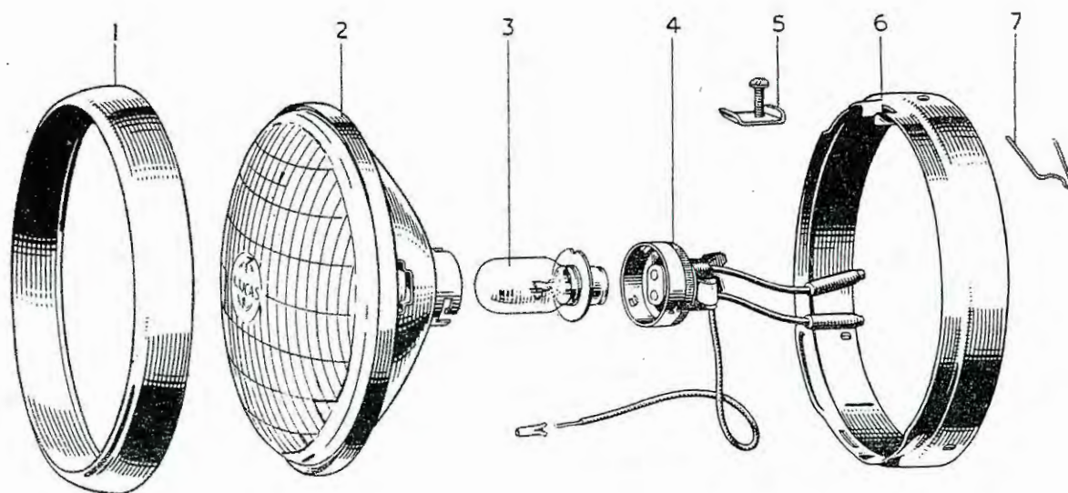
FIG. 31. HEAD LAMP
