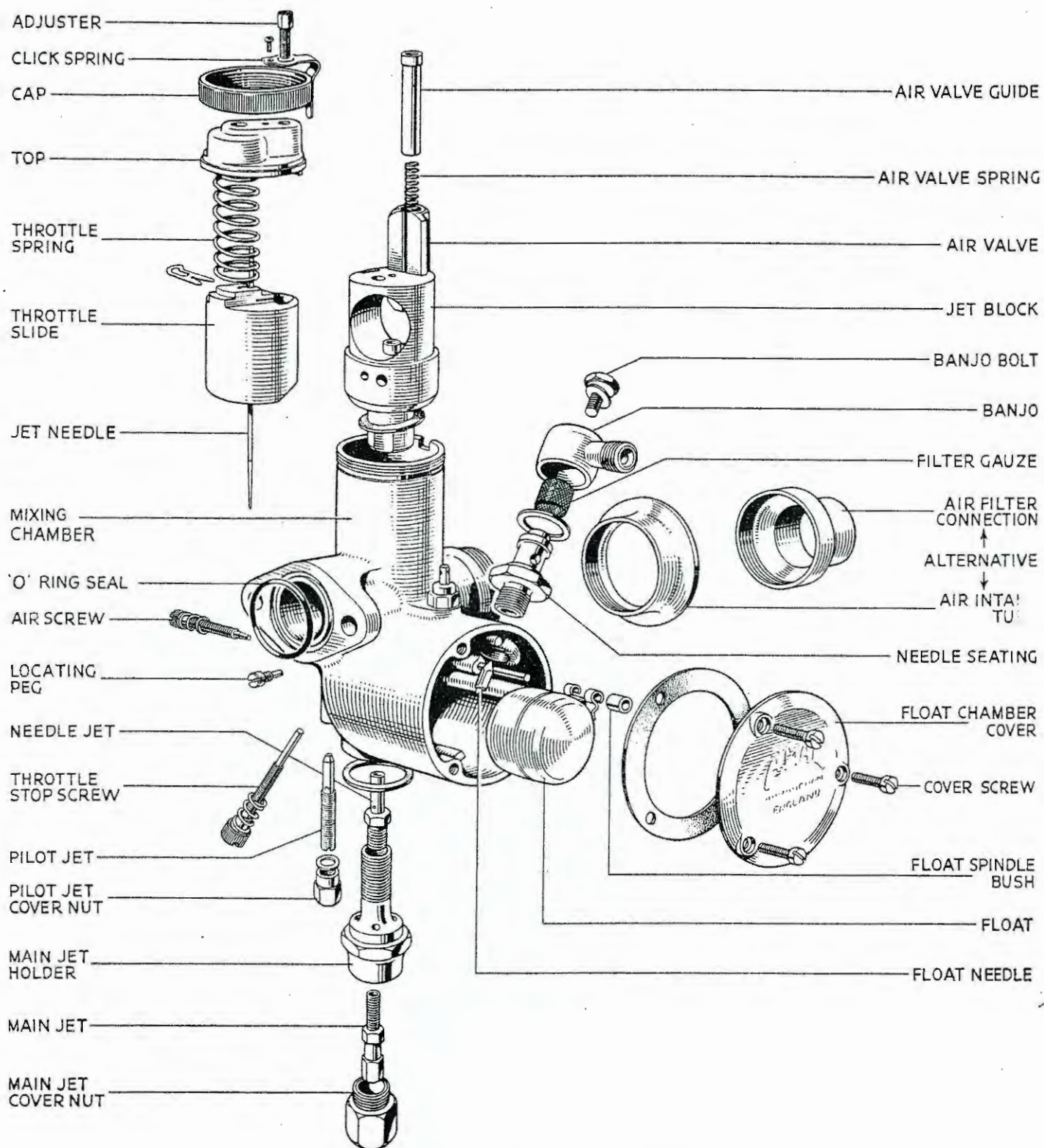
FIG. 29. AMAL CARBURETTER
