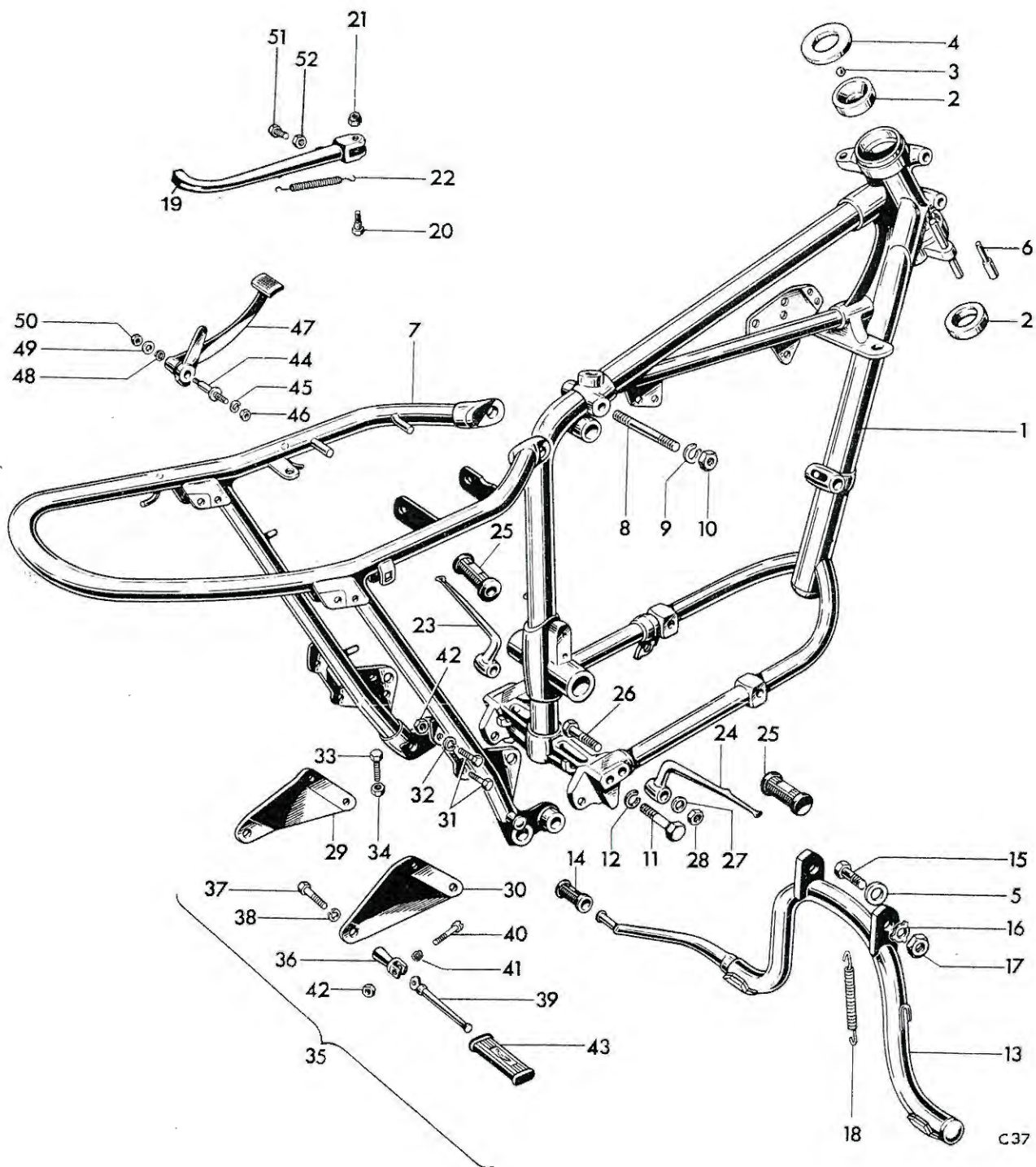
Fig. 15. FRAME
