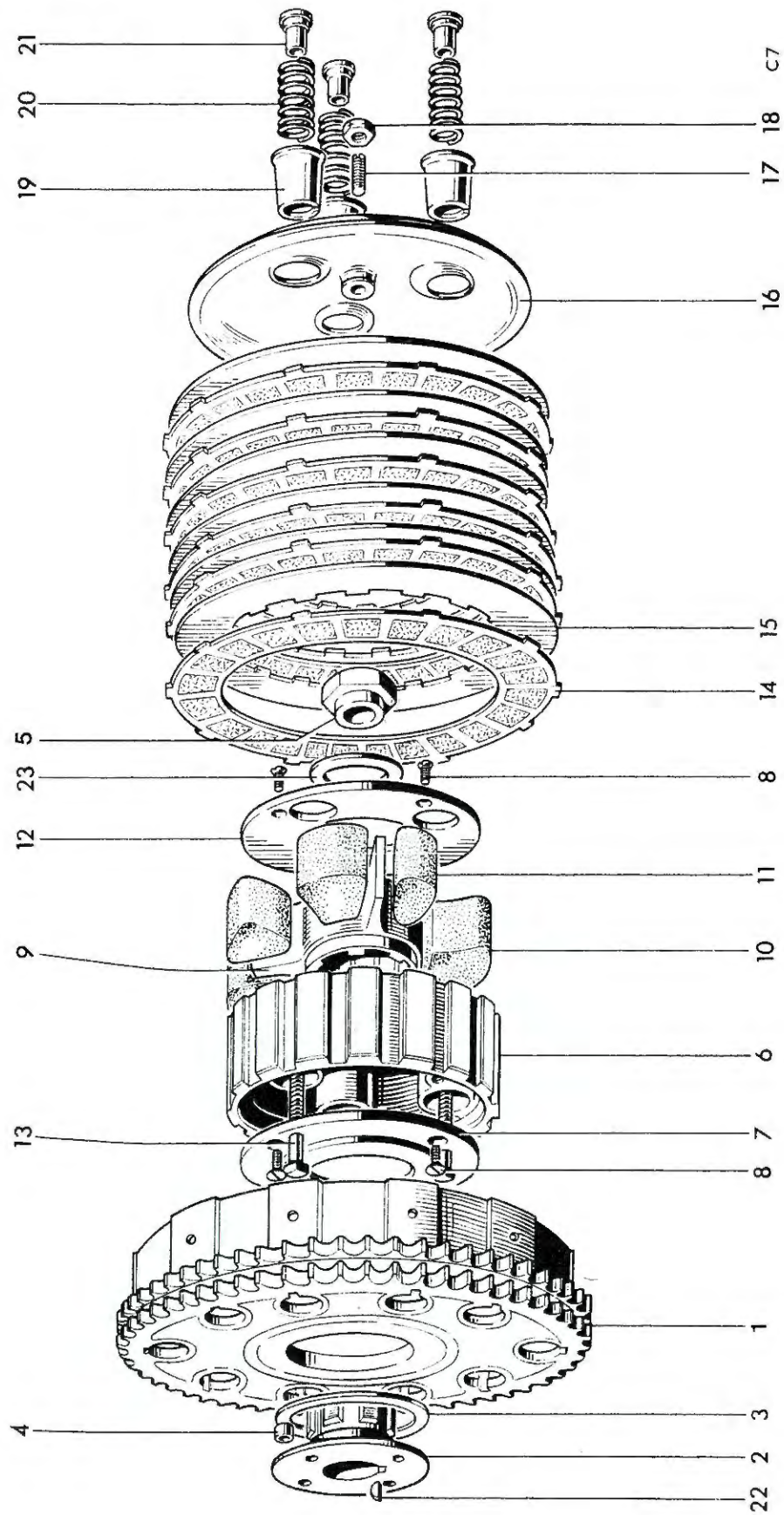
Fig. 11. CLUTCH
