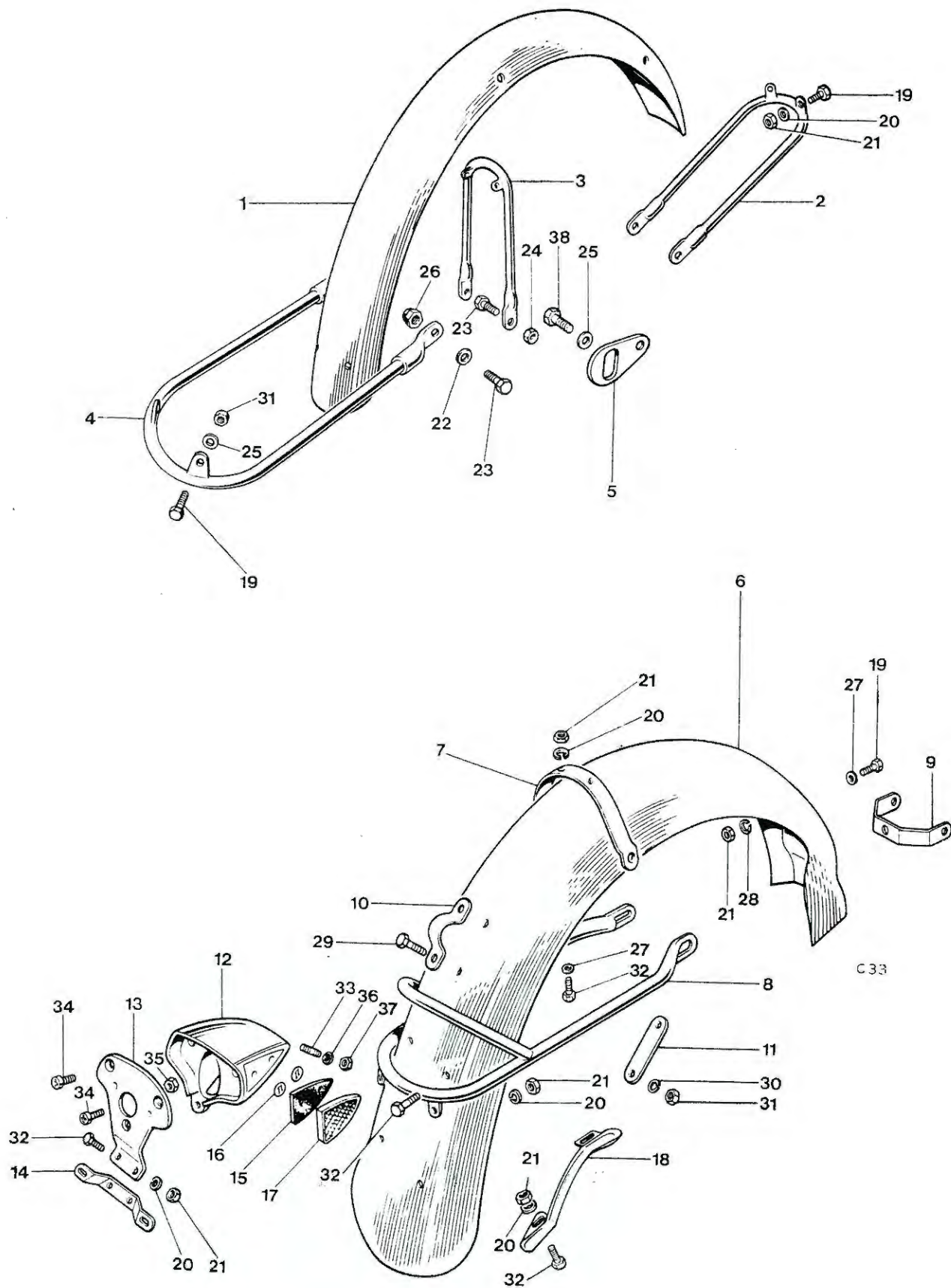
Fig. 23. FENDERS
